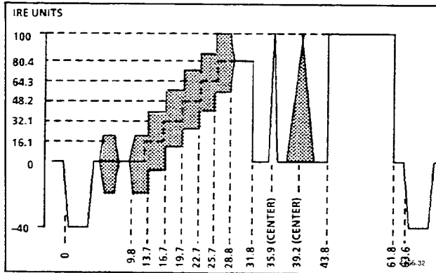
Fig. 6-7. FCC Composite.
