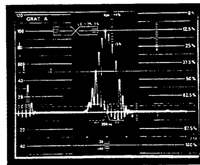
Figure 4 (d) 4.2 MHz
