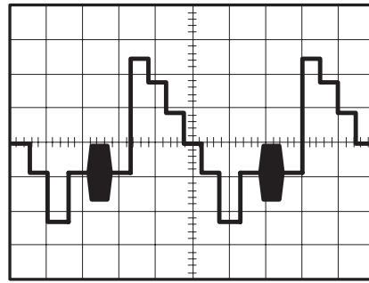
ラインにトリガした例
