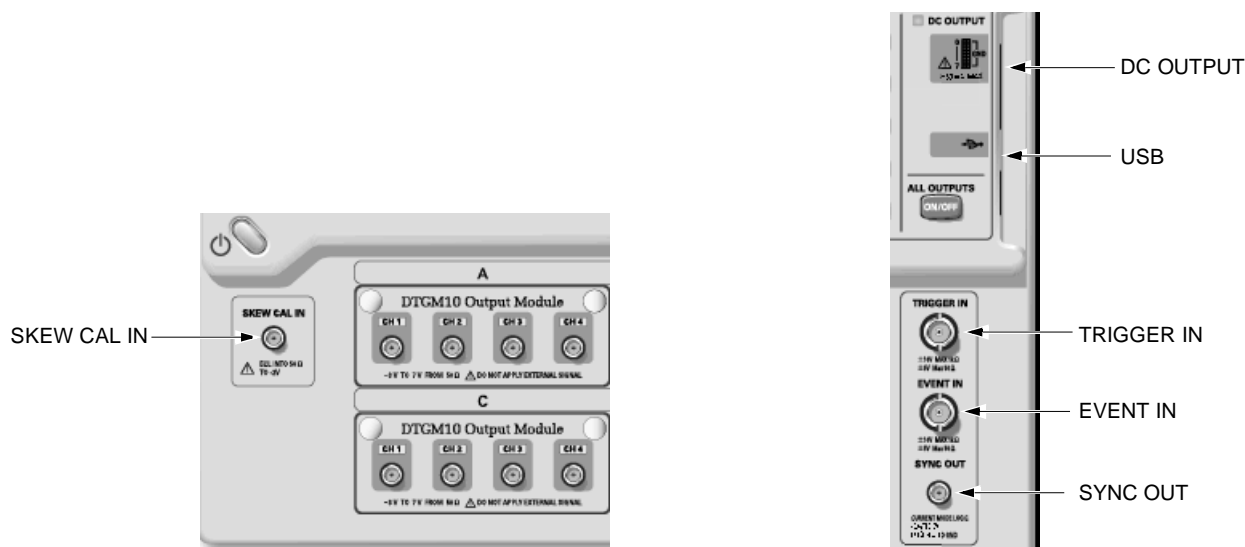
図 2-3. フロントパネル・コネクタ
