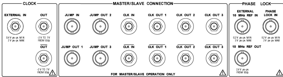
図 2-6. リアパネル・コネクタ ( 2 )
