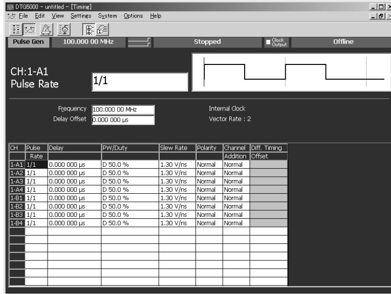
図 4-11. Pulse Gen モードの Timing ウィンドウ
