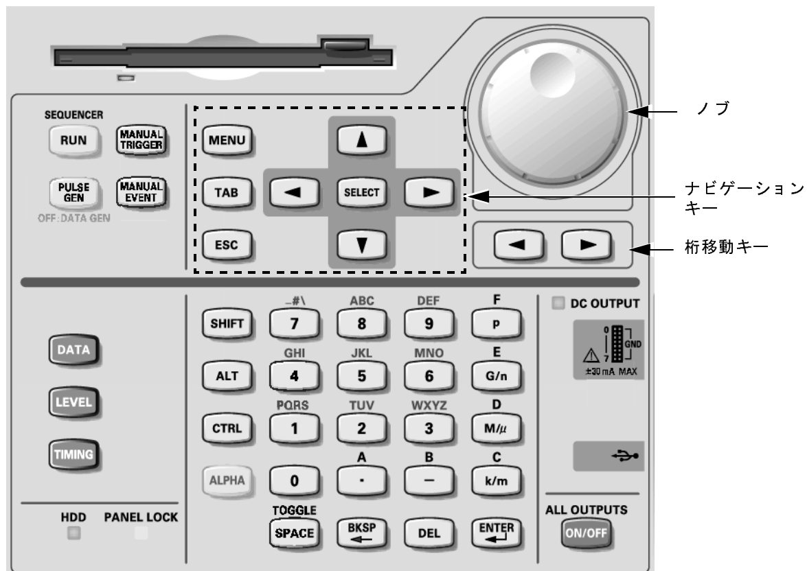
図 2-2. フロントパネル・コントロール
