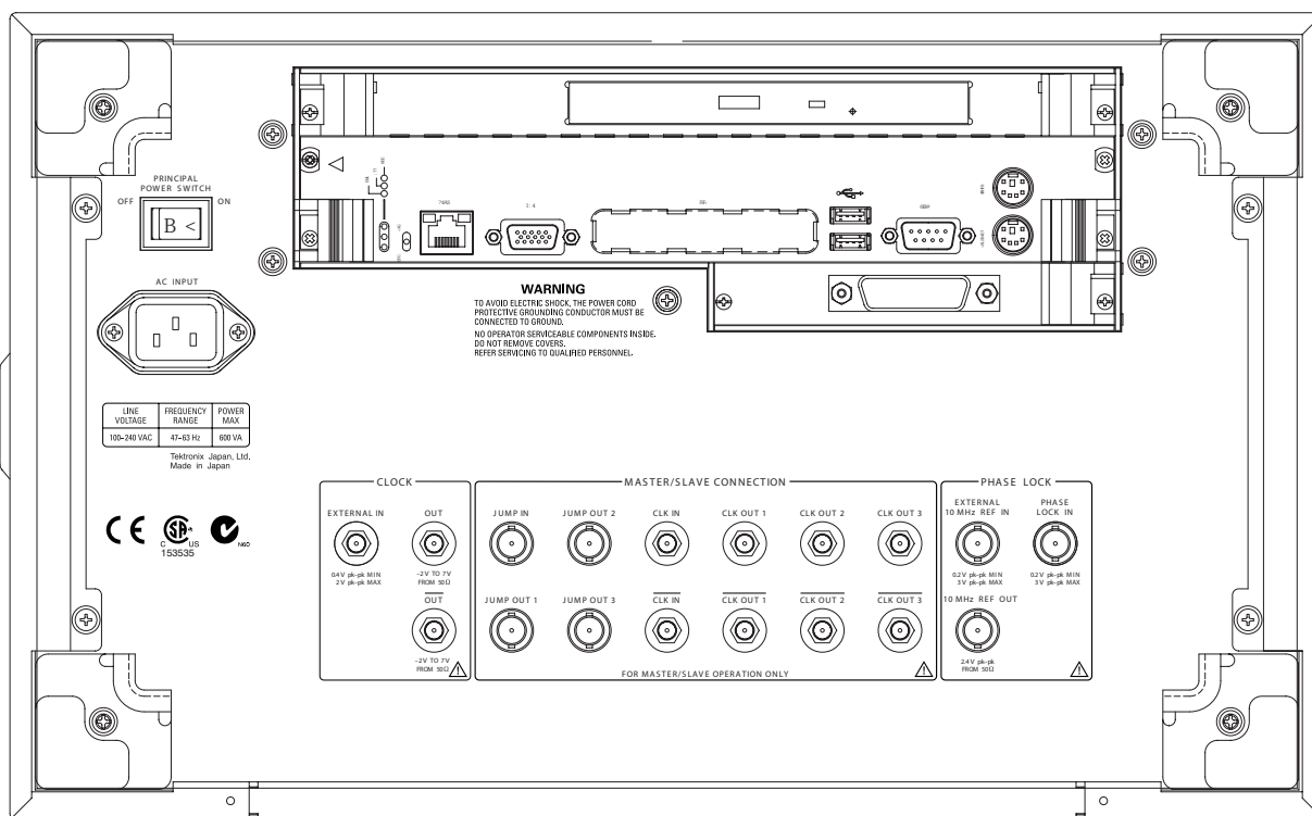
図 2-4. DTG5078 型リアパネル
