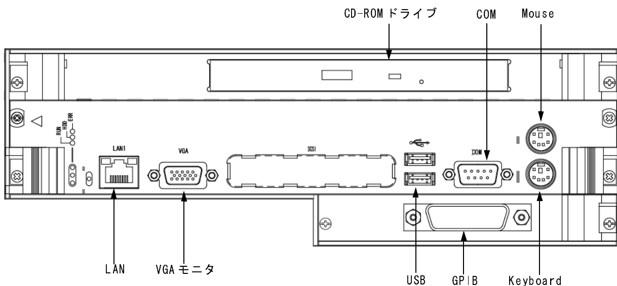
図 2-5. リアパネル・コネクタ (1)
