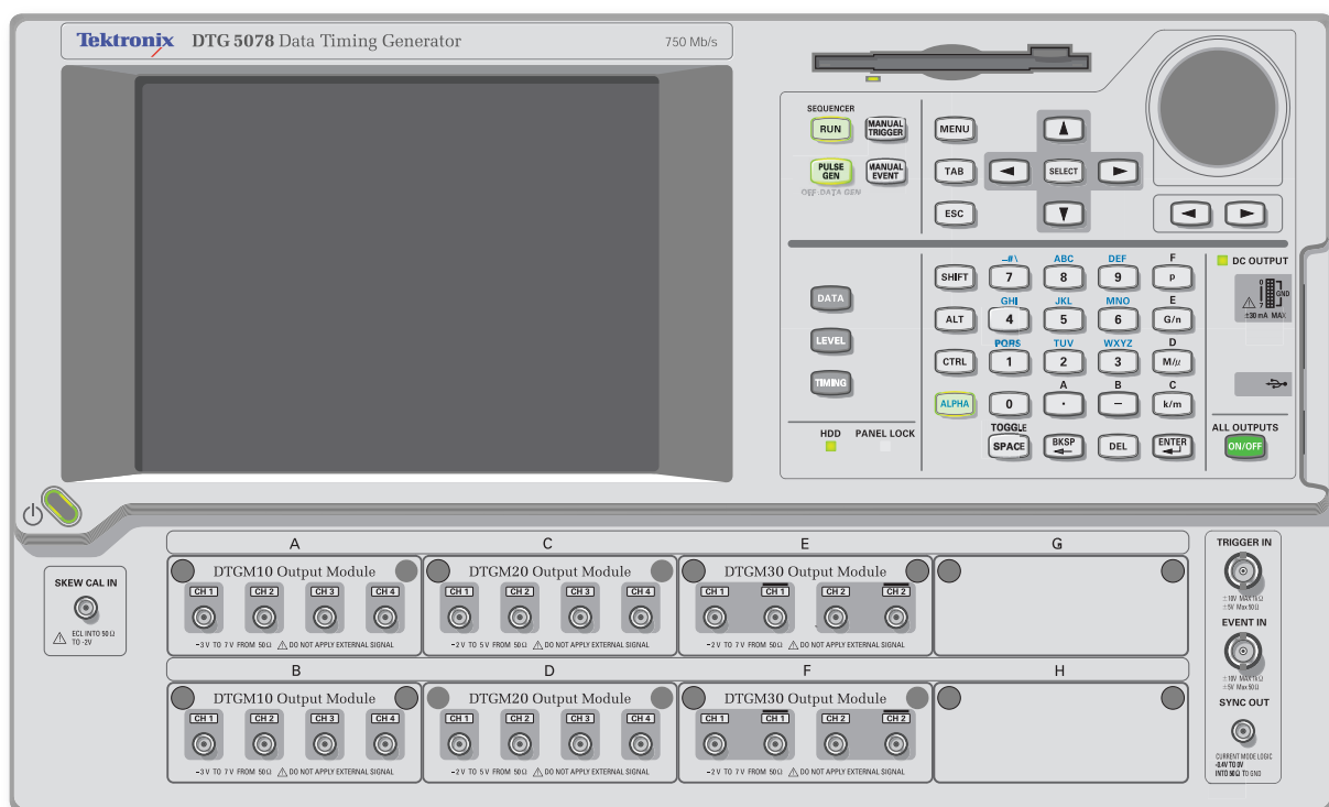
図 2-1. DTG5078 型フロントパネル
