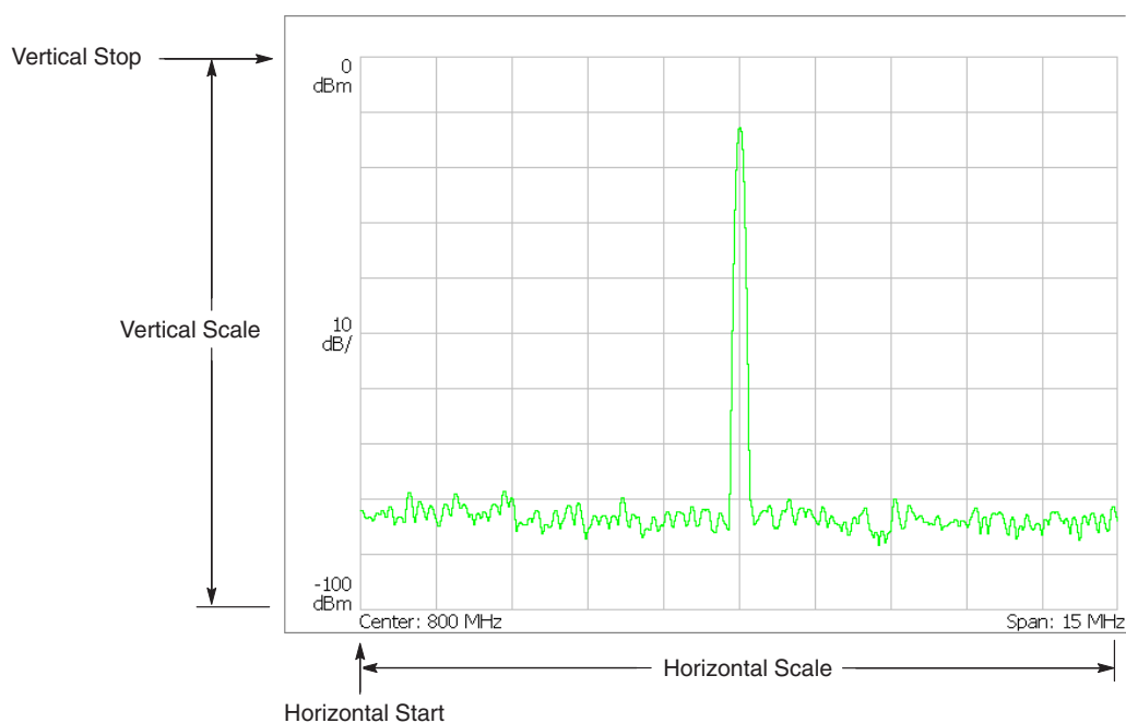
図 4-131 : スペクトラム表示のスケール設定
