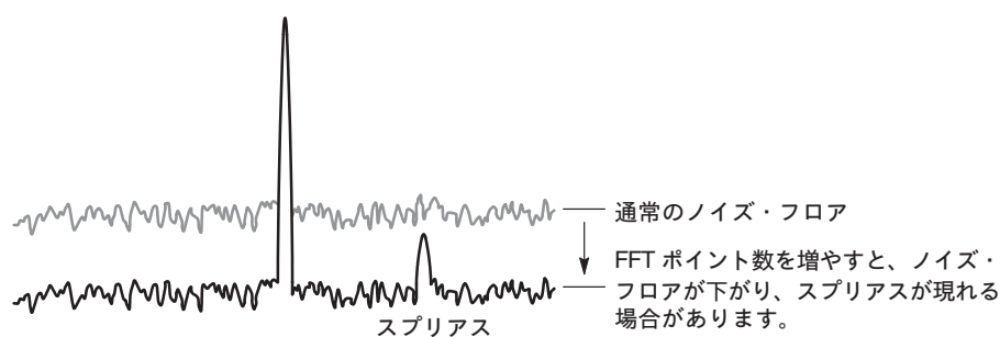
図 4-123 : FFT ポイント数の増加によるスプリアスの発生
