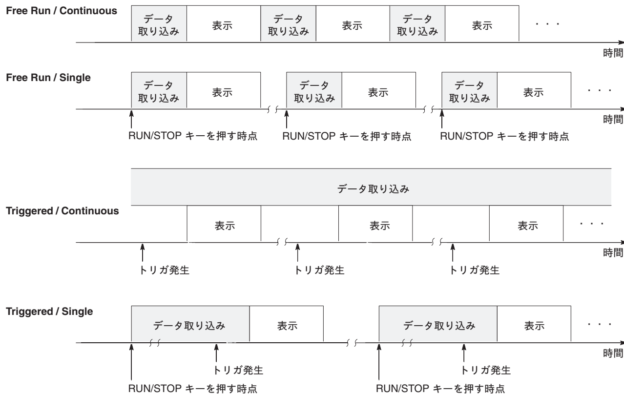
図 4-106：トリガおよびリピート・モードによるデータ取り込みと表示
