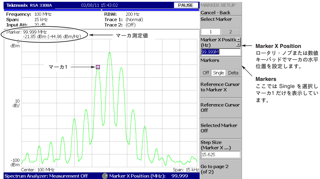
図 4-153 : メイン・マーカを使用した測定
