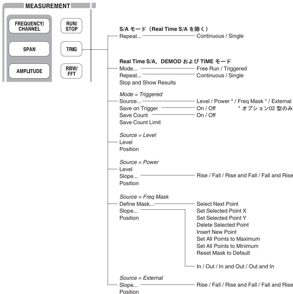
図 4-103 : TRIG メニュー
