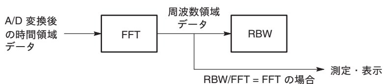
図 4-121：RBW/FFT = FFT のときの処理の流れ
