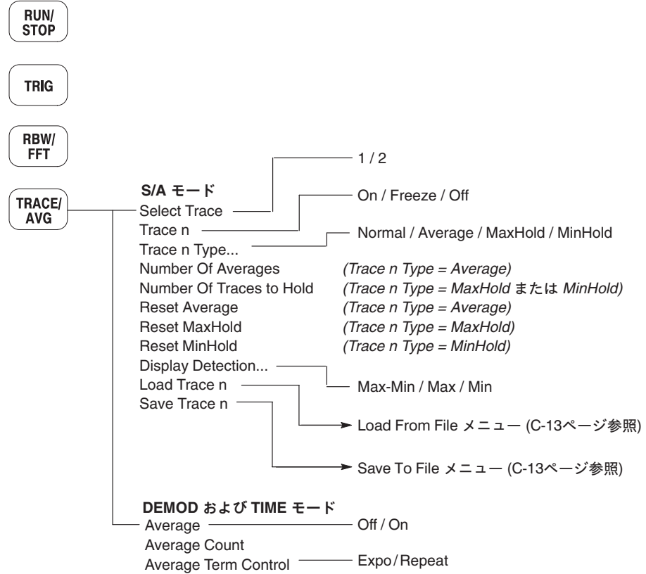
図 4-126 : TRACE/AVG メニュー
