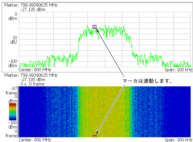
図 4-157 : マーカの連動
