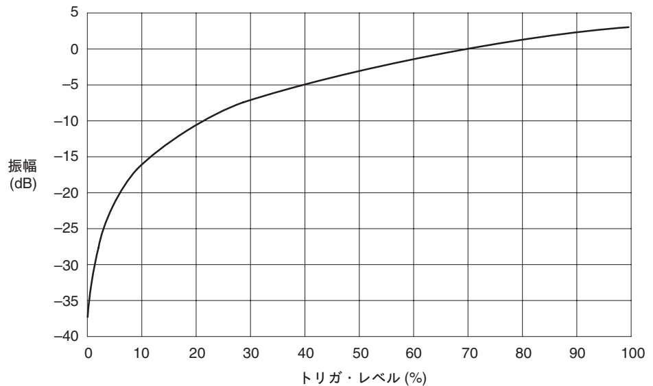
図 4-107 : トリガ・レベル vs. 振幅 (リファレンス・レベル = +3dBm)
