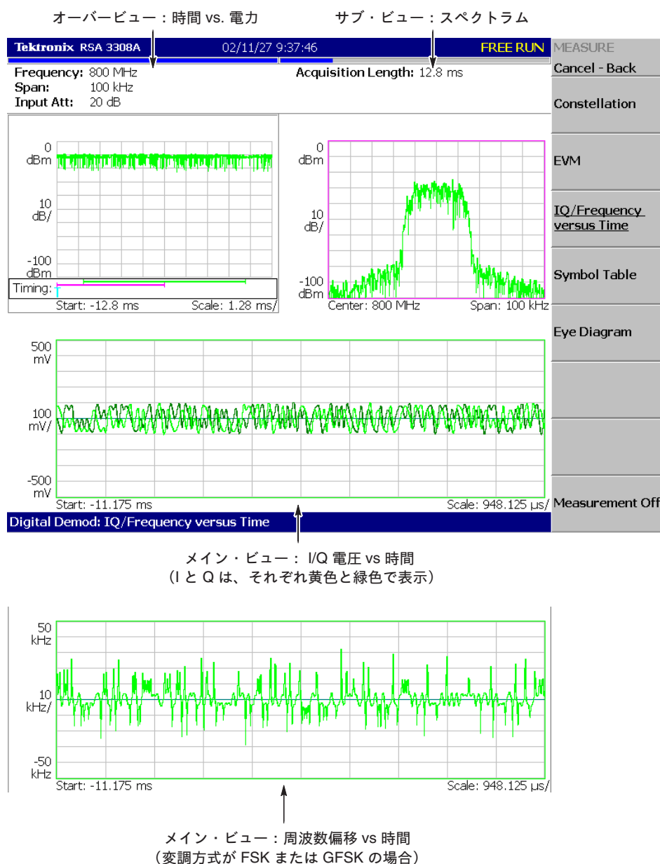
図 4-42 : IQ レベル／周波数変動測定例
