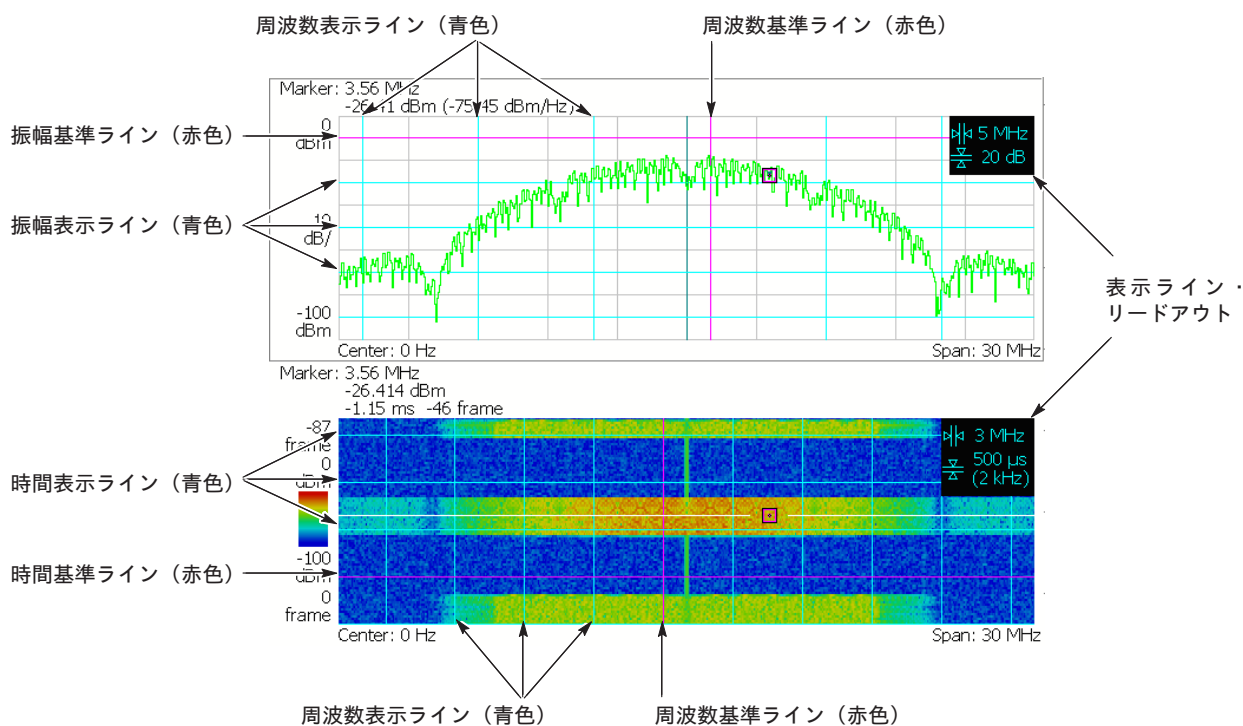
図 4-149 : マルチ表示ライン (Real Time S/A モード)
