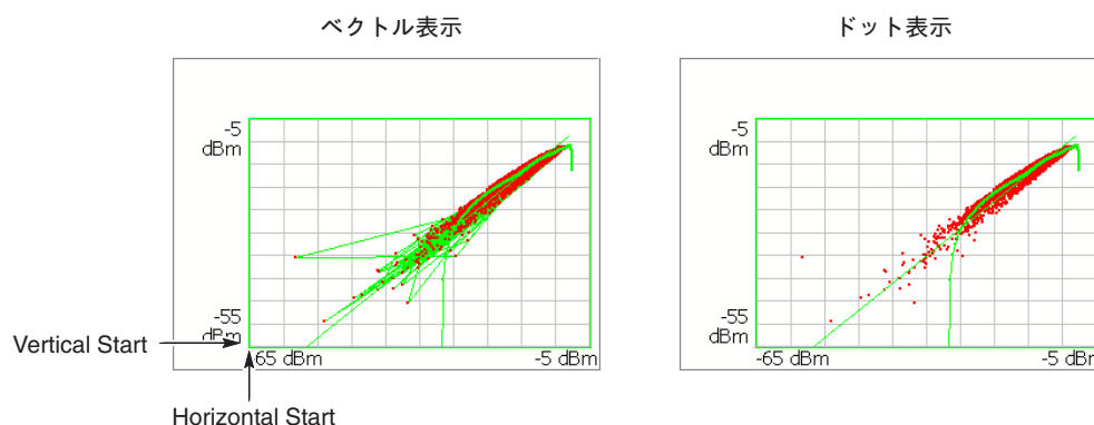
図 4-141 : AM/AM ビューのスケール設定
