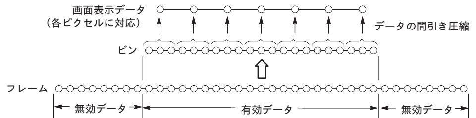
図 4-129 : フレーム、ビン、ピクセルの関係
