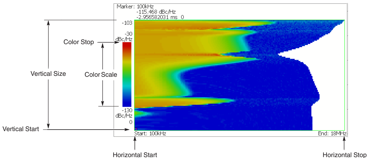
図 4-144 : ノイズグラム表示のスケールの設定
