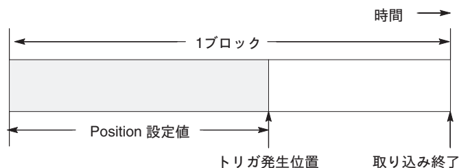
図 4-105：トリガ・ポジション
