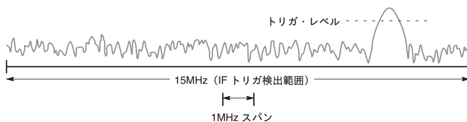
図 4-109 : IF トリガ検出範囲
