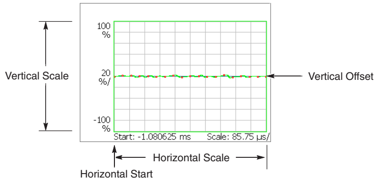
図 4-136 : EVM 表示のスケール設定
