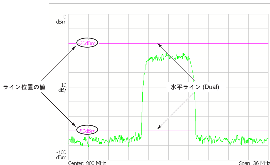
図 4-147 : 水平ライン
