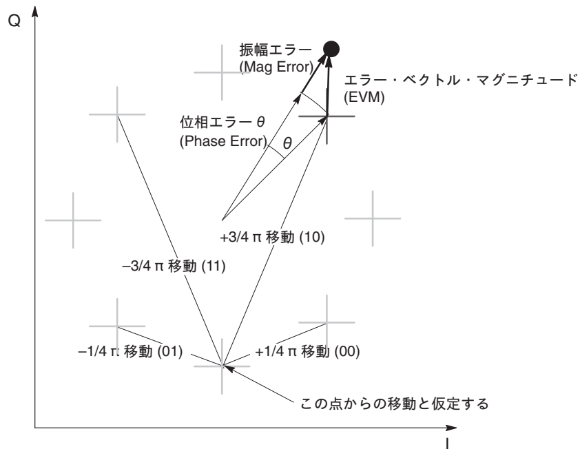
図 4-138 : 1/4\pi QPSK のコンスタレーション表示例と誤差ベクトル
