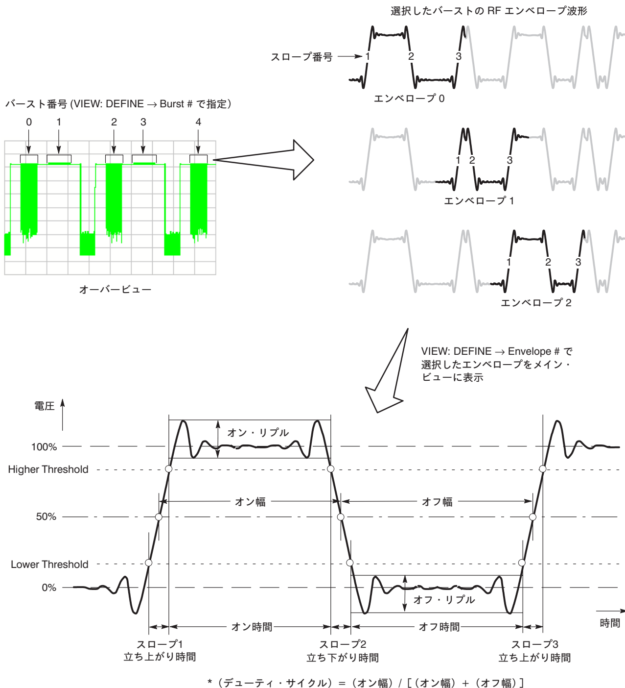
図 4-59 : RF エンベロープ測定パラメータ
