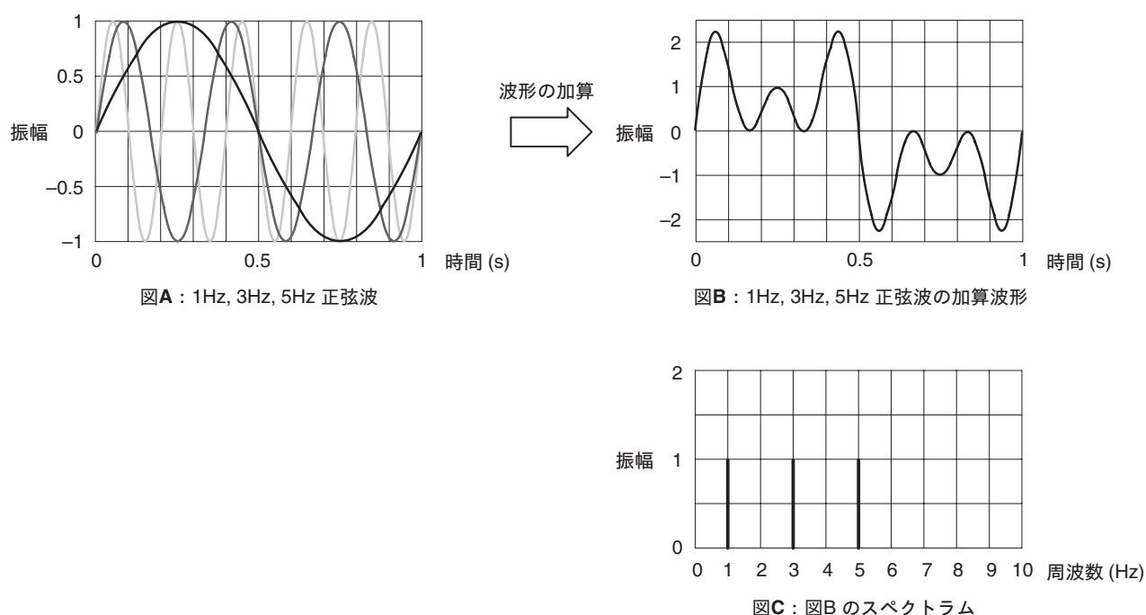
図 4-108 : 時間領域の波形と周波数領域の波形
