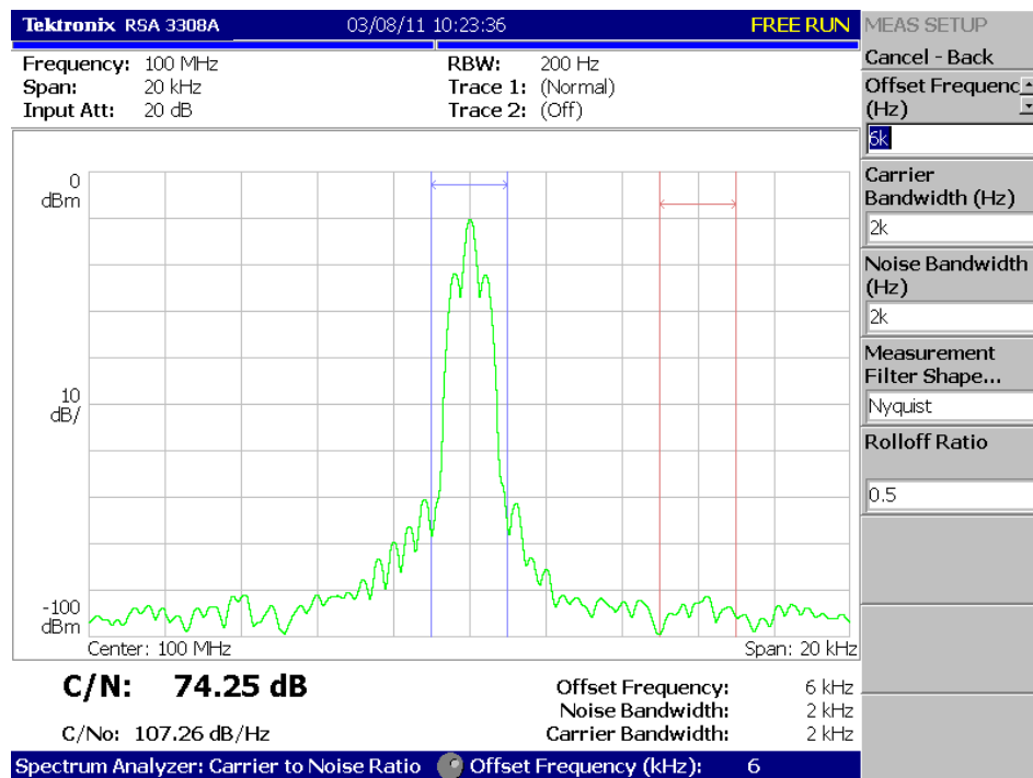
図 4-9 : C/N 測定例
