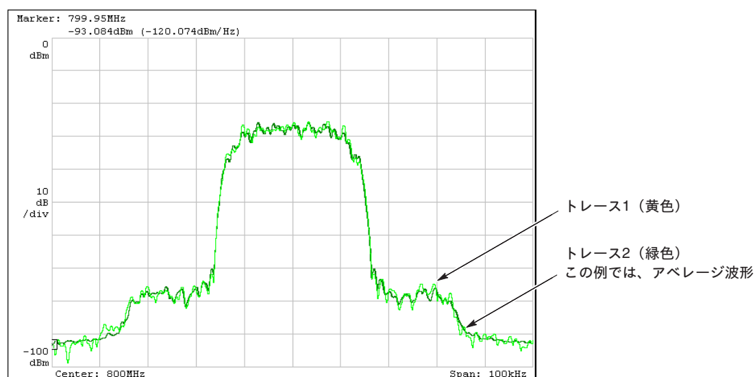
図 4-125 : トレース1 と 2 の比較表示例
