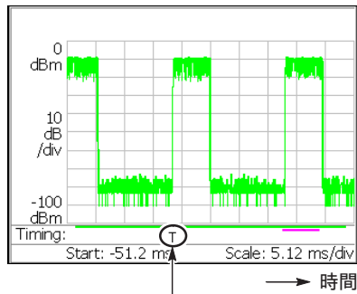
図 4-117：トリガ点の表示
