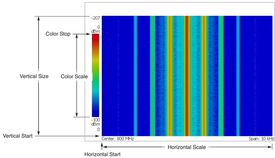
図 4-132 : スペクトログラム表示のスケールとフォーマットの設定
