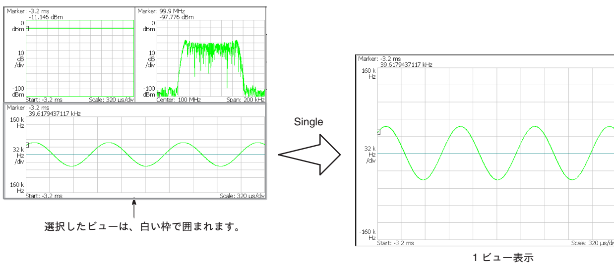
図 4-33 : 1 ビュー表示
