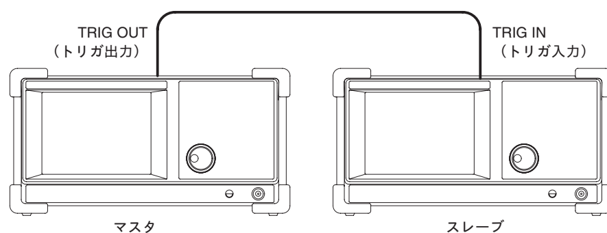
図 4-118 : 副数台の同期運転
