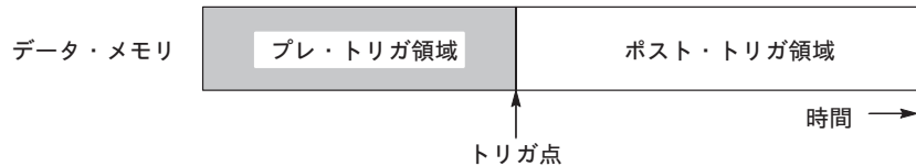
図 3-5 : プレおよびポスト・トリガ領域
