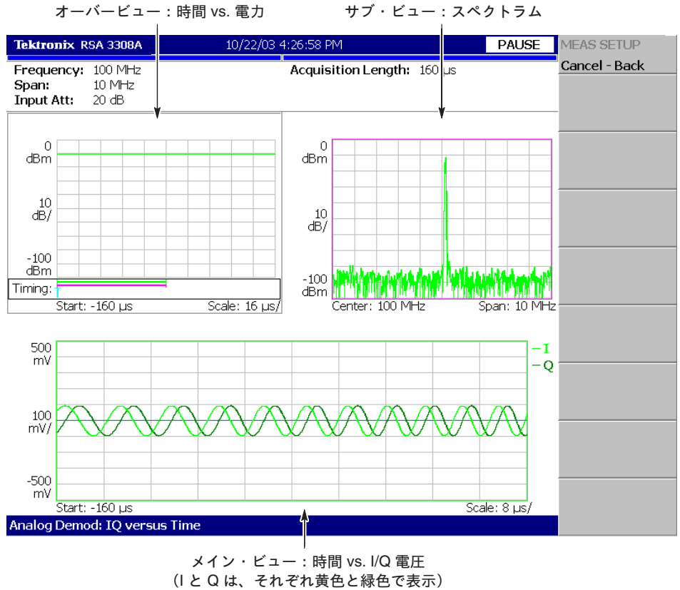
図 4-37 : IQ レベル変動測定例
