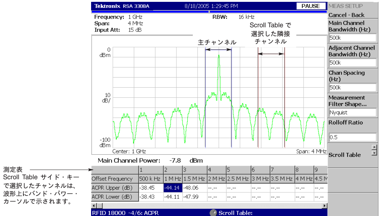
図 4-54 : ACPR 測定
