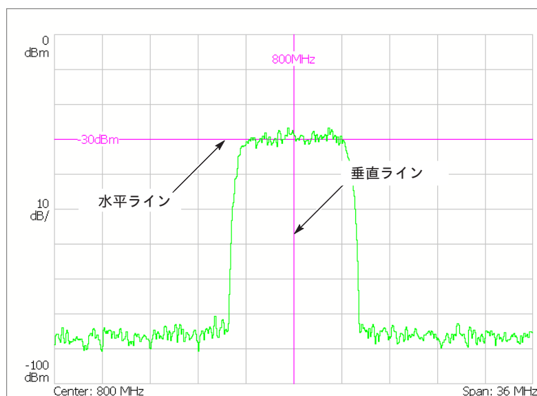
図 4-145 : 表示ライン
