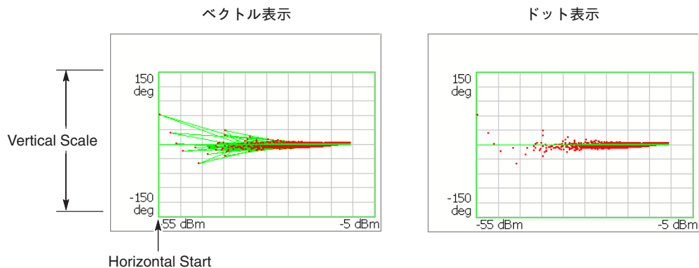
図 4-142 : AM/PM ビューのスケール設定
