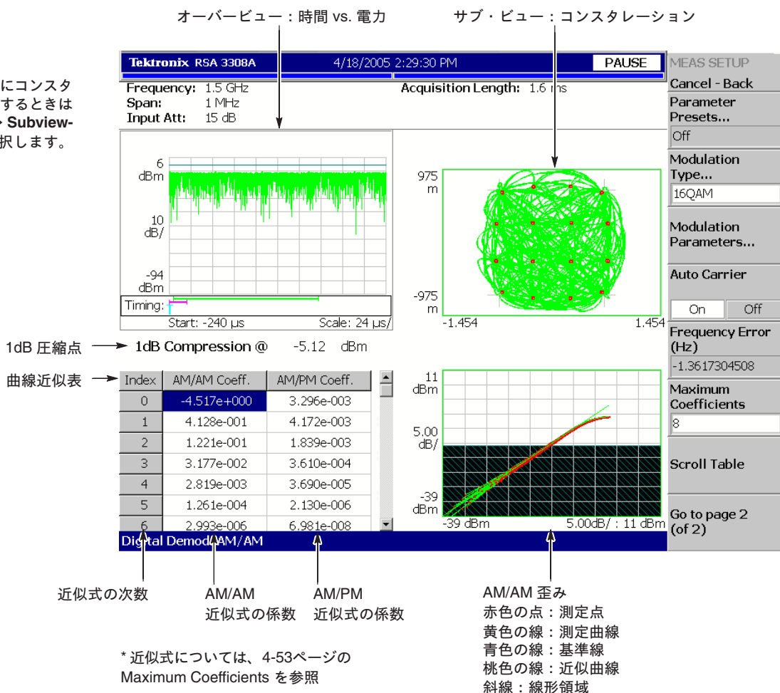
図 4-46 : AM/AM 歪み解析例
