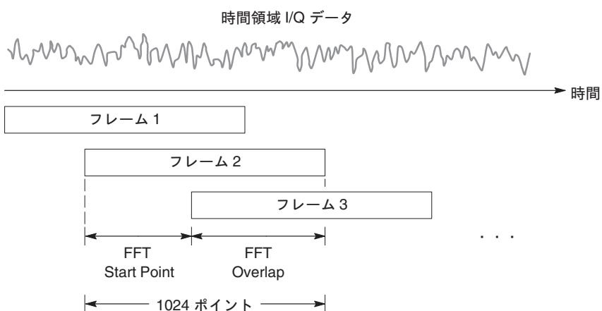
図 4-122 : FFT オーバーラップ
