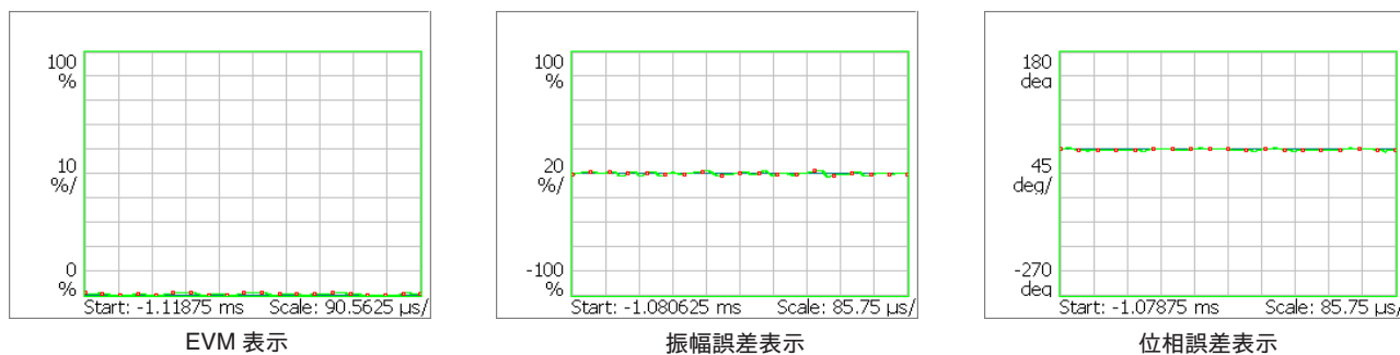
図 4-137 : EVM、振幅および位相誤差表示
