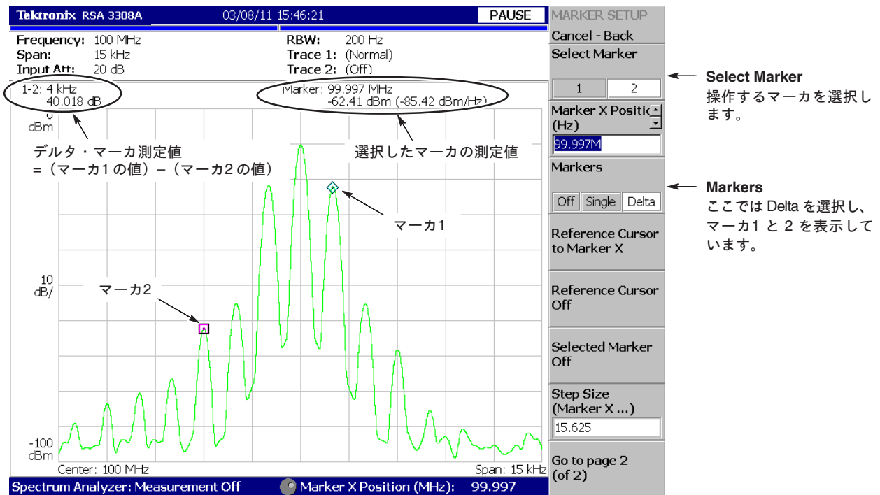
図 4-154 : デルタ・マーカを使用した測定
