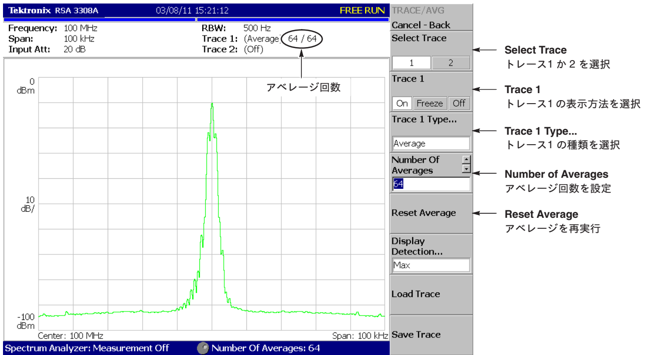
図 4-127 : アベレージ表示例
