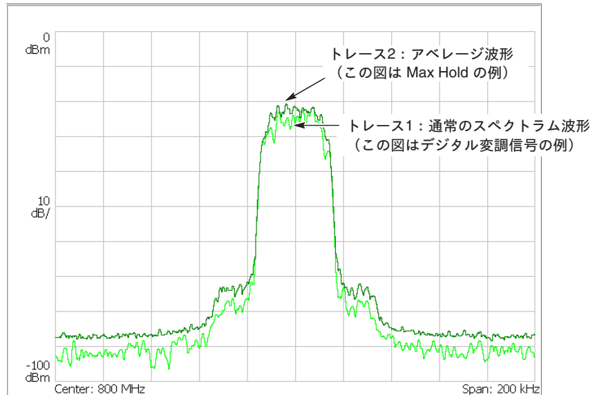
図 4-128 : 比較表示例
