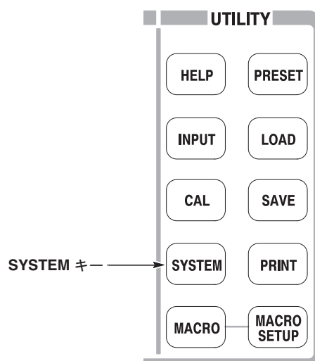
図 2-5 : SYSTEM キー
