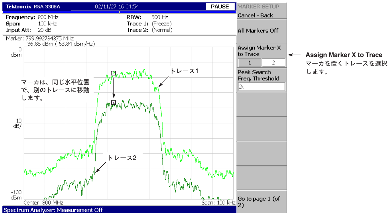
図 4-156 : マーカを置くトレースの切り替え
