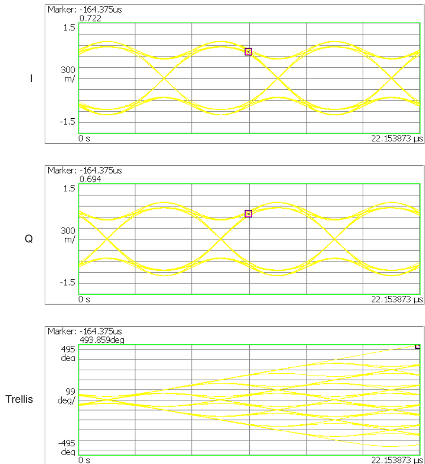
図 4-140 : アイ・ダイアグラム表示例
