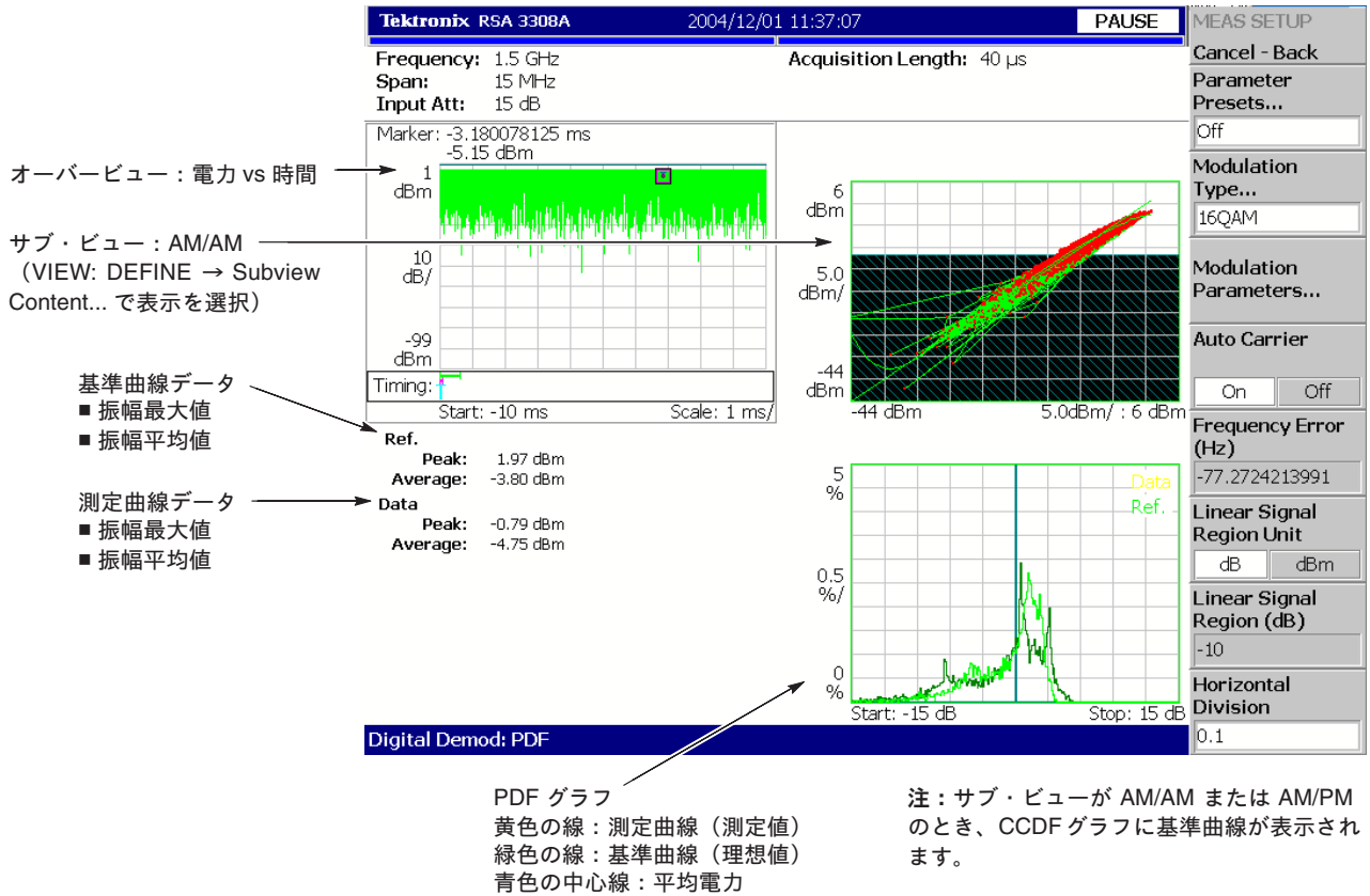
図 4-50 : PDF 解析例
