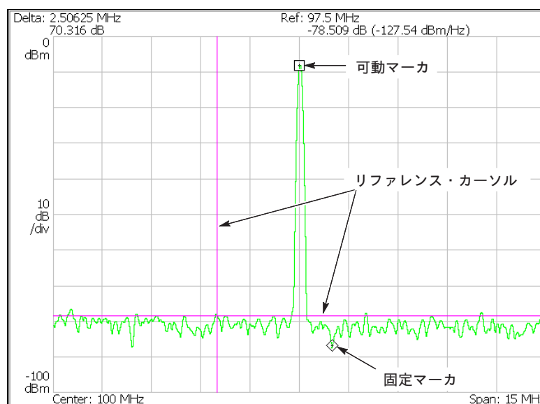
図 4-151 : マーカ表示
