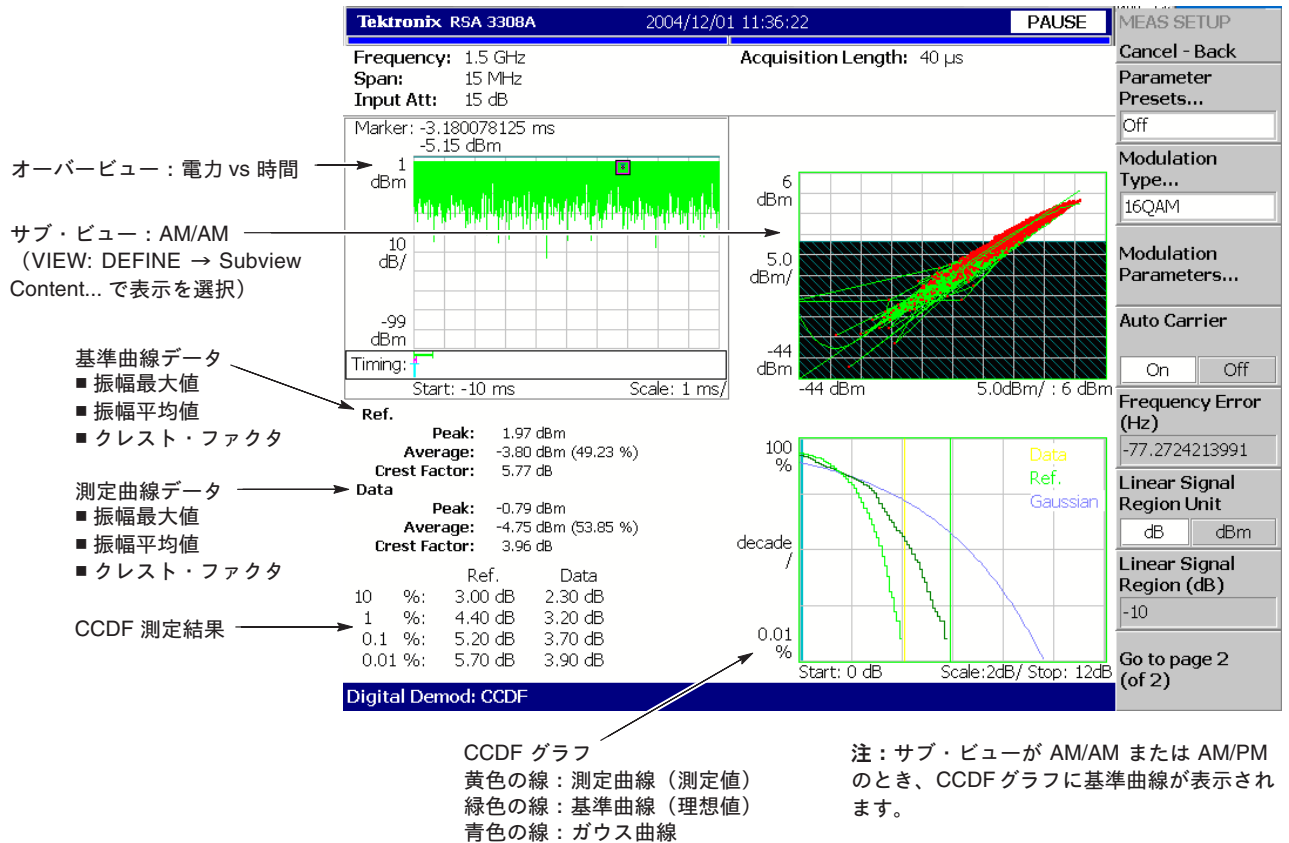
図 4-49 : CCDF 測定例
