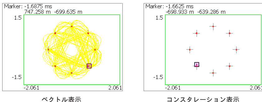
図 4-135 : ベクトル表示とコンスタレーション表示
