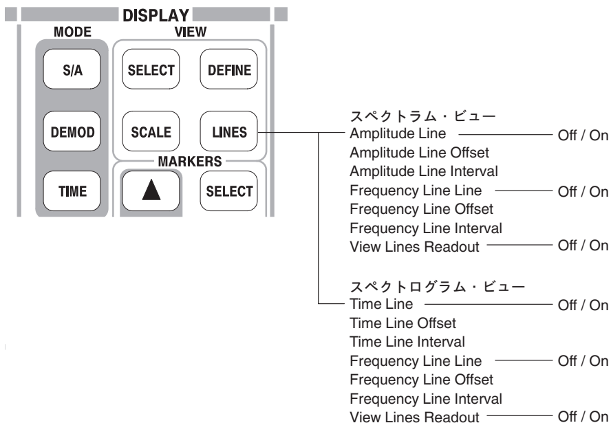
図 4-150 : LINES メニュー (Real Time S/A モード)
