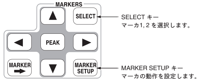
図 4-152 : MARKERS キー
