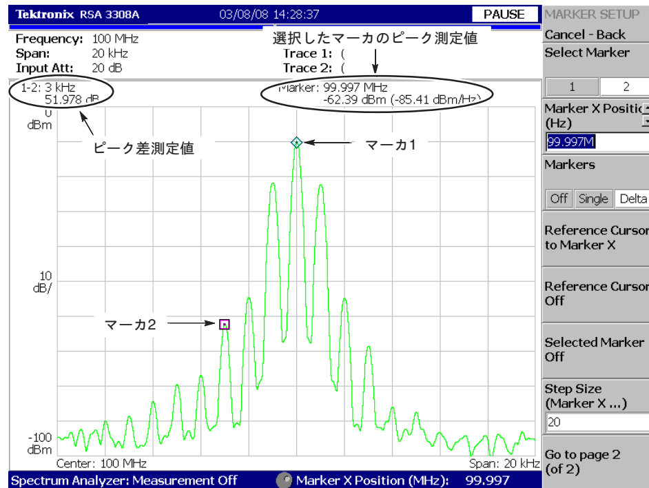
図 2-23 : ピーク検出
