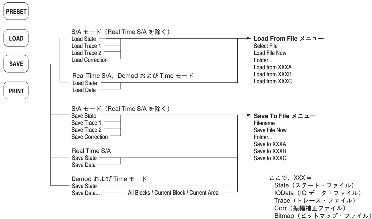
図 4-166 : LOAD/SAVE メニュー
