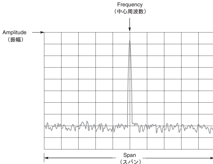
図 2-6 : 周波数、スパン、振幅の設定
