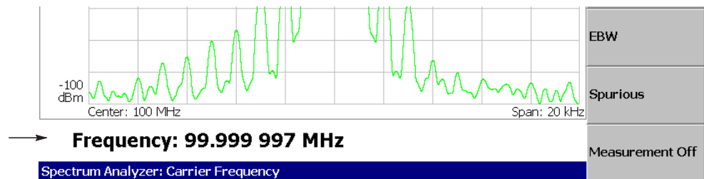
図 2-36 : キャリア周波数測定例（画面下部）
