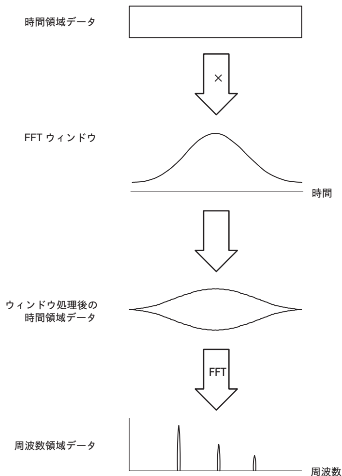
図 4-124 : 時間領域データのウィンドウ処理
