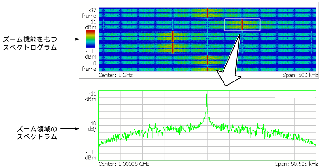
図 4-21 : ズーム機能
