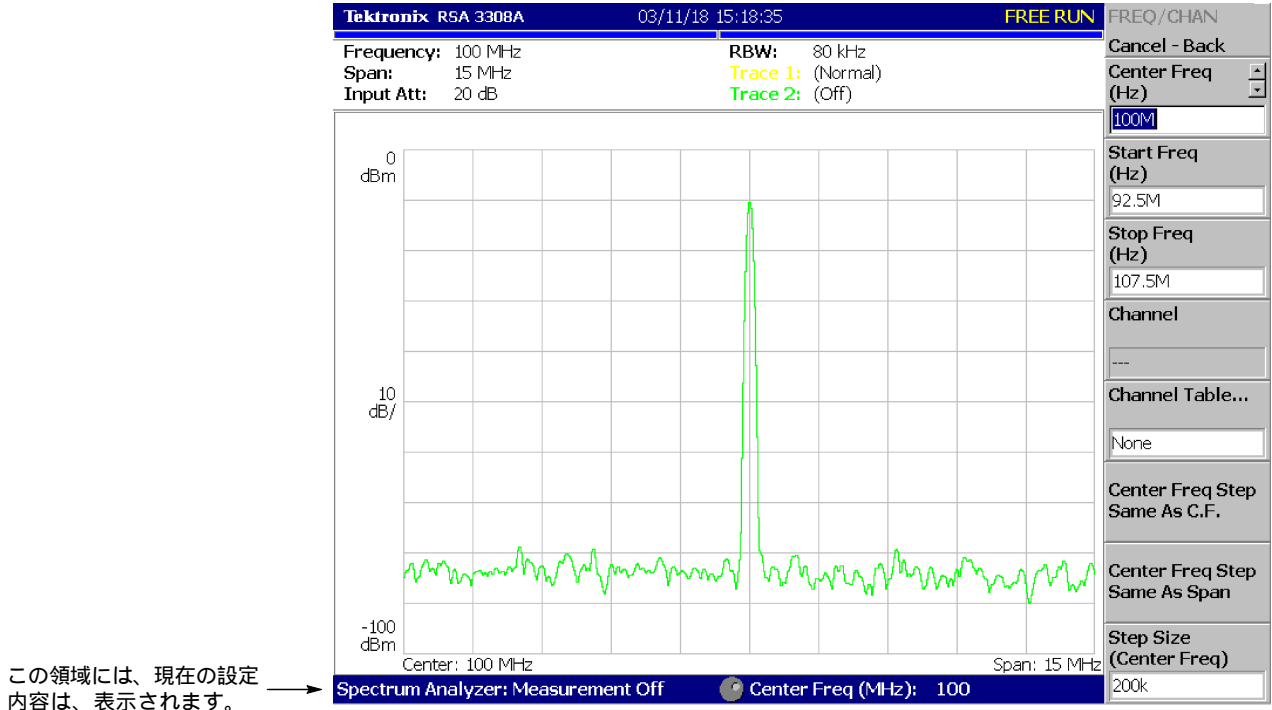
図 2-10 : 中心周波数 100MHz、スパン 15MHz
