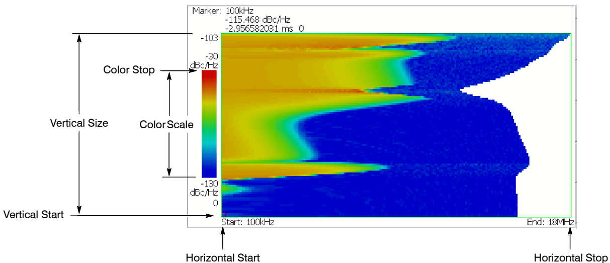
図 4-149 : ノイズグラム表示のスケールの設定
