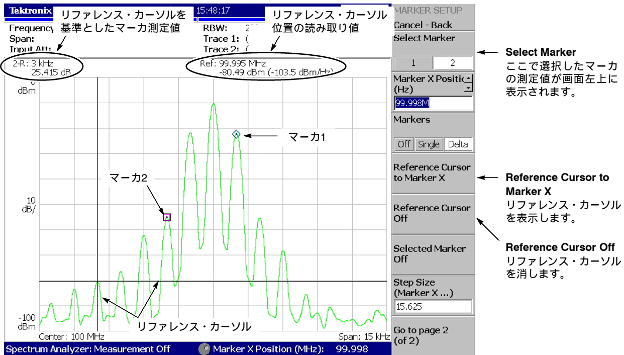
図 4-160 : リファレンス・カーソルを使用した測定
