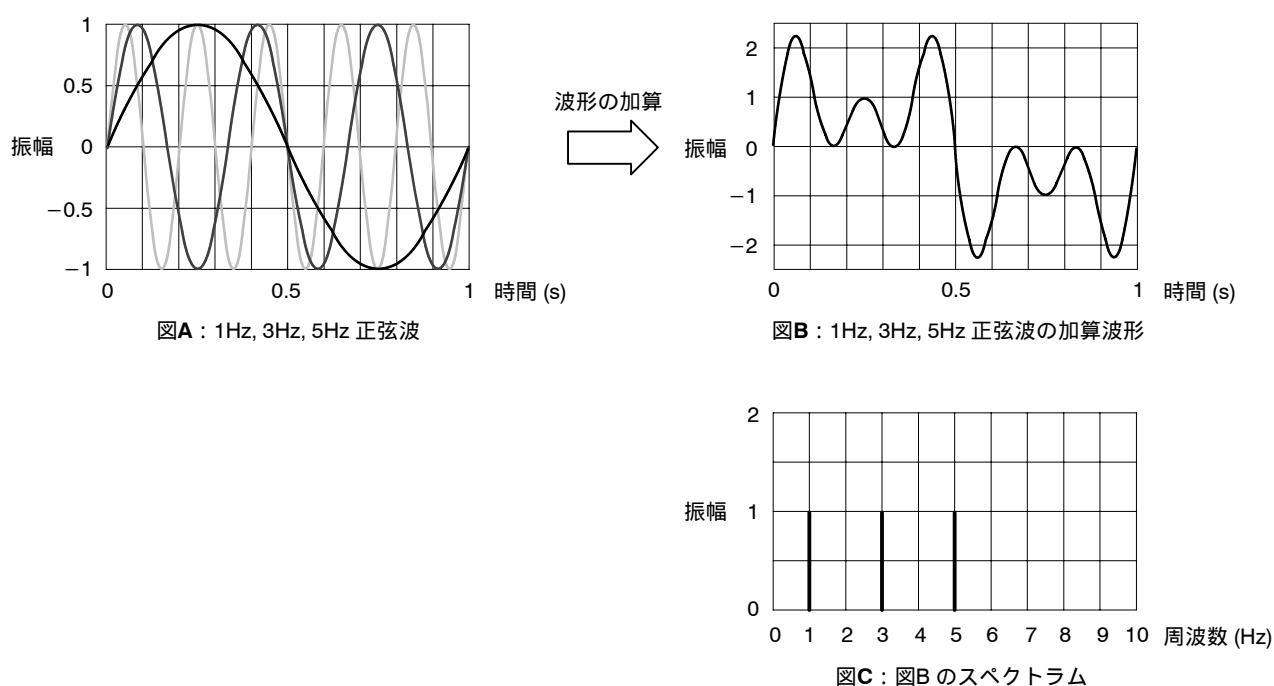
図 4-113 : 時間領域の波形と周波数領域の波形
