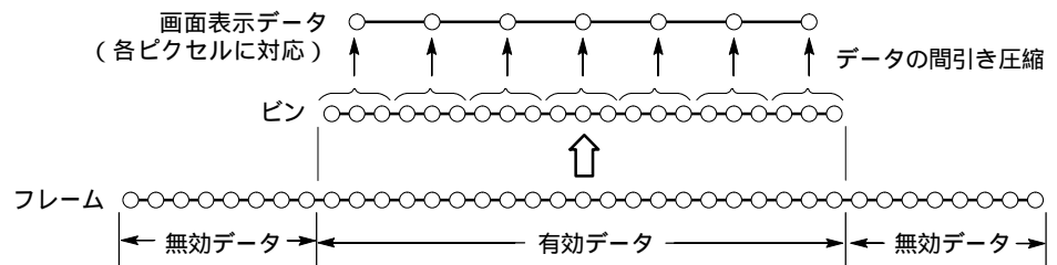
図 4-134 : フレーム、ピン、ピクセルの関係
