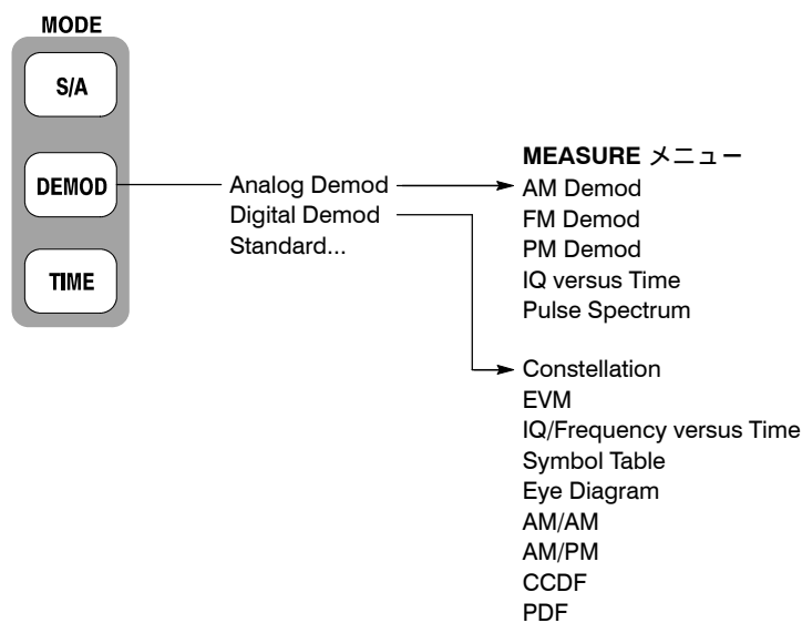
図 4-24 : DEMOD キー
