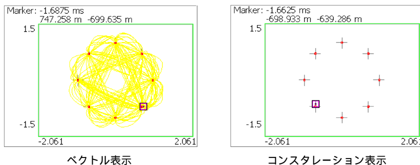
図 4-140 : ベクトル表示とコンスタレーション表示
