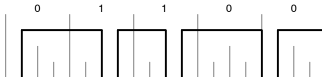
図 4-55 : Modified Miller 符号方式
