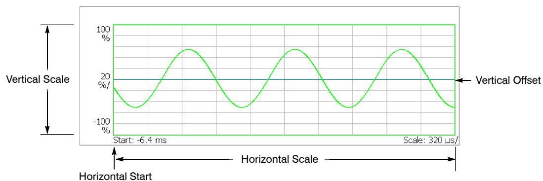
図 4-138：時間領域表示のスケール設定
