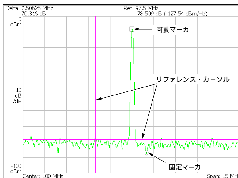
図 4-156 : マーカ表示
