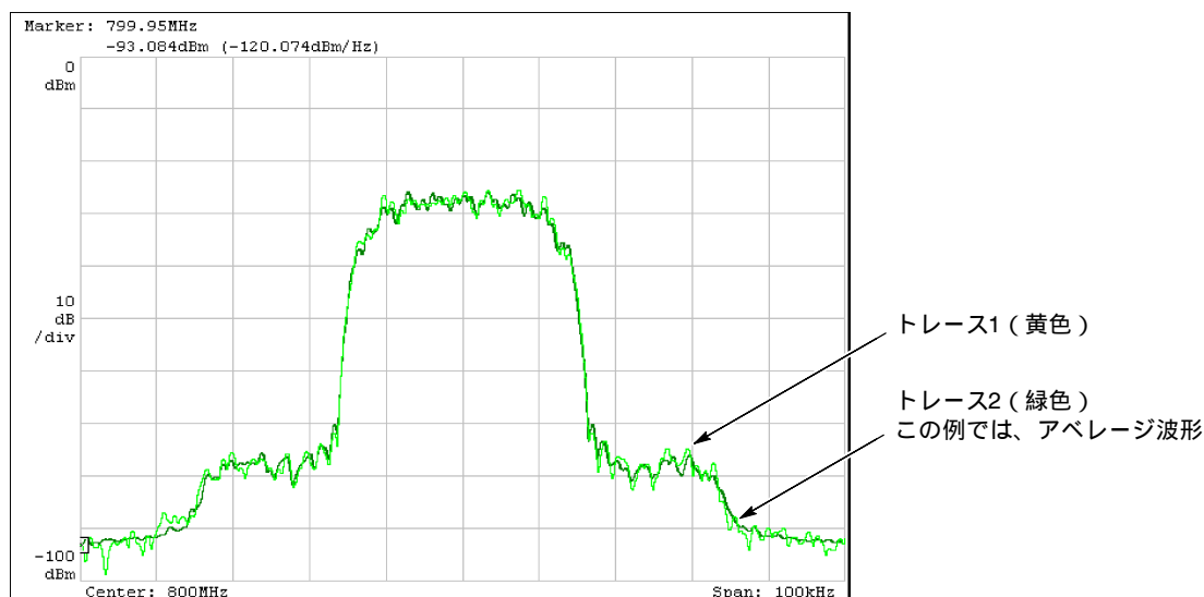
図 4-130 : トレース1 と 2 の比較表示例
