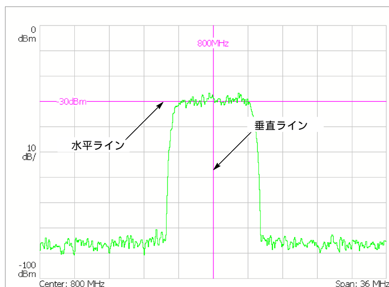
図 4-150：表示ライン
