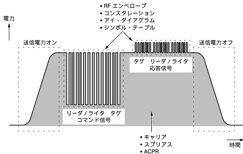
図 4-51 : RFID 波形と測定項目
