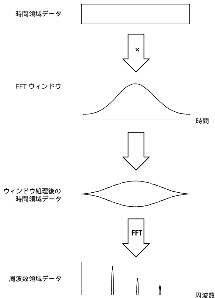
図 4-129：時間領域データのウィンドウ処理
