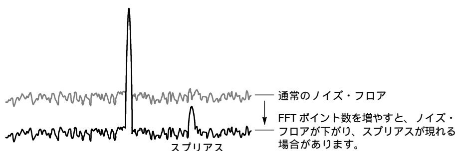
図 4-128 : FFT ポイント数の増加によるスプリアスの発生
