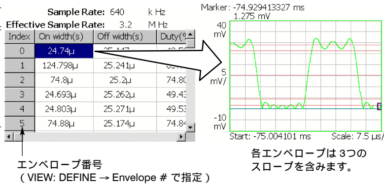
図 4-58 : RF エンベロープ測定 (メイン・ビュー)
