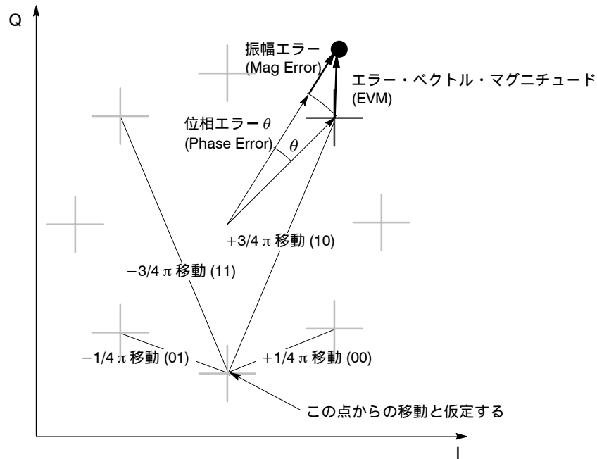
図 4-143 : 1/4 \pi QPSK のコンスタレーション表示例と誤差ベクトル
