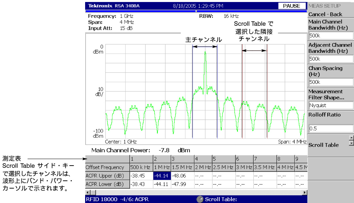
図 4-54 : ACPR 測定
