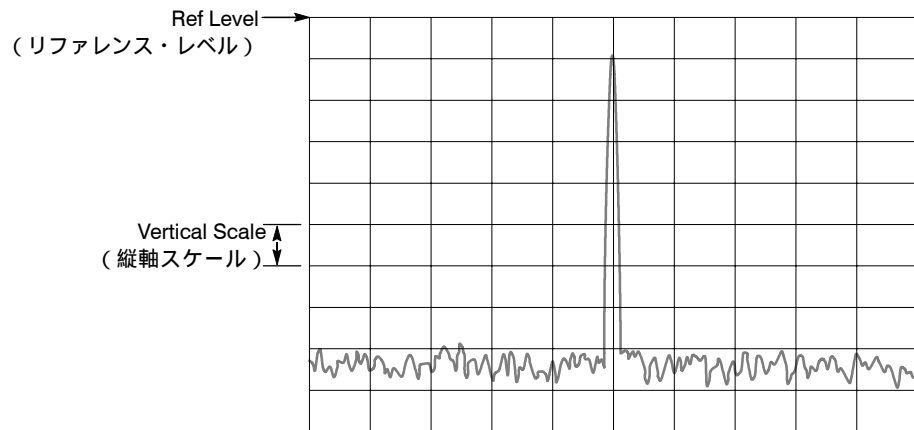
図 4-90：振幅の設定
