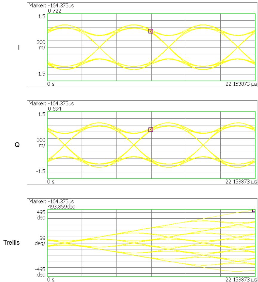
図 4-145 : アイ・ダイアグラム表示例
