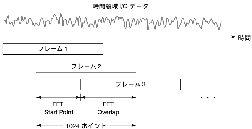
図 4-127 : FFT オーバーラップ
