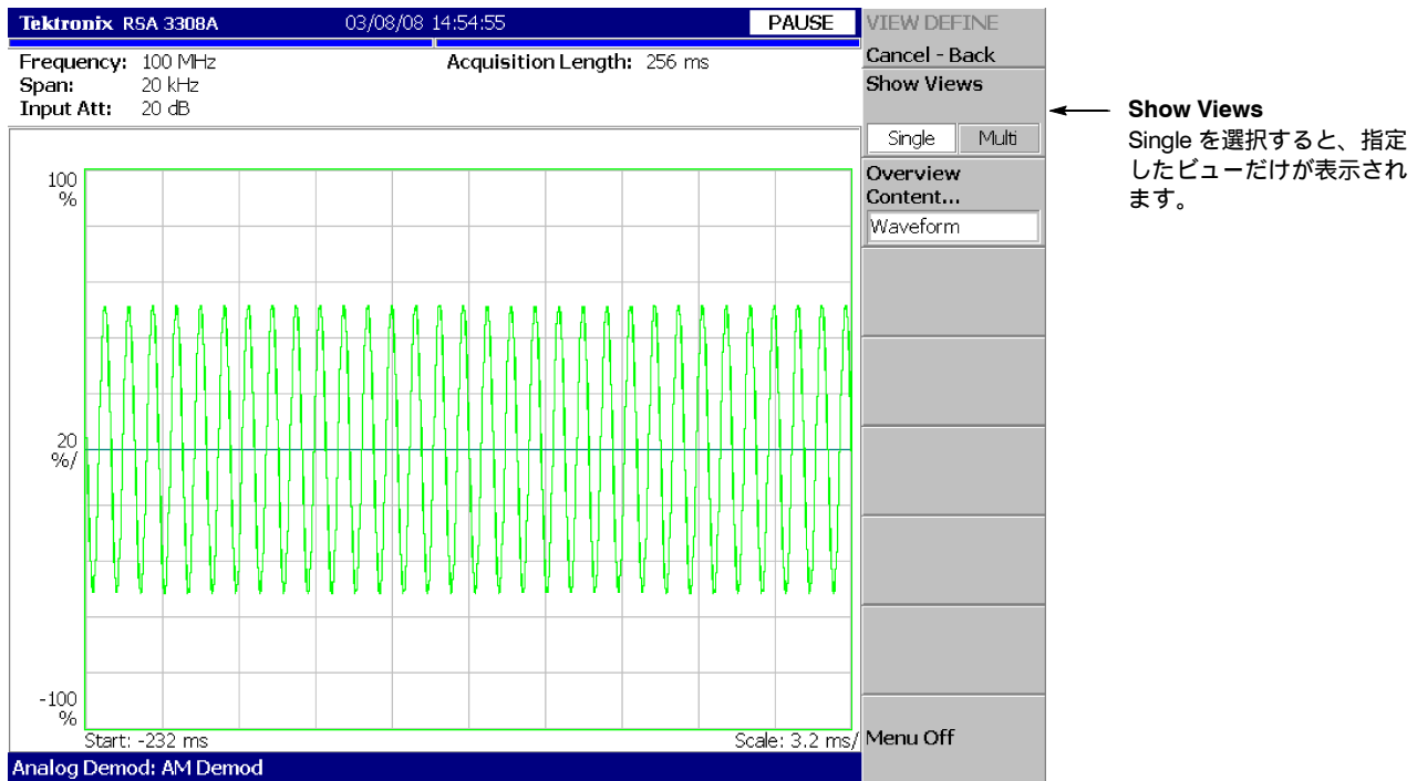
図 2-44 : 1ビュー表示
