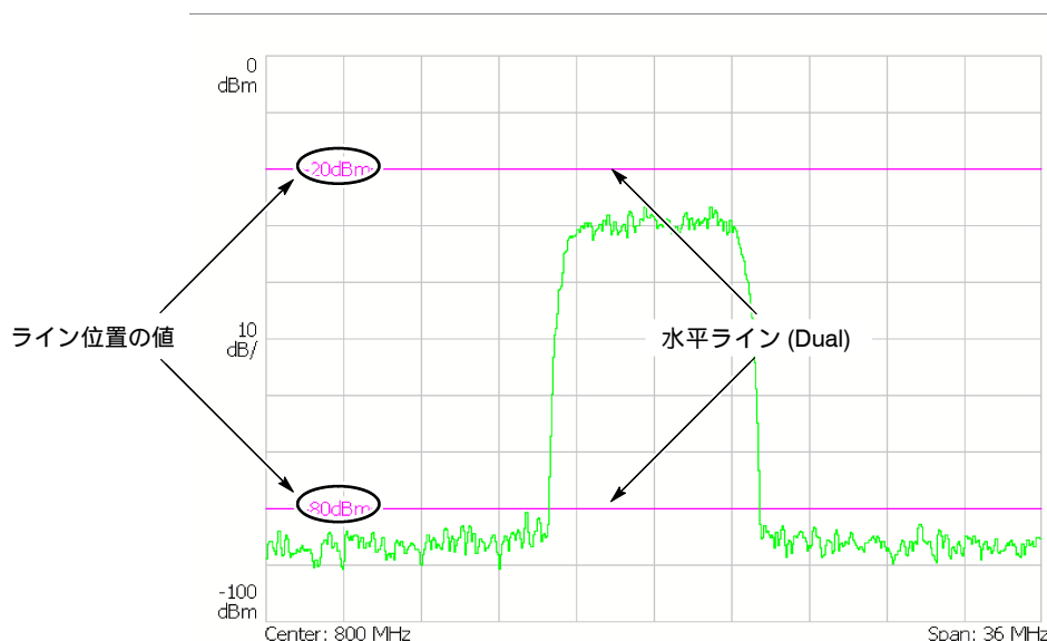
図 4-152 : 水平ライン
