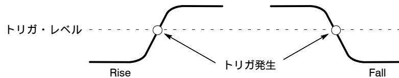
図 4-109 : トリガ・レベルとスロープ
