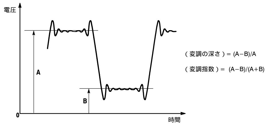
図 4-61 : 変調の深さと変調指数の定義
