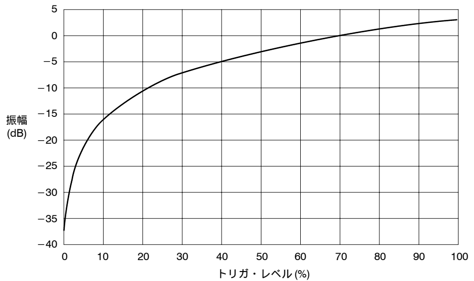
図 4-112：トリガ・レベル vs. 振幅 (リファレンス・レベル = +3dBm)
