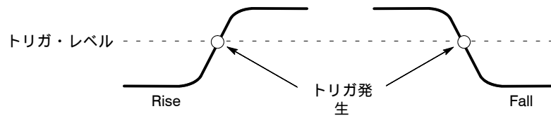
図 4-105 : トリガ・レベルとスロープ
