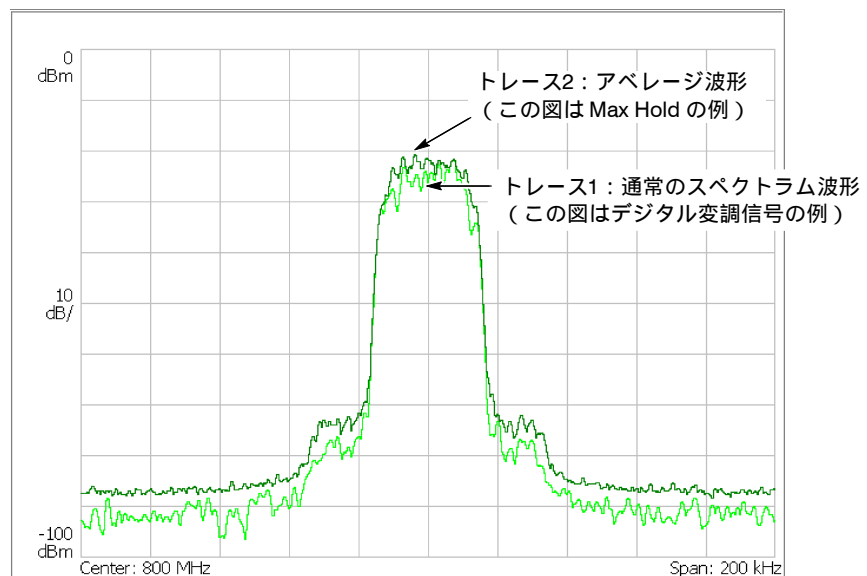
図 4-133 : 比較表示例
