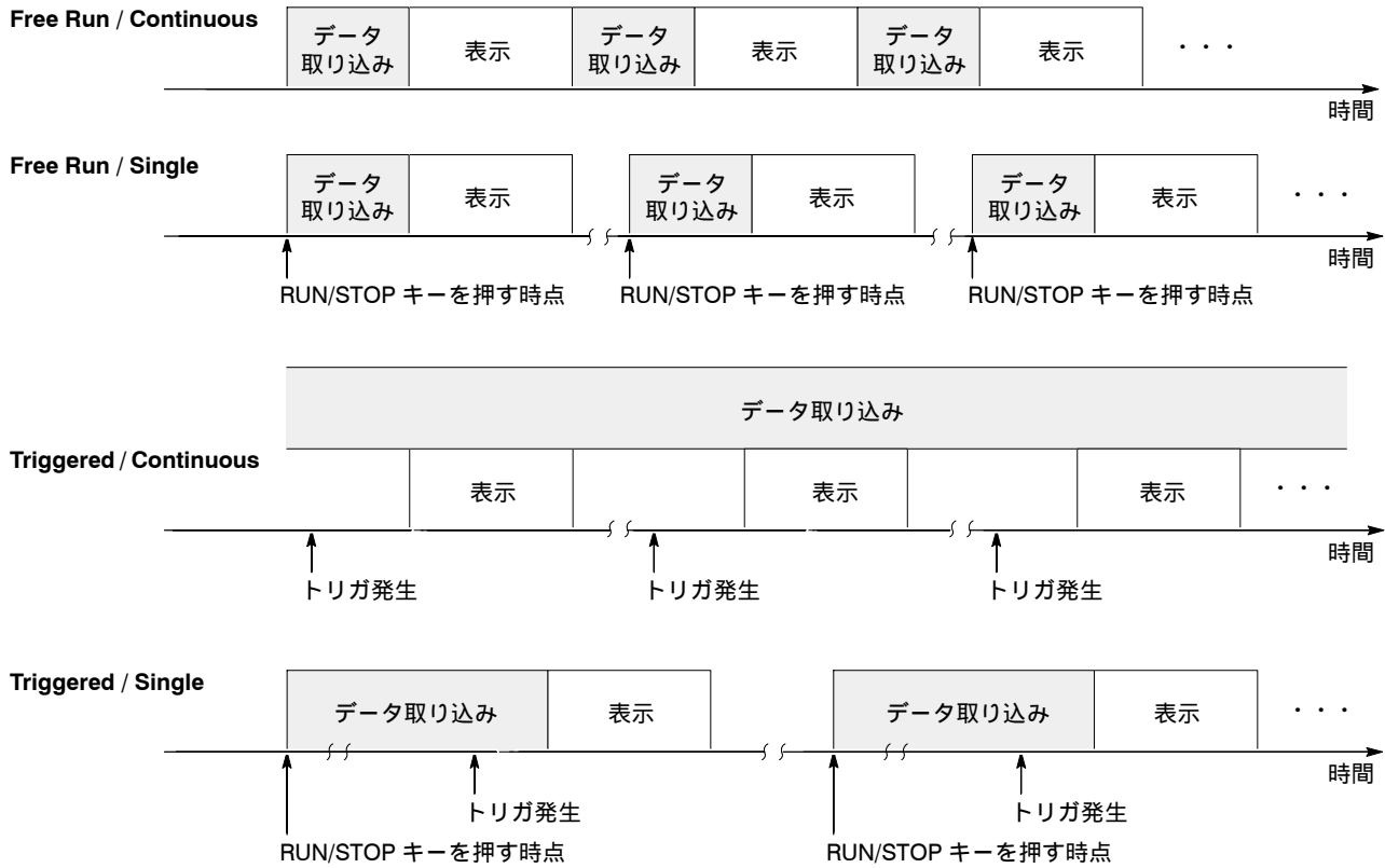
図 4-111：トリガおよびリピート・モードによるデータ取り込みと表示
