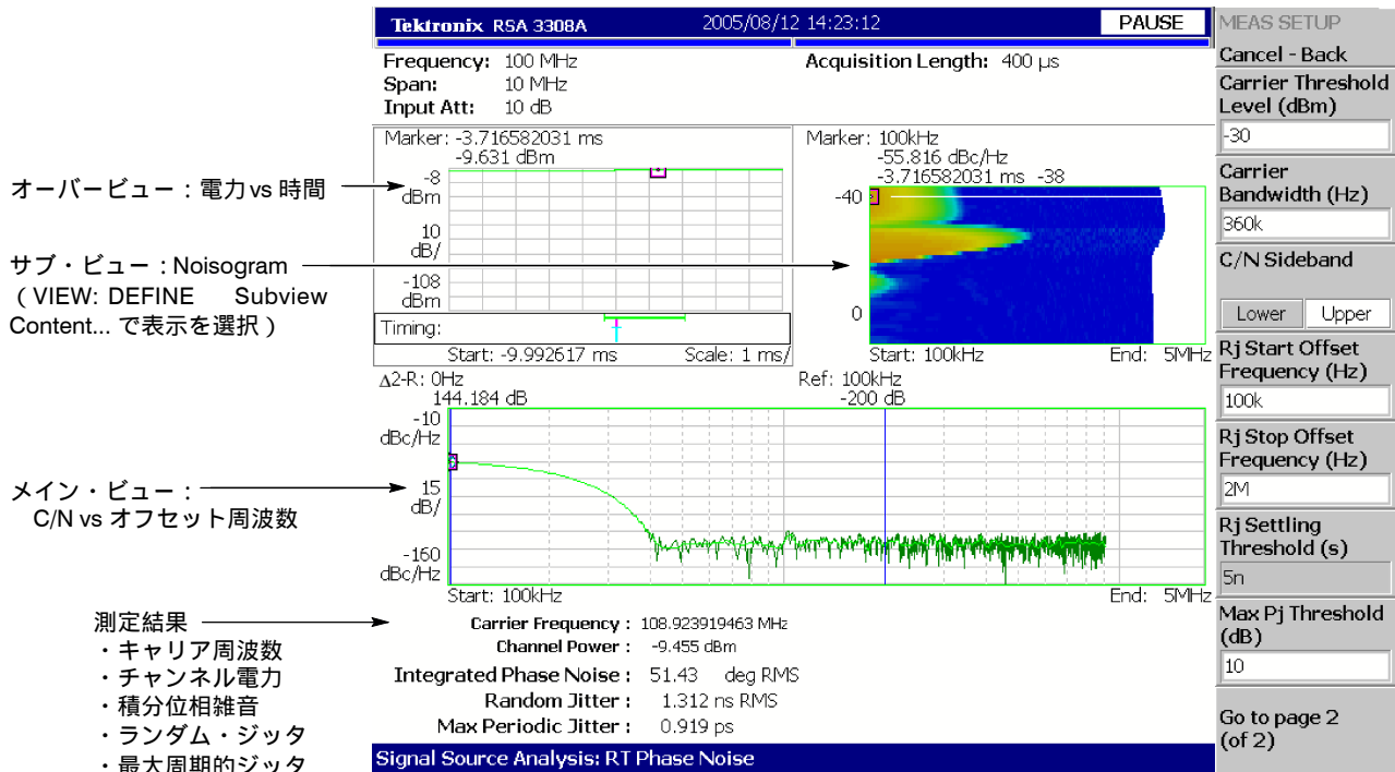
図 4-79：リアルタイム位相雑音測定
