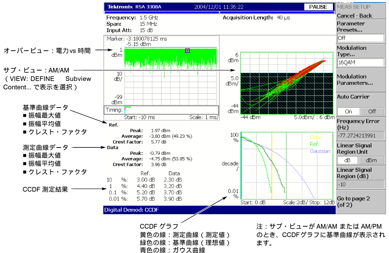
図 4-49：CCDF 測定例
