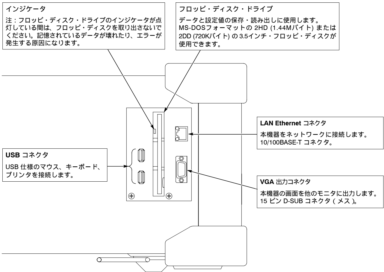
図 3-1 : 側面パネル
