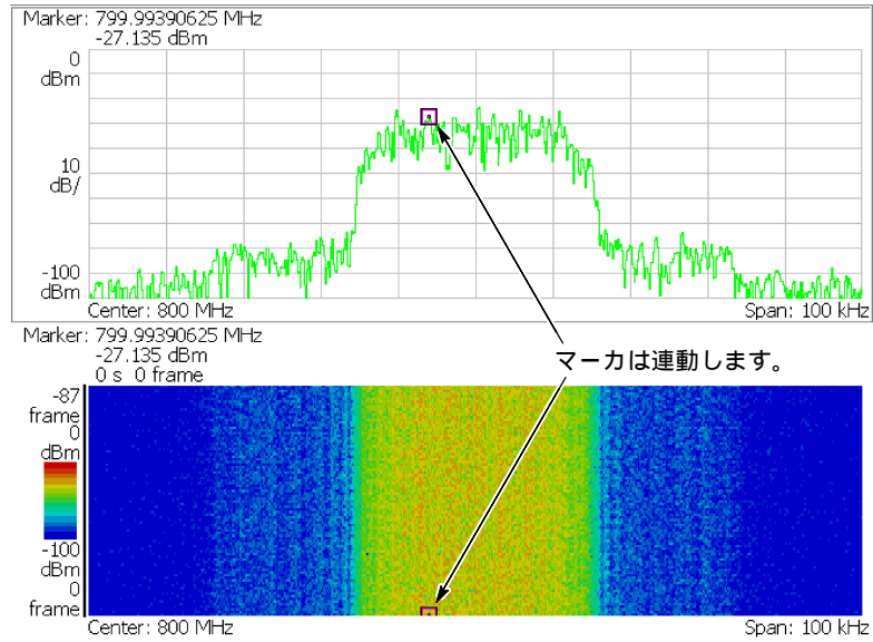
図 4-162 : マーカの連動
