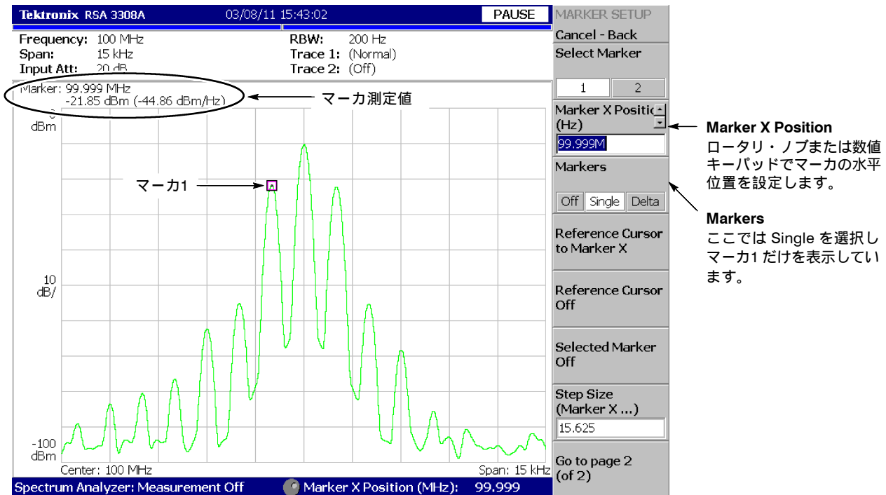
図 4-158 : メイン・マーカを使用した測定
