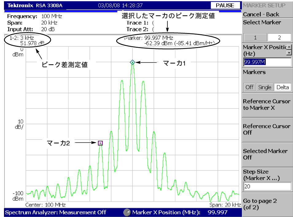
図 2-23 : ピーク検出
