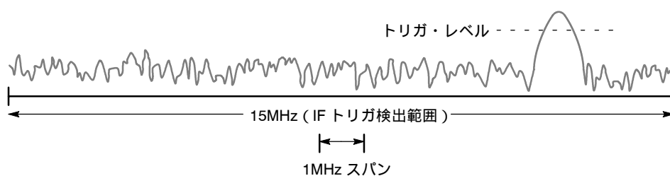
図 4-114 : IF トリガ検出範囲
