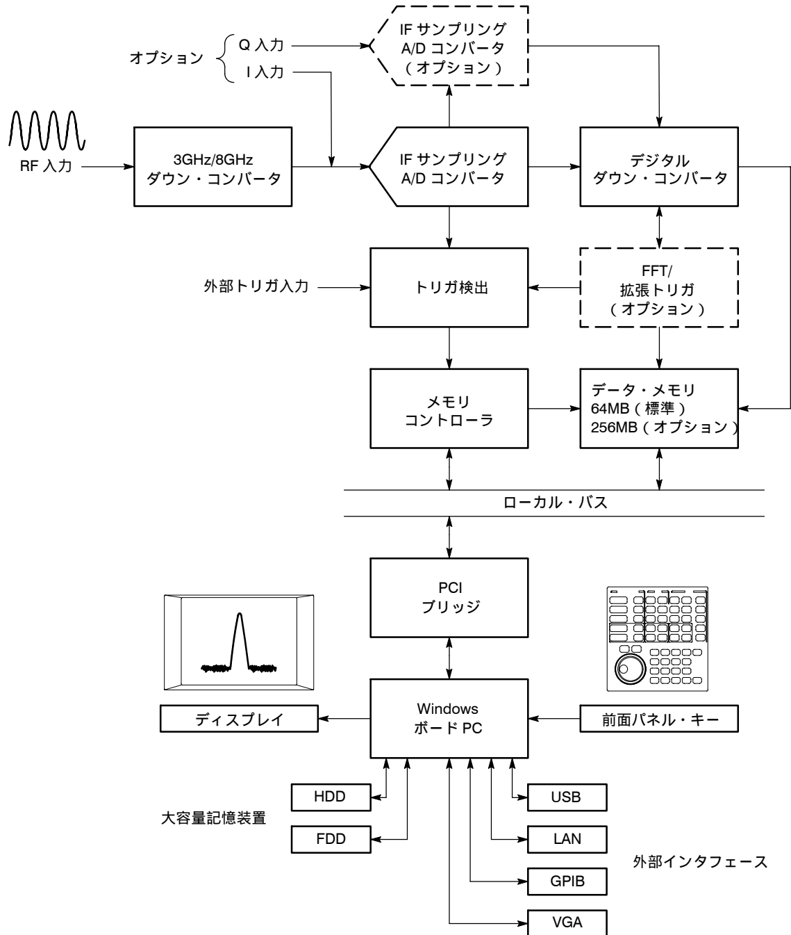
図 1-6 : ブロック図
