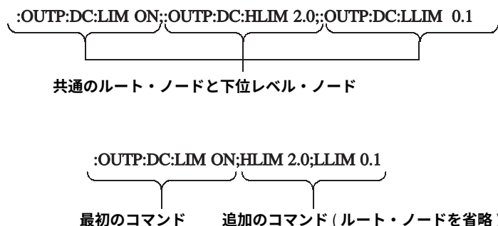
図 2-4：連結したメッセージ内での上位ノードと下位レベル・ノードの省略
