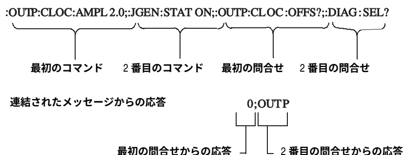
図 2-3：複数のコマンドと問い合わせの連結
