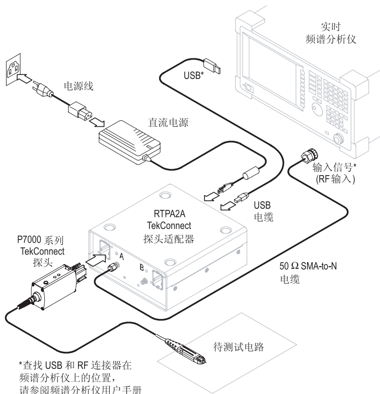
图 22: 安装 RTPA2A 探头适配器
