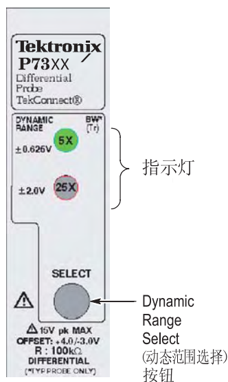
图 2：探头（前面）
