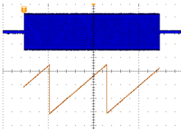
Rauschsperrung ein
