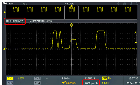
最大擷取的縮放波形記錄 (含 2000 點)
