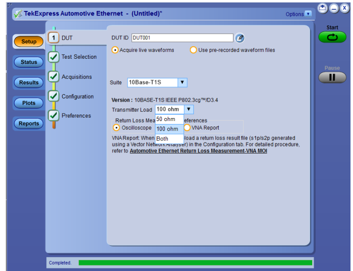
DUT setup
