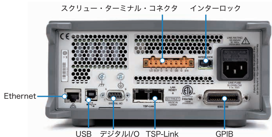
シグナル・インテグリティを維持し、迅速なシステム設定のため後部パネルのコネクタ、インターフェース
