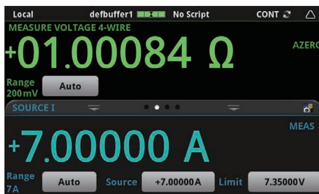
2460型のメイン・ホーム画面
