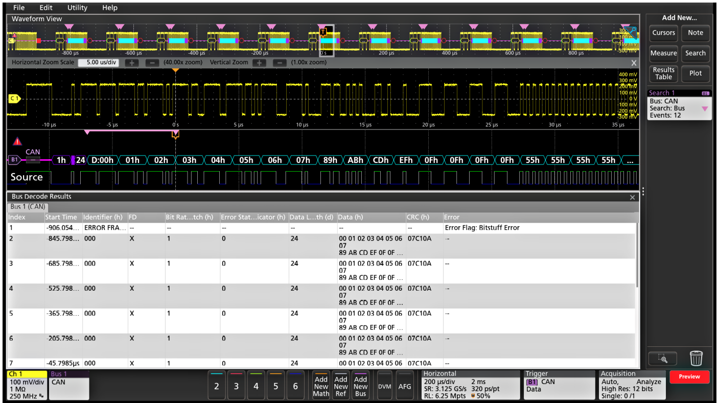
CAN シリアル・バスにトリガした例。バス波形は、スタート、アービトレーション、コントロール、データ、CRC、ACK など、時間相関のとれた、デコードされたパケットの内容を表示。バス・デコード・テーブルでは、アキュイジション全体のすべてのパケット内容を表示
