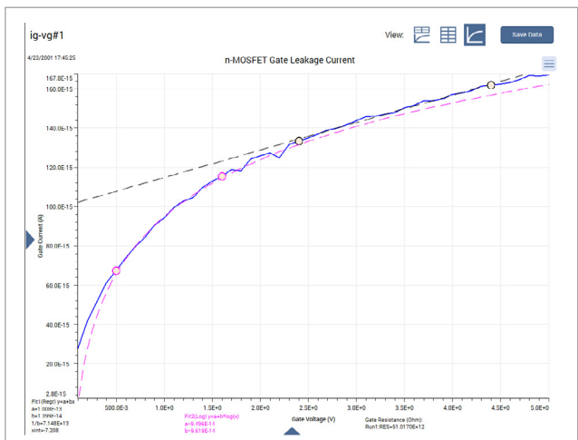
选配 4200-PA 前端放大器模块，支持 fA 级测量。
