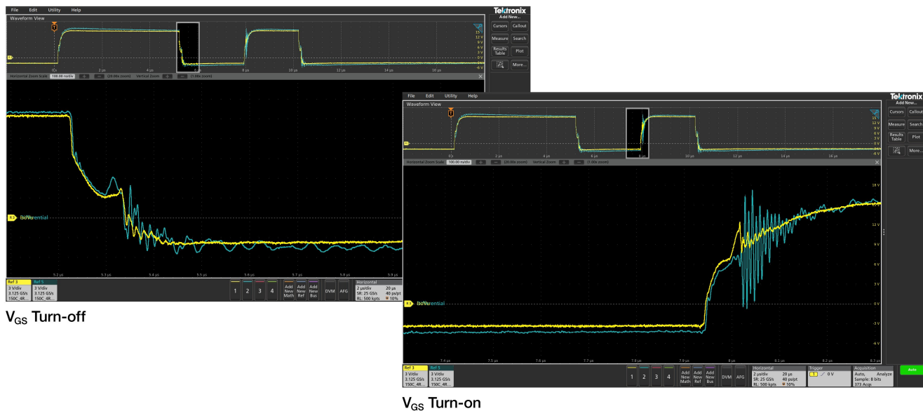
Differenzialtastkopf (blaue Messkurve) vs. IsoVu optisch isolierten Tastkopf (gelbe Messkurve)
