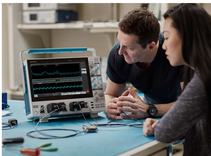
开关电源上的电压测量，显示了其中一条电源轨上的纹波电压。
