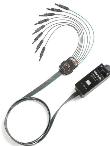
TLP058 提供了 8 个高性能数字输入。根据需要连接多只 TLP058 探头，支持最多 48 条数字通道。
