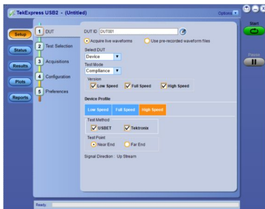
TekExpress USB 2.0 自動相容性測試設定功能表。
