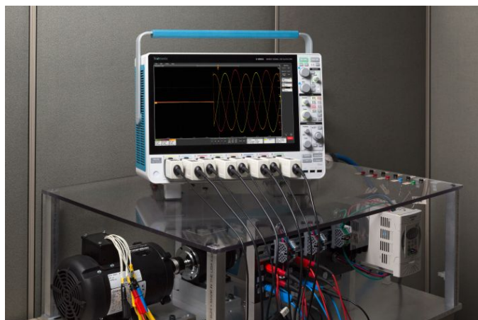
三相馬達啟動後會進行電壓量測，顯示三相位輸入電壓。
