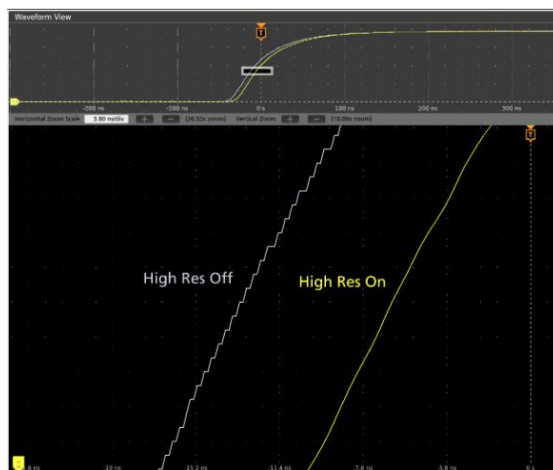
5 系列 MSO 的 12 位元 ADC，再結合新的高解析度模式，打造業界頂尖的垂直解析度。
