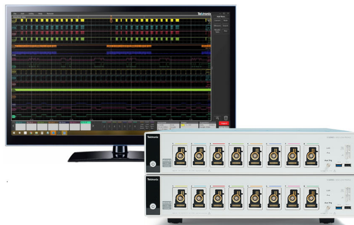
在运行 TekScope 'Multi-Scope' 的 PC 上分析两台 MSO58LP 仪器
