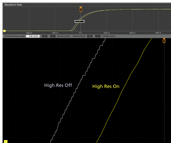
12 ビットの ADC と新しいハイレゾ・モードにより、業界トップクラスの垂直分解能を実現しています。
