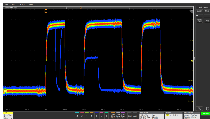
FastAcq の高速取込みにより、デジタル設計によく見られる捕捉困難な問題も検出できます。
