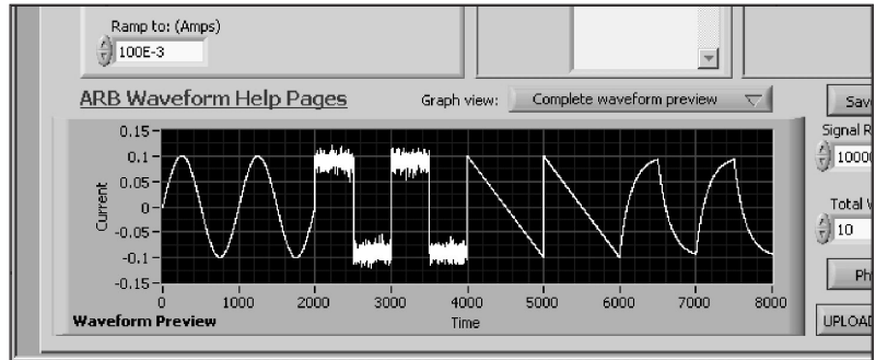
図 4 :6221 型および無償スタートアップ制御ソフトウェアを使用して、標準波形を加算、乗算、連結、フィルタリングすることで、複雑な波形を容易に作成可能
