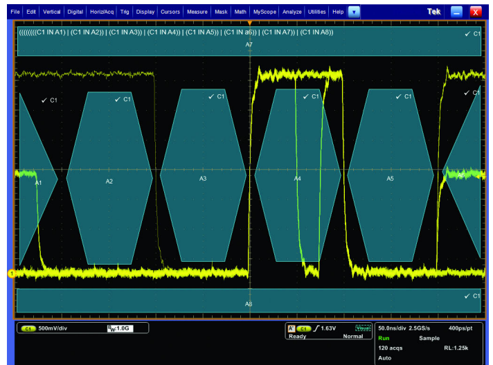
부울리(Boolean) 로직 트리거 자격. 로직 OR을 사용한 부울리(Boolean) 로직을 통해 사용자는 각 비트를 동시에 모니터링하고 획득의 모든 포인트에서 발생한 이상을 캡처할 수 있습니다.
