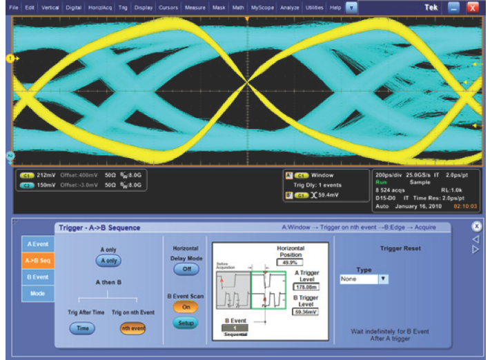
버스트에서 모든 비트의 아이 다이어그램을 구축하는 데 사용되는 DDR DQS 에지에서 B 이벤트 스캔 트리거를 사용합니다.
