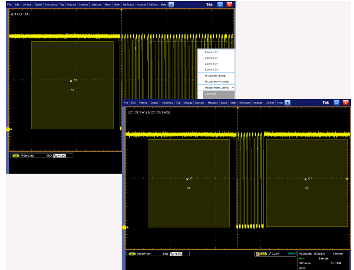
10 パルスのバースト幅にトリガした例。この例のように、最初のクロック・パルス前に Must be outside の領域を、10 パルス後に Must be outside を設定することにより、目的のバースト幅を取込むようにビジュアル・トリガを設定可能
