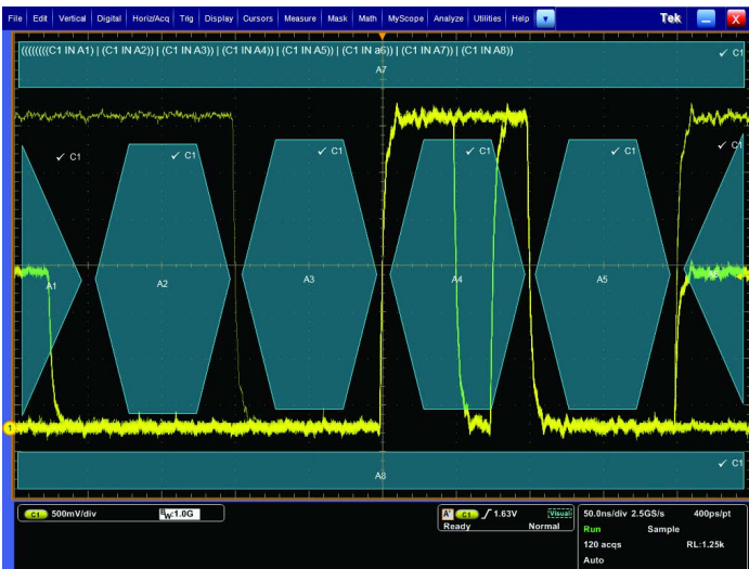
ブール・ロジック・トリガ・クオリフィケーションの例。ロジック OR を使用したブール論理により、各ビットを同時にモニタし、任意のポイントにおける異常を取込むことが可能
