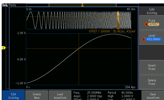
Arbiträr-/Funktionsgenerator-Editor mit Anzeige des Punkt-für-Punkt-Editors.
