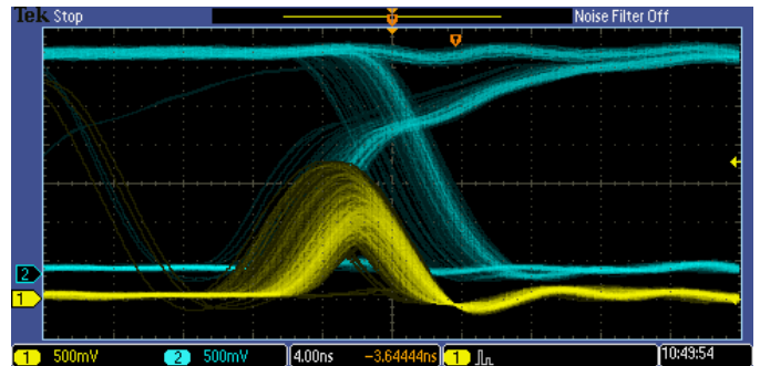
MSO/DPO2000B シリーズに搭載したデジタル・フォスファ技術で実現される、毎秒 5,000 波形の取込レートとリアルタイムな輝度階調表示
