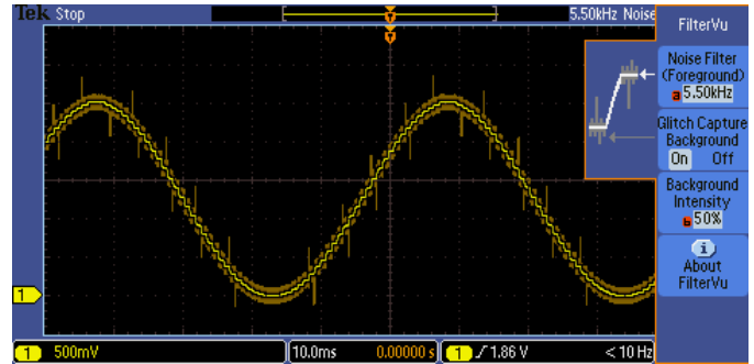
DAC 訊號輸出 - 請見 FilterVu™ 如何以前景軌跡（黃色）清楚顯示 DAC 的無雜訊階段，此軌跡移除了所有 5.5 kHz 以上的頻率。FilterVu 也會擷取達示波器完整頻寬的高頻突波，並加以顯示於背景軌跡（橘色）。
