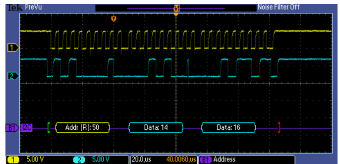
通過 I 2 C 匯流排的特定資料封包觸發。黃色波形表示時脈，藍色波形表示資料。匯流排波形提供解碼封包內容，包括 Start（起始）、Address（位址）、Read/Write（讀取/寫入）、Data（資料）和 Stop（停止）。
