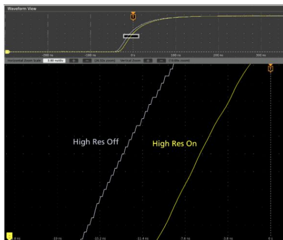
6 系列 MSO 的 12 位 ADC 及新型 High Res 模式实现了业界领先的垂直分辨率。
