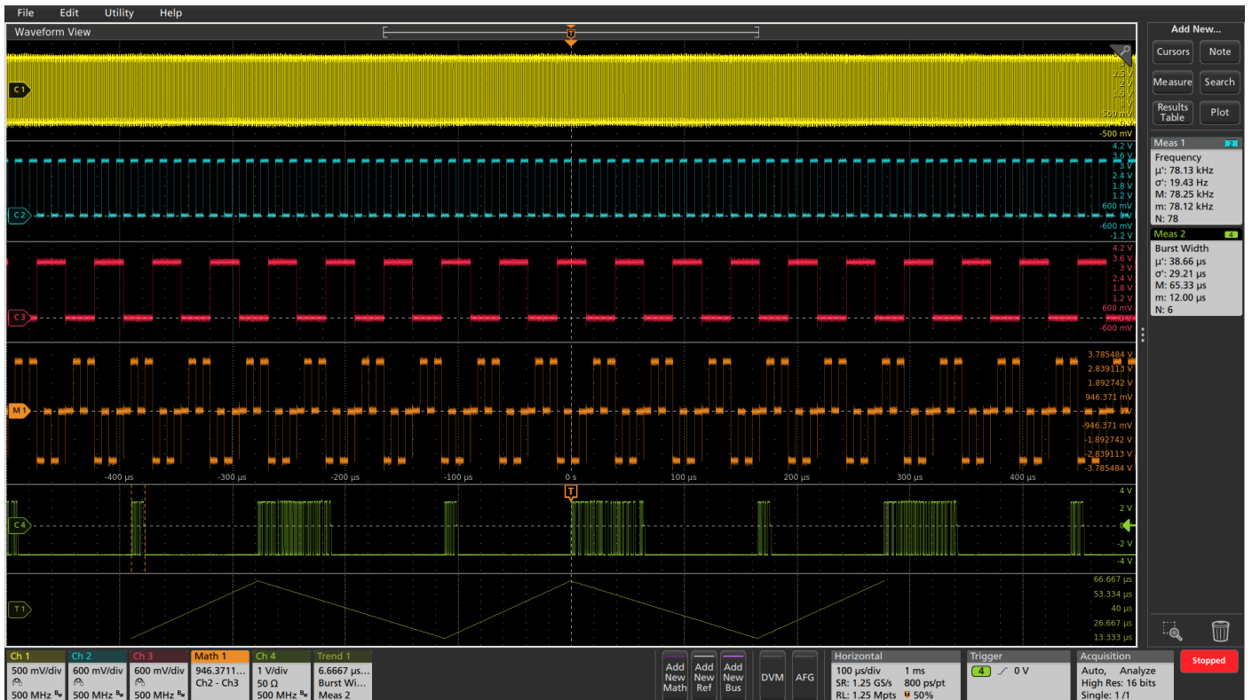
使用测量功能表征突发宽度和频率。
