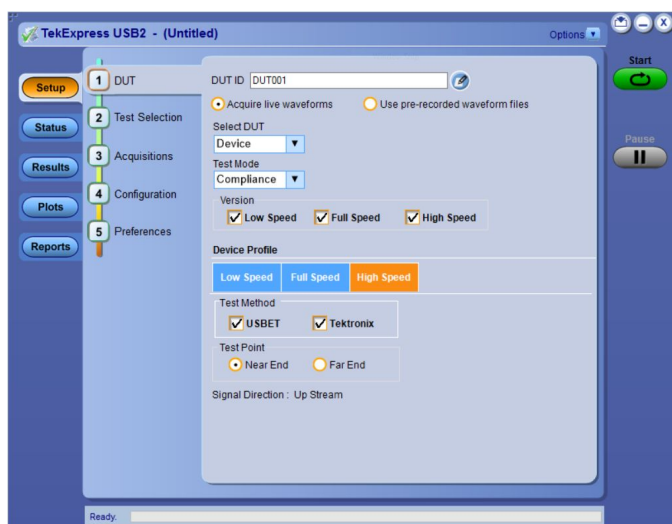
TekExpress USB2 (選項 6-CMUSB2) DUT 面板設定 DUT 特定的設定
