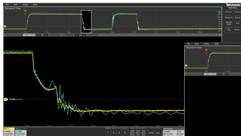
V_{GS} Turn-off
