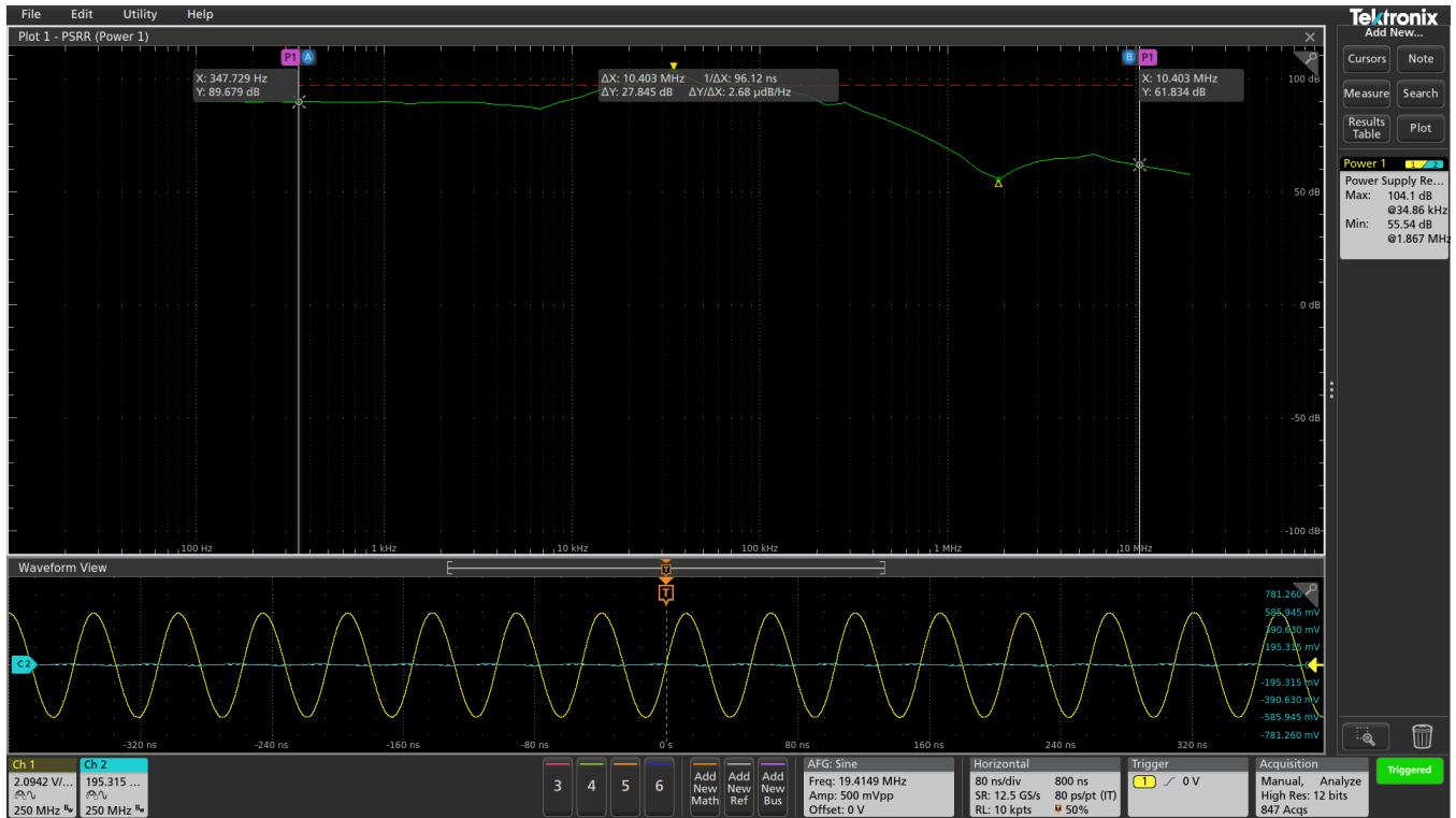
電源電圧変動除去比 (PSRR) の測定：周波数対除去比のプロットとともに、最小値と最大値も表示されます。
