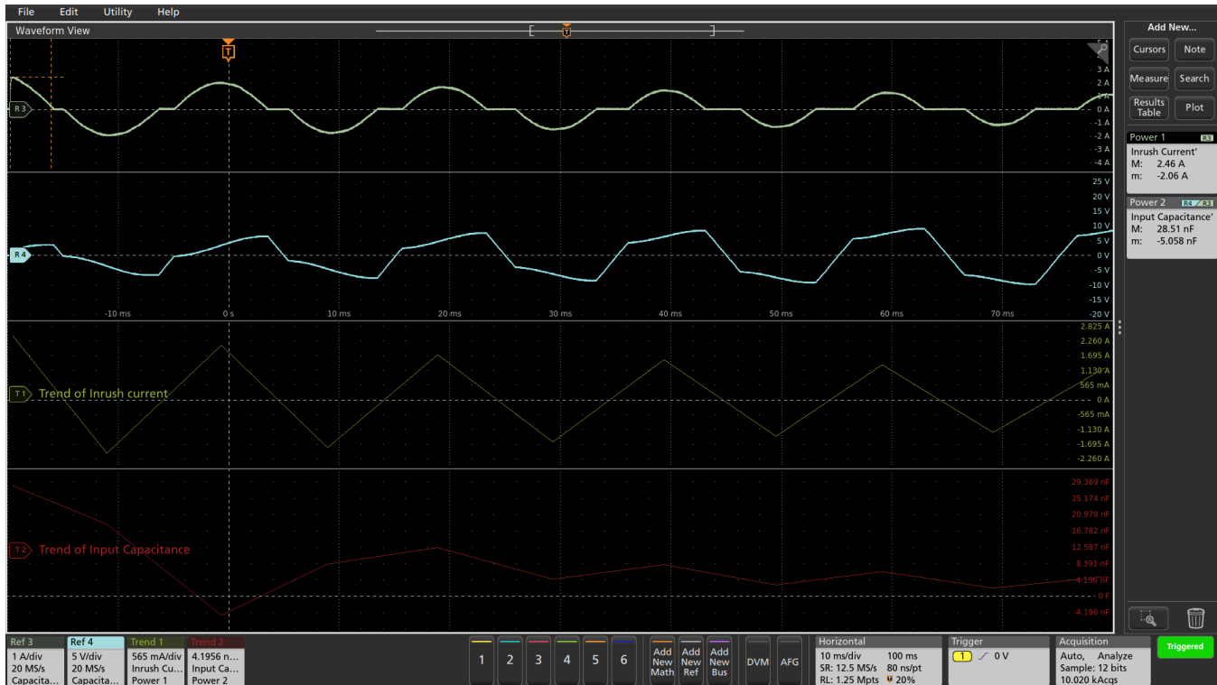
トラバース機能による入力キャパシタンス／突入電流測定
