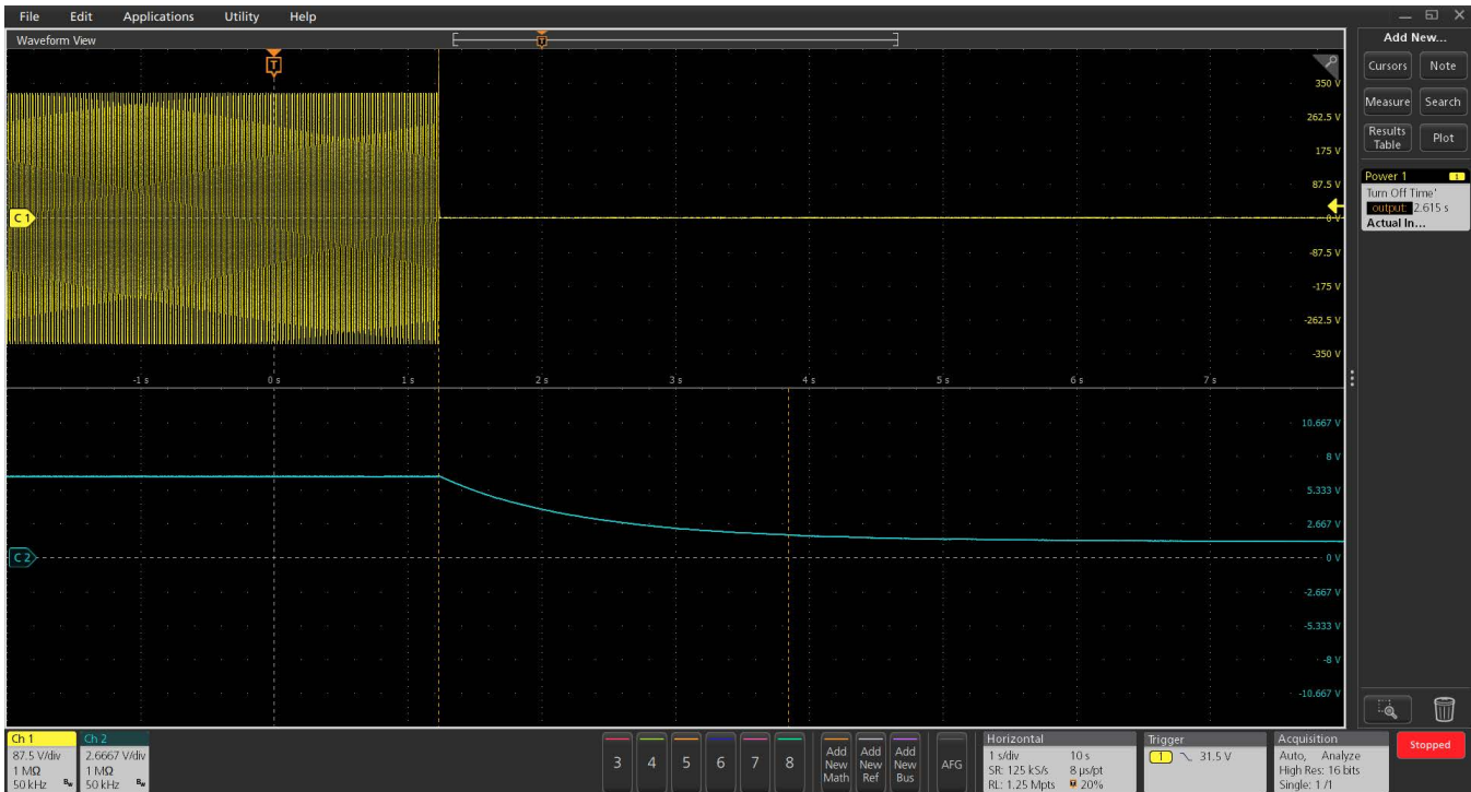
ターン・オフ時間測定
