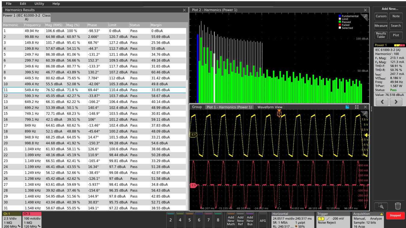
高調波のバー・グラフ、高調波の測定結果表、結果バー（右上）を使用したトラバース機能
