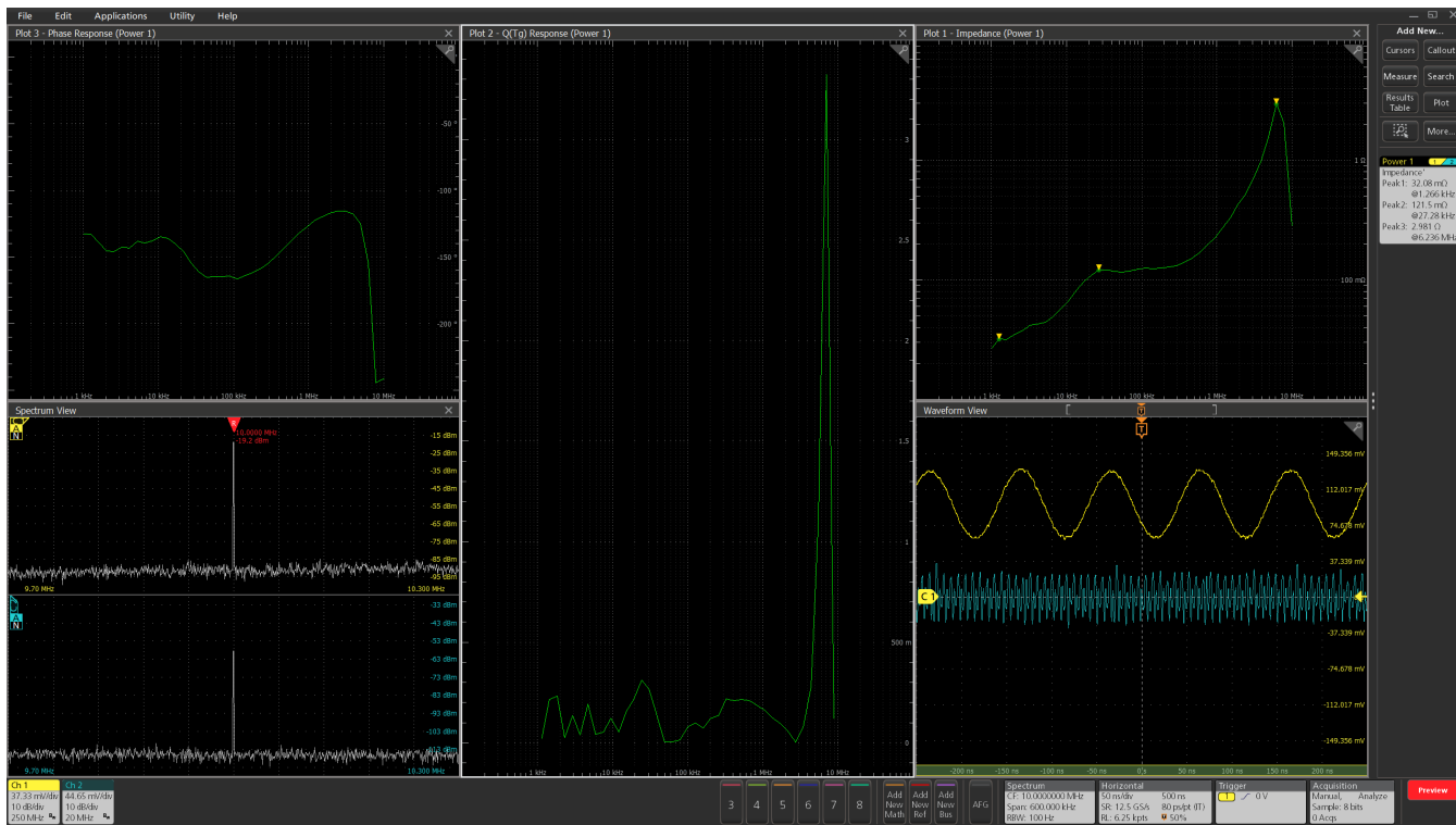
インピーダンス測定：測定結果表と結果バッジにピーク・インピーダンス・ポイントの値が表示されている対応するインピーダンス・プロット、グループ遅延プロット、位相プロットも表示されます。
