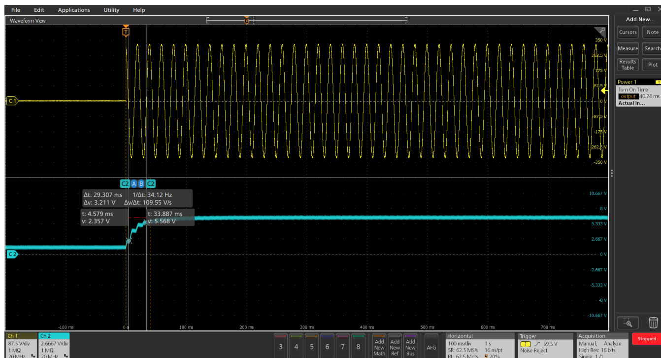
ターン・オン時間測定
