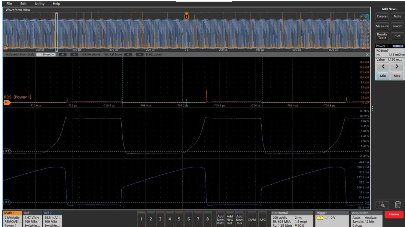
R DS(on) の測定
