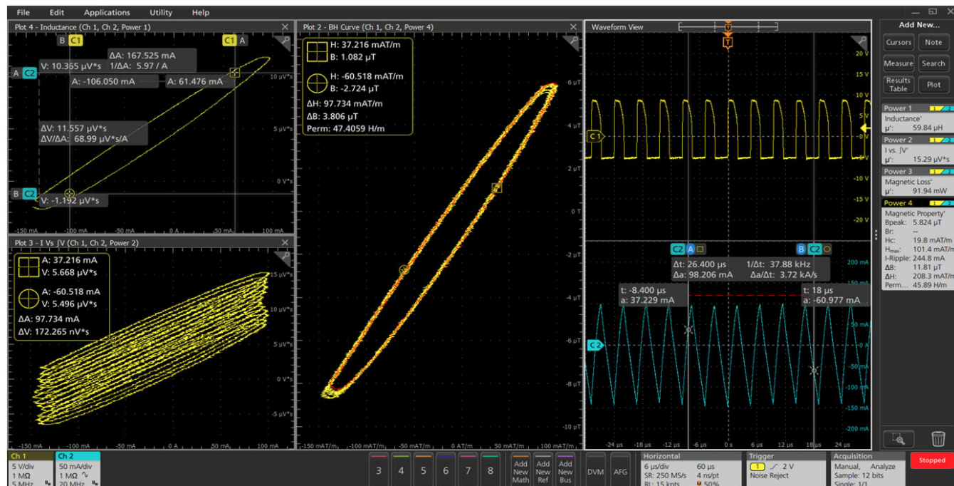
磁気解析／測定 (B-H 曲線、I対V、インダクタンスのplot)
