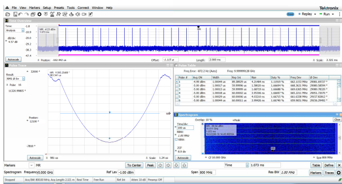
上图显示了宽 700 MHz 的线性调频信号。时间总览出现在画面顶部，显示当前采集中的脉冲。相位偏差显示在左面，表明了线性调频的抛物线特性。信号在重复时段有变化，脉冲表和右侧频谱图均显示了这些变化。
