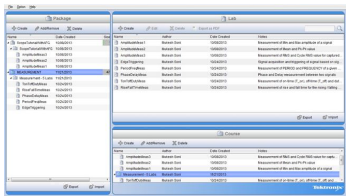
课件 PC 界面使用 Labs 构建课程。然后使用课程构建包，包上传到示波器中。
