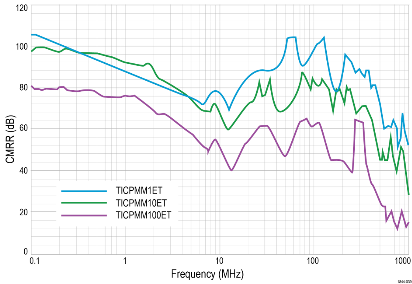
极端温度下探头共模抑制比 (CMRR)
