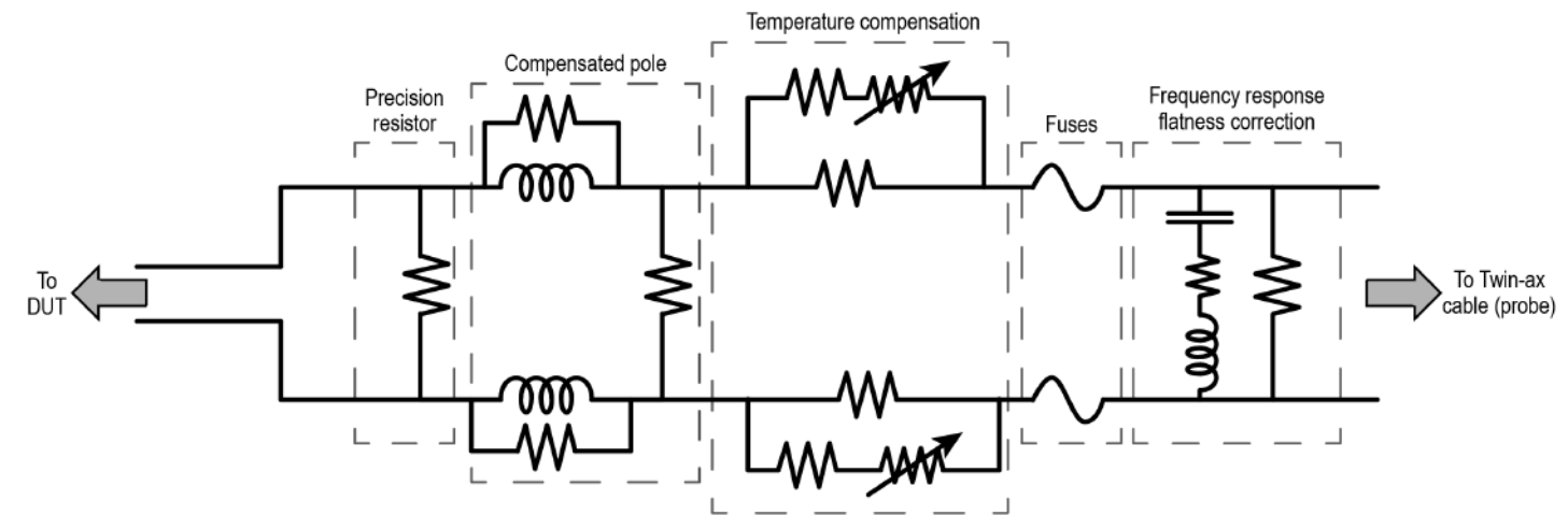
宽带分流器框图
