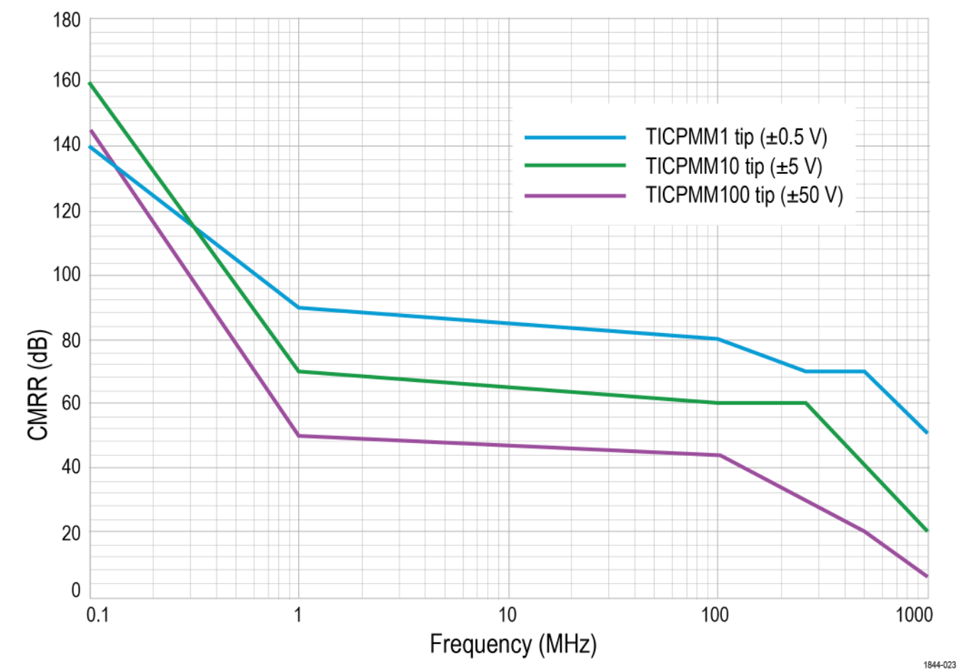
IsoVu隔离电流探头的共模抑制比（CMRR）
