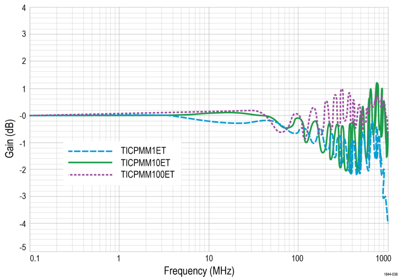
极端温度下尖端频率响应
