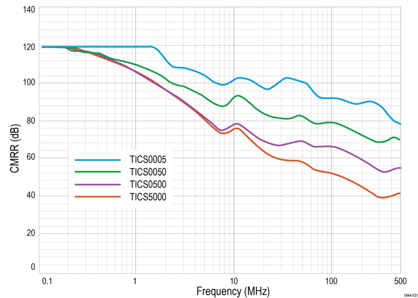
宽带分流器的共模抑制比（ CMRR ）
