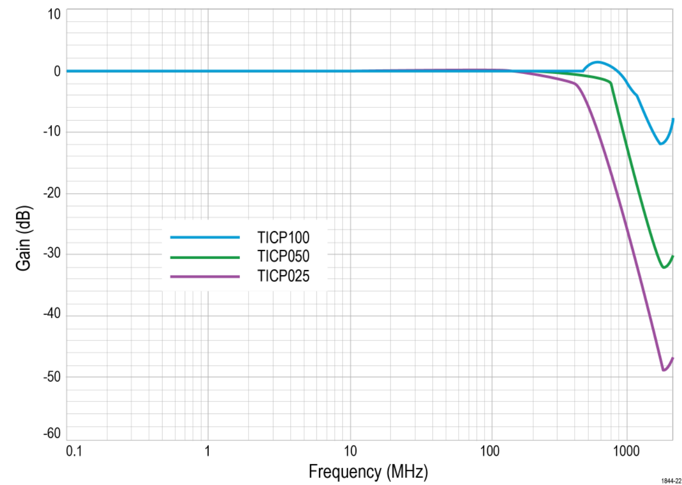
IsoVu 隔离电流探头的频率响应
