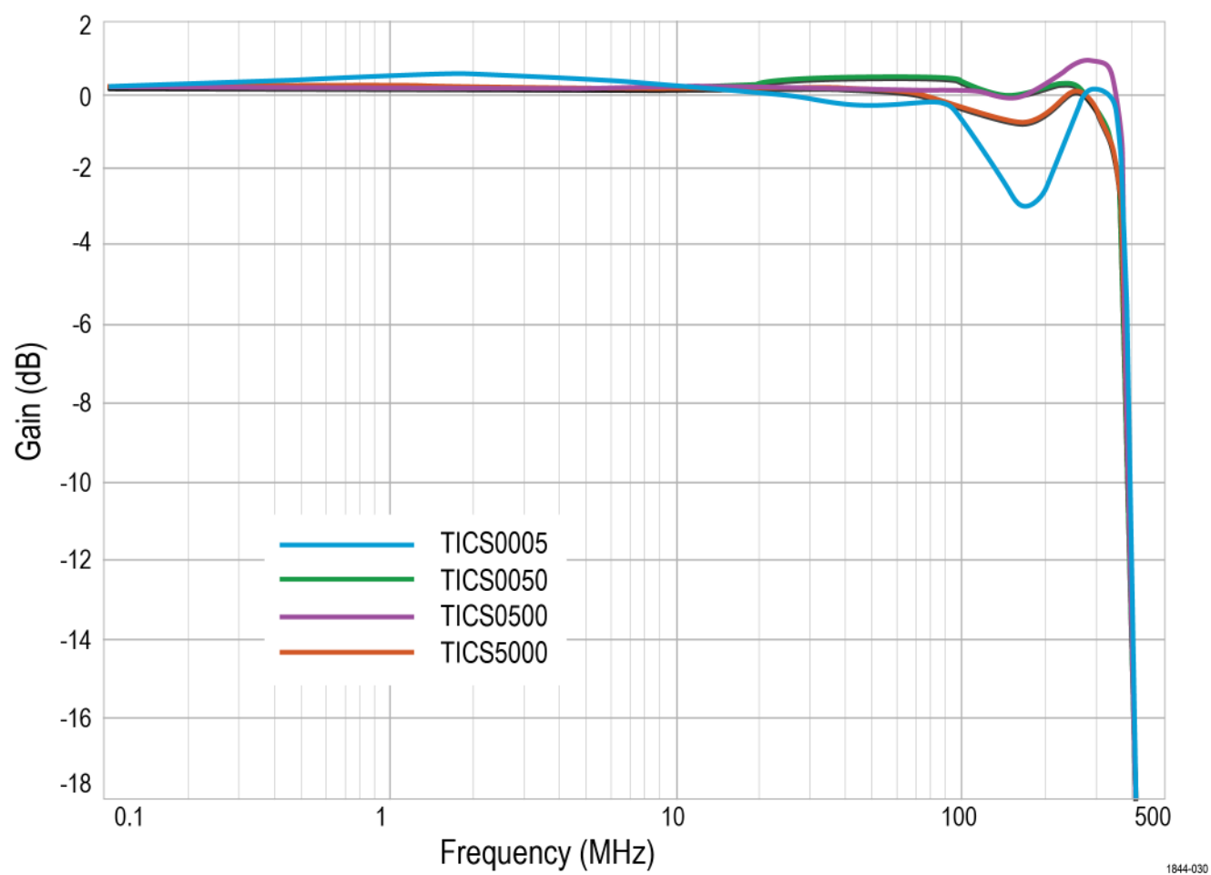
宽带分流器的频率响应
