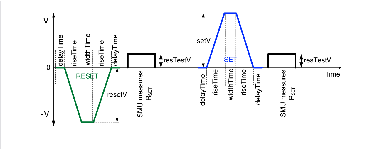
图 43. reramSweep 和 reramEndurance 测量的脉冲波形。
