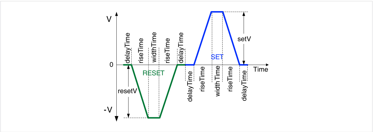
图 44. 压力 reramEndurance 的脉冲波形参数。
