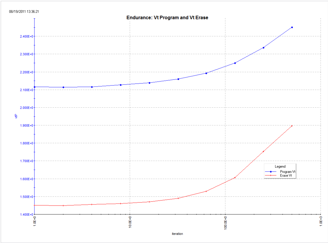
图 15. 来自闪存耐受性测试 (用户模块 flashEndurance) 的 NANDw 存耐受性结果。
