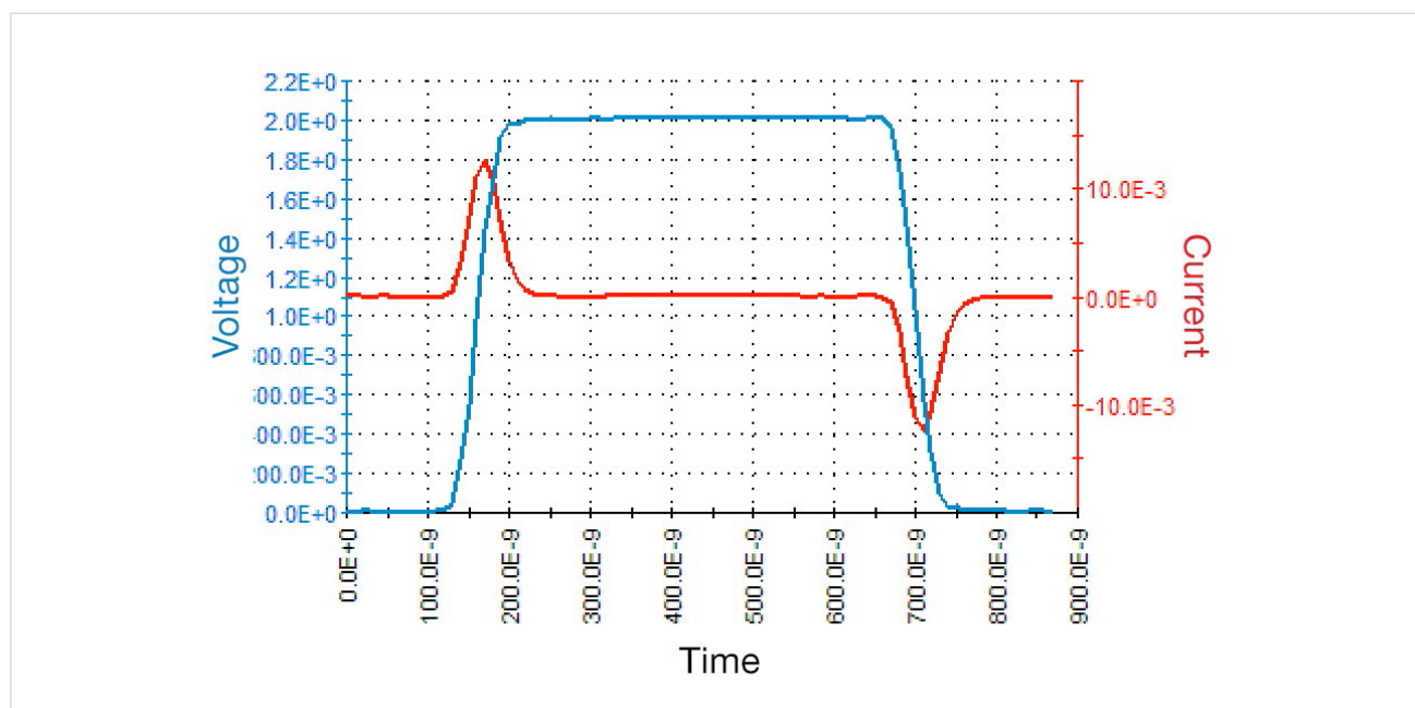
图 49. 电容充电效应。蓝色曲线是应用到同轴电缆短长度上的电压脉冲。红色曲线是得到的电流流动，是从应用的电压脉冲同一侧测得的（图 48 或图 50 中的通道 1）。充电效应是电压脉冲跃变过程中红色曲线的隆起部分。
