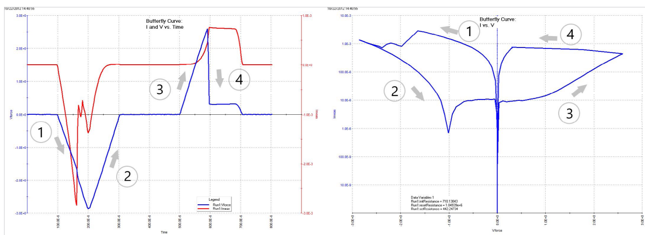
图 41. ReRAM “蝴蝶”曲线。
