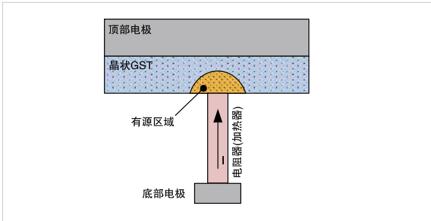
图 18. GST [ 锗 (Ge)、锑 (Sb) 和碲 (Te) ] 结构。
