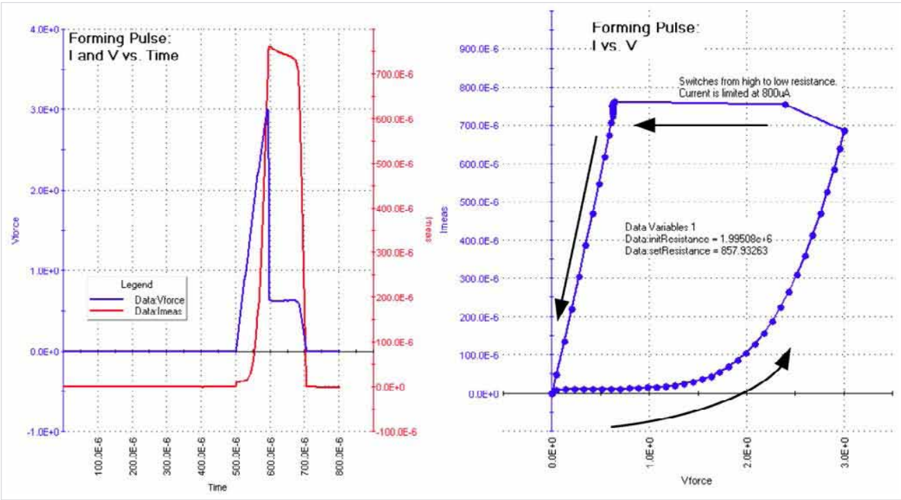
图 40. ReRAM 成形。
