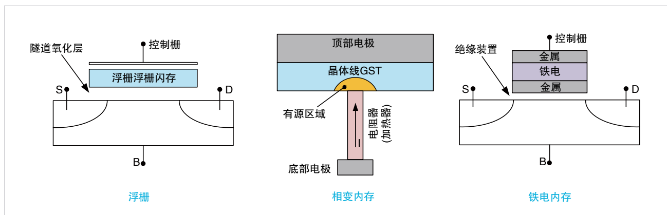
图 1. 各种非易失性内存器件。
