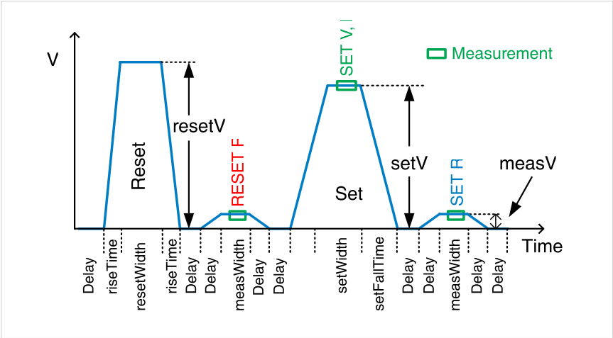
图 28. PRAM 波形定义。
