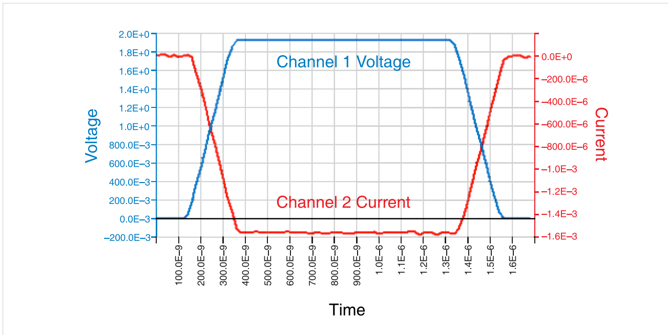
图 51. 图 50 所示的配置的脉冲 I-V 波形。在脉冲跃变过程中看不到电容充电电流，只看到电流流经电阻器 DUT。
