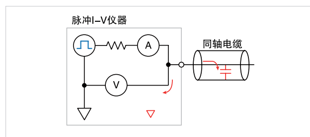
图 48. 脉冲 I-V 仪器方框图，显示了脉冲跃变过程中的电容充电电流。
