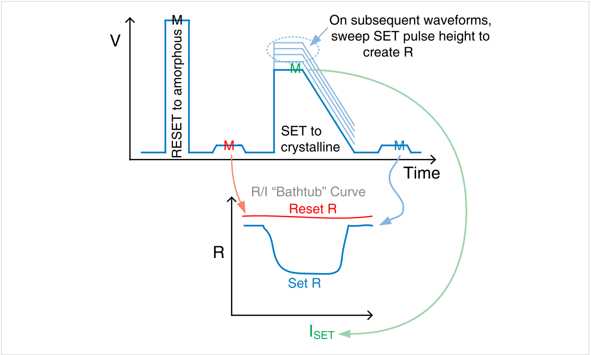
图 25. 这个图解释了怎样使用各种测量确定 R-I 曲线。在测量 RESET 电阻 (红色 M)、SET 电流 (绿色 M) 和 SET 电阻 (蓝色 M) 的同时, 会扫描 SET 曲线。
