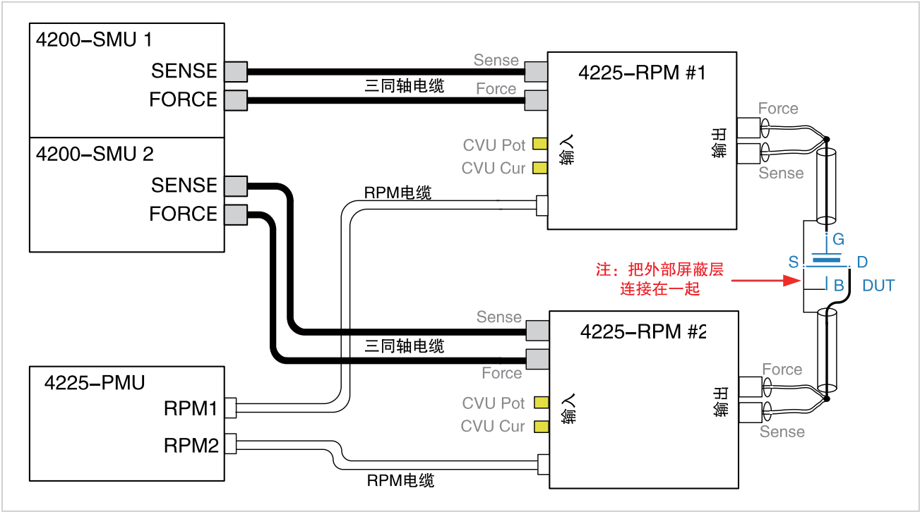
图 12. 连接 4 端子浮栅浮栅闪存器件。
