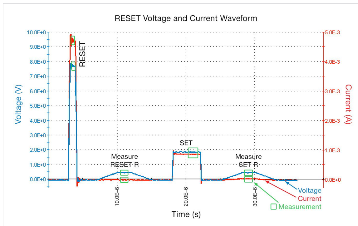
图 23. 4225-PMU 及 4225-RPMs (用户模块 pramSweep) 生成和测量的 R-I RESET-Measure-SET-Measure 波形。这个图显示了电压 (蓝色, 左面 y 轴) 和电流 (红色, 右面 y 轴) 波形。这个波形内部有四个脉冲。第一个脉冲是 RESET 脉冲, 重设 PRAM 材料, 把它置入高阻抗非晶相状态。第二个脉冲测量 RESET 状态的电阻。第三个脉冲是 SET 脉冲, 把材料置于低电阻晶相状态。第四个也是最后一个脉冲, 测量材料在 SET 状态下的电阻。图 24 是一条 R-I 曲线, 是扫描 SET 脉冲高度, 在 R-I 曲线中绘制结果图得到的。
