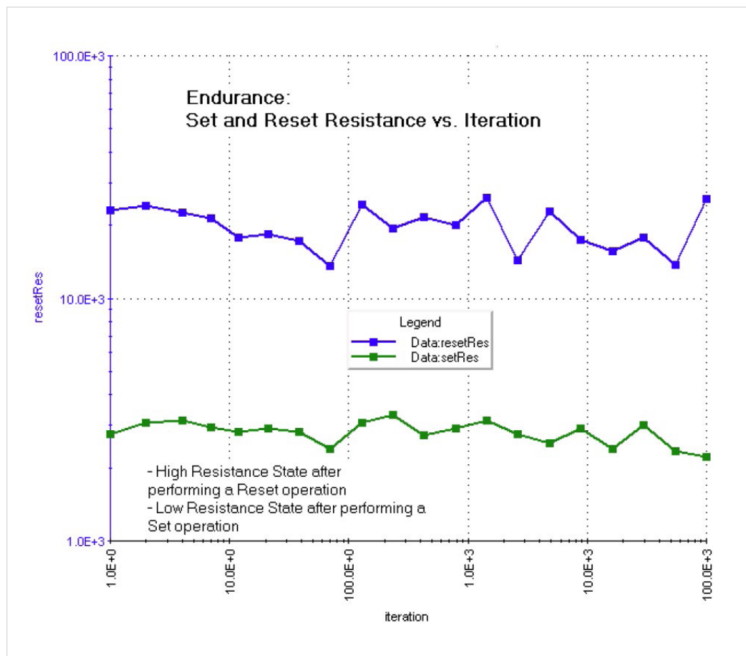
图 42: ReRAM 耐受性测试。
