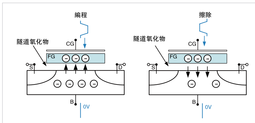
图 10. 闪存结构，显示了 Fowler-Nordheim 隧道的编程和擦除条件。
