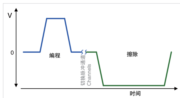
图 5. 闪存编程和擦除波形：两种脉冲，三种电平。传统脉冲发生器只能输出两电平脉冲，因此闪存测试对每项测试要求两条脉冲通道，并要求一个耗时的开关对测试器件应用第二个（负）脉冲。注意这个设置只适用于一个器件端子。对栅极和漏极上的典型脉冲传送，必须重复这一设置。
