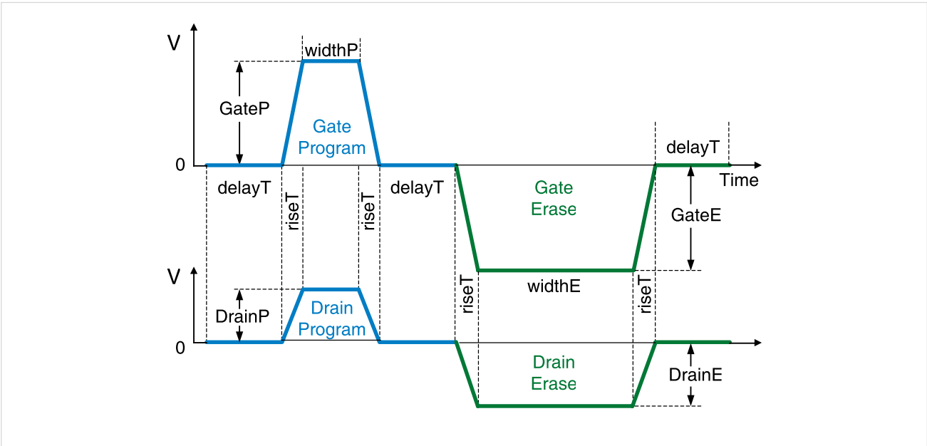
图 16. flashProgramErase 模块的波形参数。
