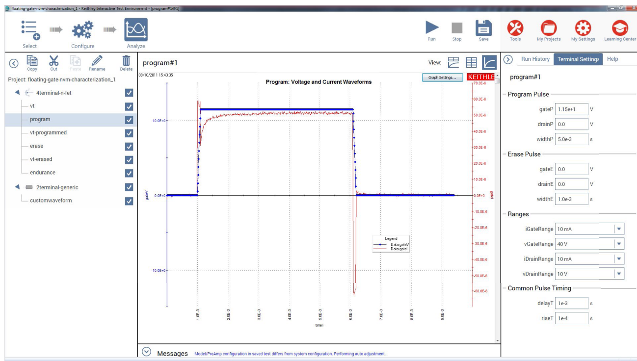
图 9. 浮栅非易失性内存表征项目截图。
