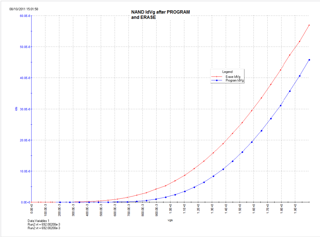
图 14. VT 扫描, 使用 SMU 从 vt-erased 测试 (用户模块 vt_ext) 中获得编程和擦除的单元。在这个图中, 编程后和擦除后的 VT 差约为 180mV。
