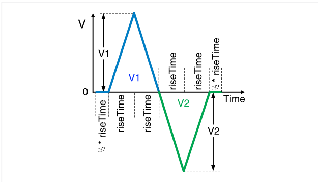
图 27. doubleSweep 的多脉冲波形。
