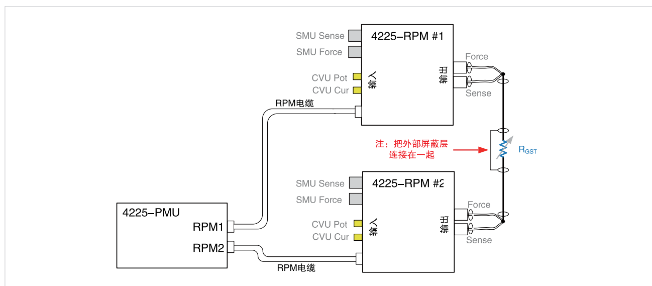
图 19. PRAM 测试连接图。注意 PRAM 测试不使用 SMU 或 CVU。
