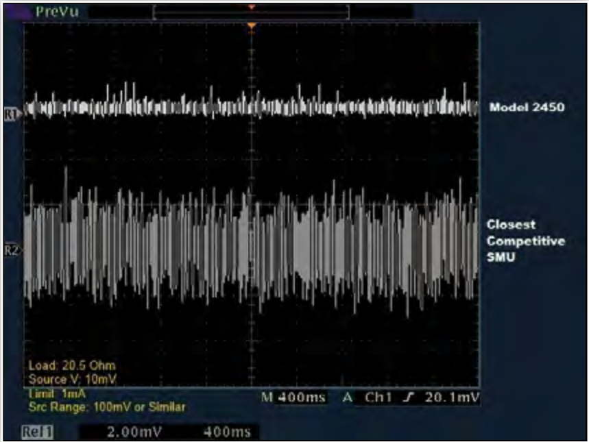
由于宽带噪声比竞争产品大幅降低，2450仪器成为下一代器件I-V测试的完美解决方案
