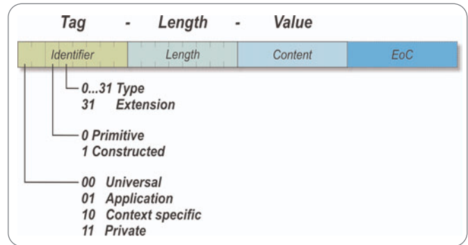
► Figure 3. Parameter Encoding in ASN.1.
