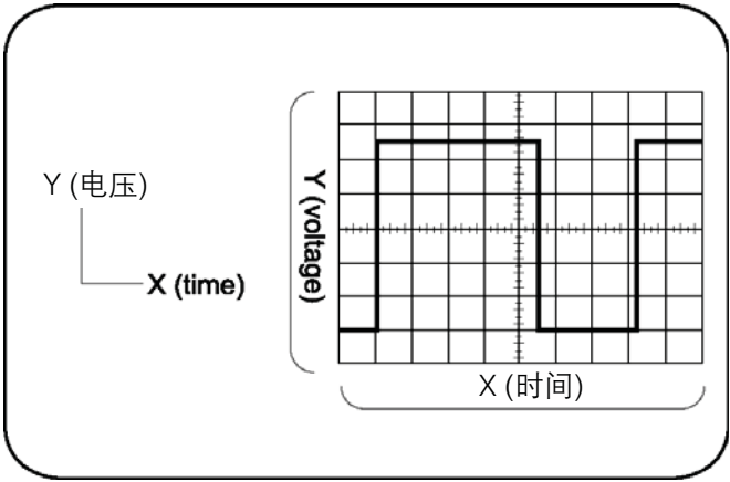
图1. 典型的示波器显示画面。
