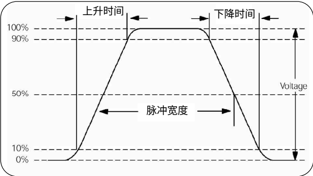
► 图69. 上升时间和脉冲宽度测量点
