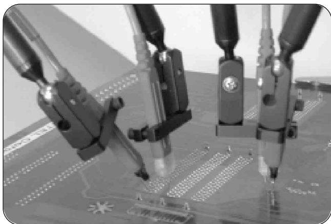
► 图42. 现代计算机总线和数据传输线具有快速时钟和边缘，在测量时高性能的探头非常重要
