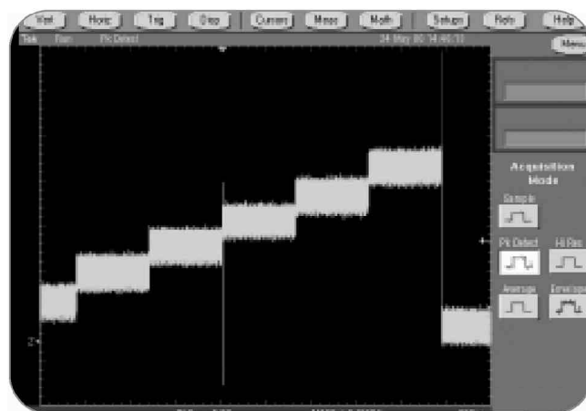
► 图27. TDS7000 系列示波器采用峰值检测模式能够捕获窄到100ps 的瞬态异常
