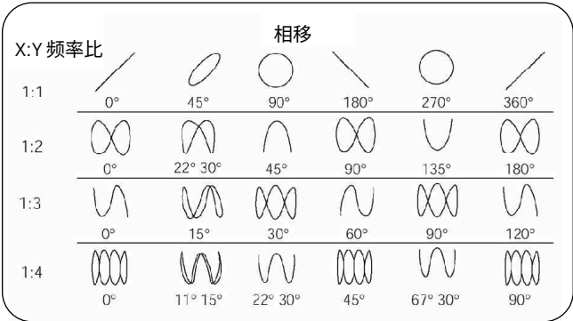
图70. 李萨如模式
