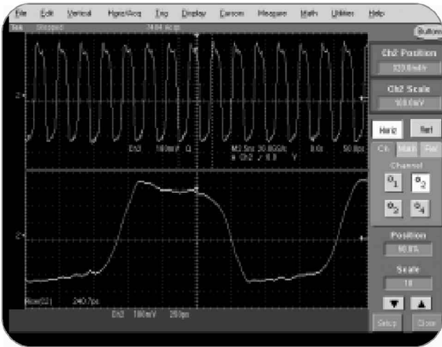
► 图48. 高速数字信号的上升时间特性
