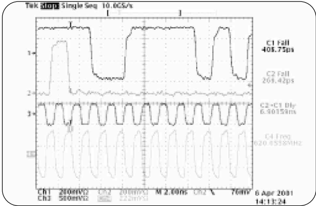
► 图17. TDS694C 提供多通道同时的高速单次脉冲捕获，增加了对偶发毛刺和瞬态现象的捕获
