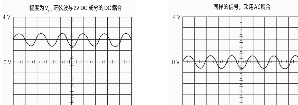
► 图23. AC 和DC 输入耦合
