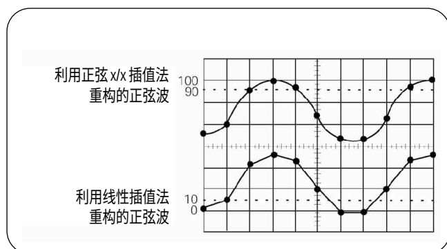
► 图31. 线性 and \sin x/x 插值法
