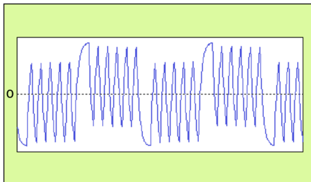
► 图 4.2.4a 带有数据相关抖动的数据信号
