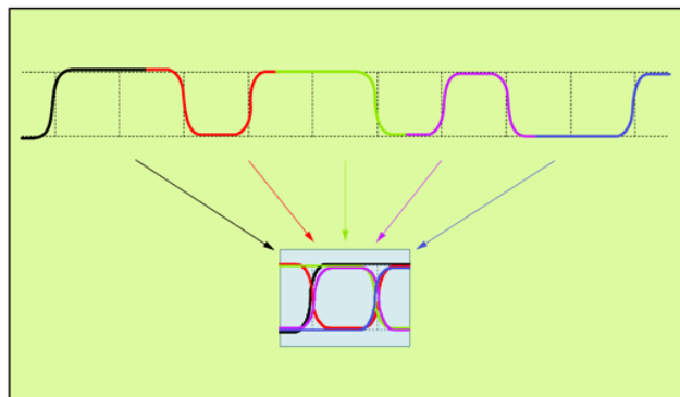
► 图 3.5a 建立实时眼图
