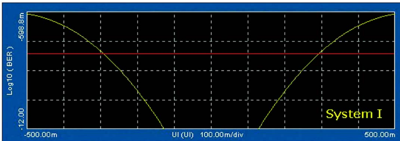
► 图 5.3a 随机性抖动为主的系统的 BER 曲线
