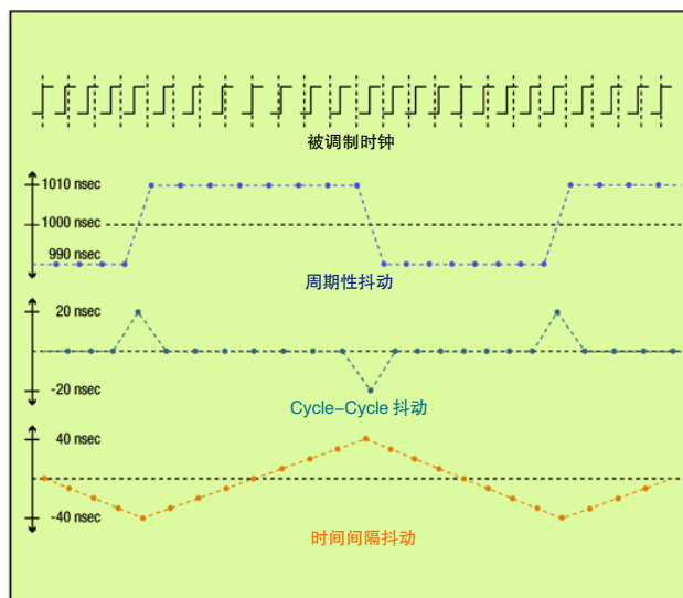
► 图 2.4c 不同测量的趋势图
