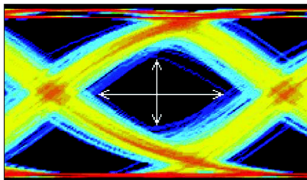
► 图 3.5b 带有颜色等级的波形数据库
