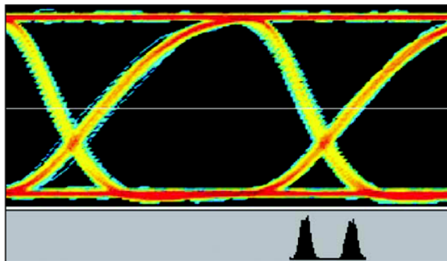
► 图 4.2.5a 不对称上升/下降时间导致的占空比失真
