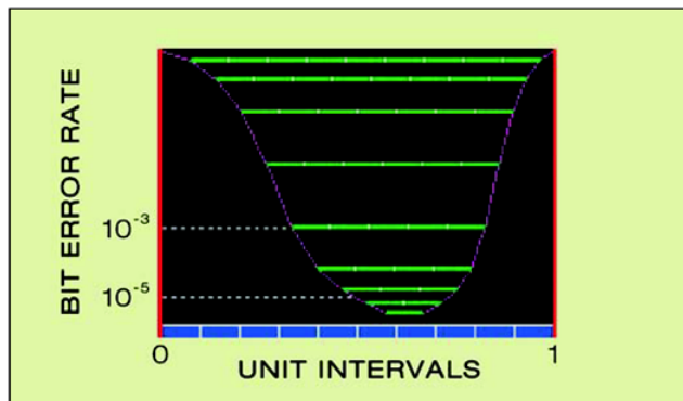
► 图 5.2b 测量眼宽随时间变化，确定误码率
