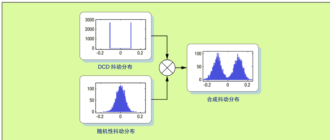
► 图 4.3a 使用确定性抖动对随机性抖动求卷积，找到总抖动
