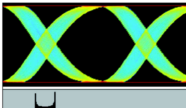
► 图 4.2.3b 非高斯抖动的眼图和直方图
