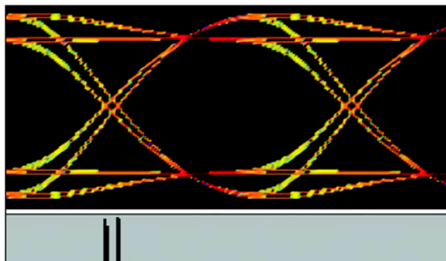
► 图 4.2.4c 数据相关抖动的眼图和直方图
