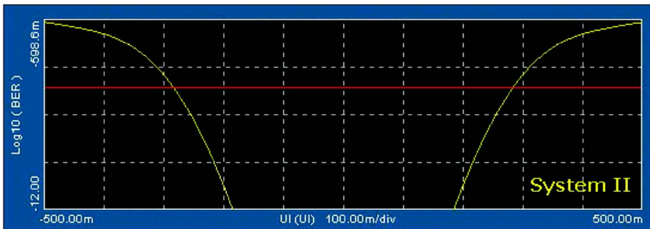
► 图 5.3b 确定性抖动为主的系统的 BER 曲线
