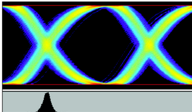
► 图 4.2.1b 高斯抖动的眼图和直方图
