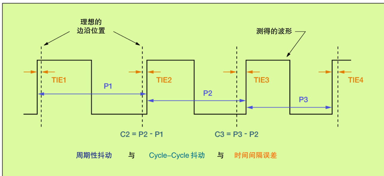
► 图 2.4a 不同的抖动测量项目
