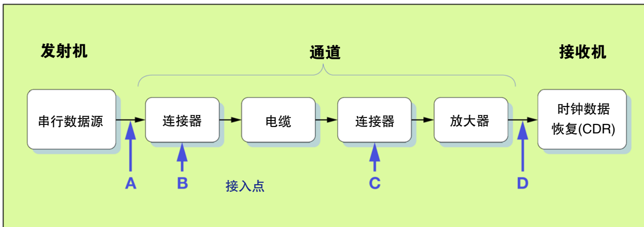
► 图 5.1 设置系统抖动预算的常用测量点
