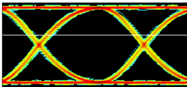
► 图 4.2.5b 不正确的检测门限导致的占空比失真
