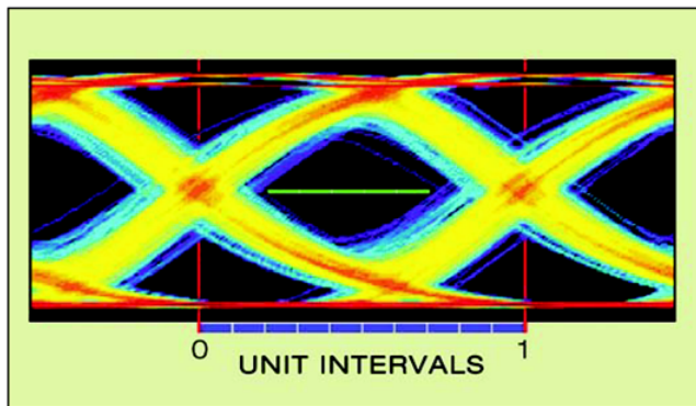
► 图 5.2a 眼宽用来确定性能
