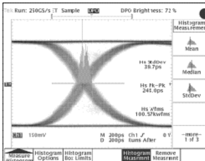
그림 11. 막대 그래프를 사용하여 디지털 비디오 신호의 무작위 지터를 특성화한다. 막대 그래프의 이항 모드 (bi-modal) 특성에 유의한다. 또한 막대 그래프의 속성은 화면 오른쪽에 나타나서 관련된 피크-피크 지터와 같은 특성을 나타낸다.
