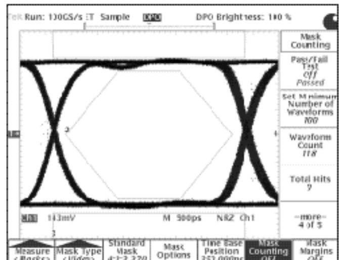
그림 12. 마스크 시험은 직렬 비디오 신호가 쉽게 표준을 준수하는지 여부를 확인하는 편리하고 신뢰성 있는 방법을 제공한다. 이 예에서, 최소 100 파형이 오류 없이 (0 "히트") 마스크와 비교되었다.
