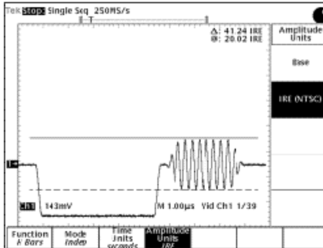
그림 8. NTSC 신호에서 전폭 측정의 예. 버스트 계정의 피크-피크 전폭은 격자나 비디오 커서를 사용하여 시간적으로 측정할 수 있다 (오른쪽 상단 모서리에 커서 좌표값을 기록한다).
