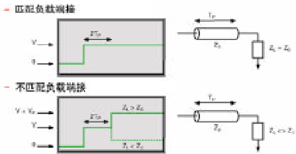
► 图 5: 匹配的和不对应的负载端接
