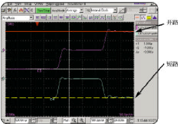
► 图 2：时域测量显示了一个开路和短路的阶跃。短路测量结果为 -1 r(\rho) ，开路(无穷大欧姆)测量结果为 r = +1_0 。
