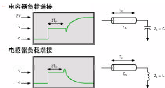
► 图 6: 电容和电感负载端接
