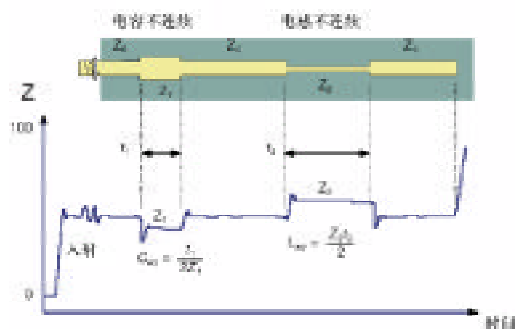
► 图 9: TDR 波形揭露了轨迹不连续点
