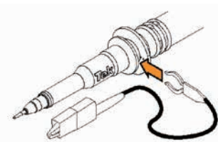
ワニ口グラウンド・リード (15cm) 196-3521-01
