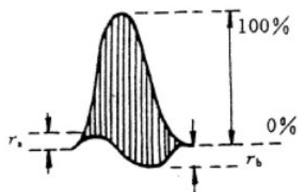
图 2.28 失真的复合 2Tc 脉冲
