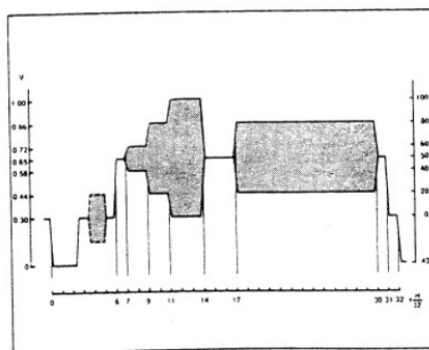
图 2.31 第 18 行插测信号
