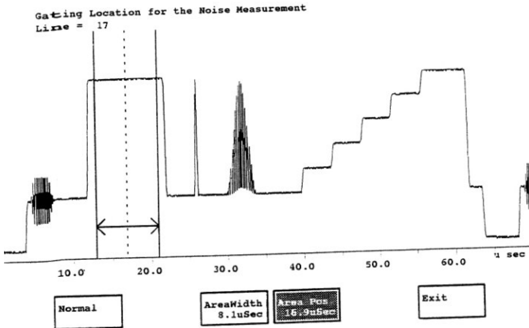
图 6.13 噪声谱输入选通显示
