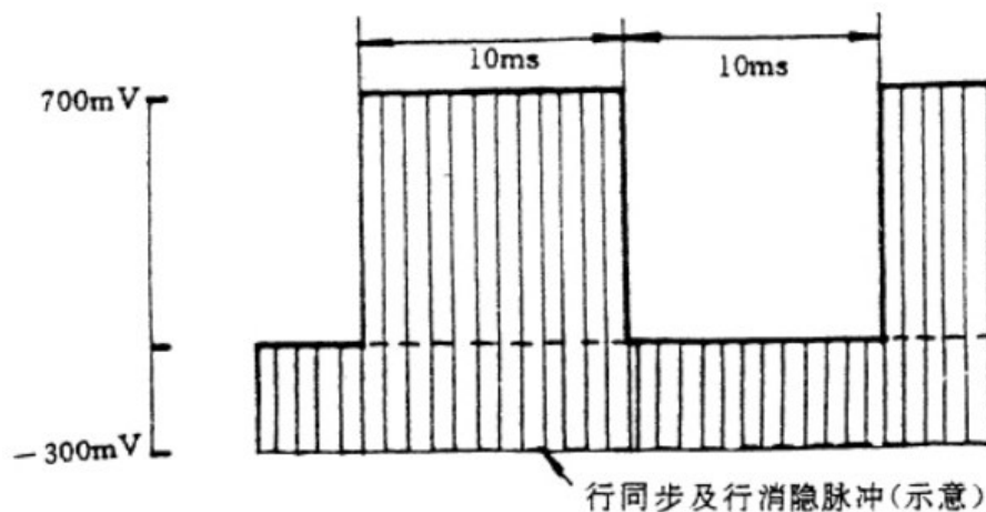
图 2.15 场方波信号
