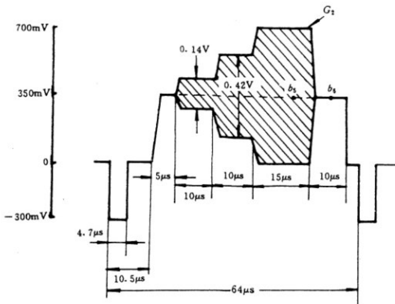
(b) 三电平色度信号 G2
