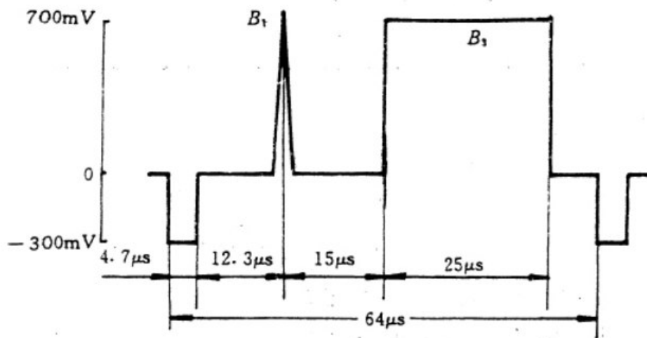
图 2.17 2T 正弦平方脉冲和条脉冲信号 B1、B3
