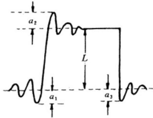
图 2.22 过冲式中波形
