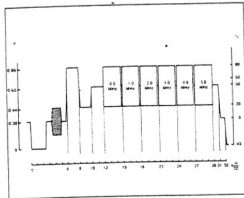
图 2.33 第 331 行插测信号
