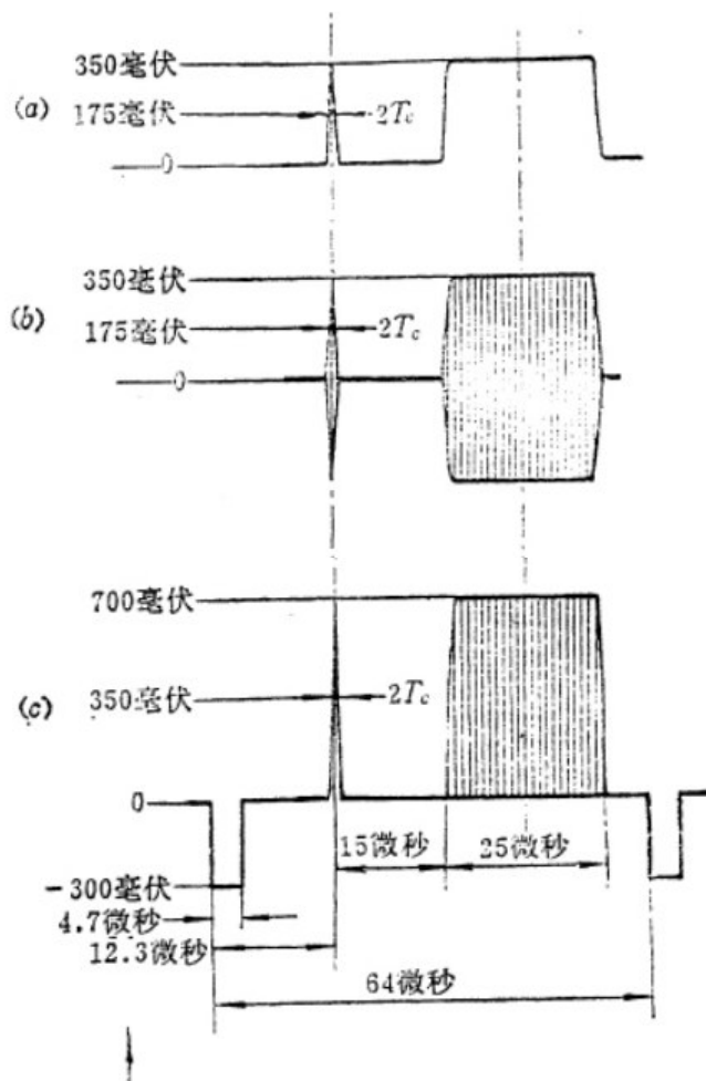
图 2.27 (a) 2Tc 正弦平方脉冲和条信号 (b) 由(a)信号调制的彩色负载波 (c) 信号(a)+信号(b)
