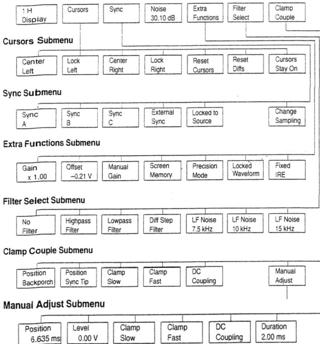
图 3.1 波形(Waveform)方式下软按键菜单(Menu)一览表
