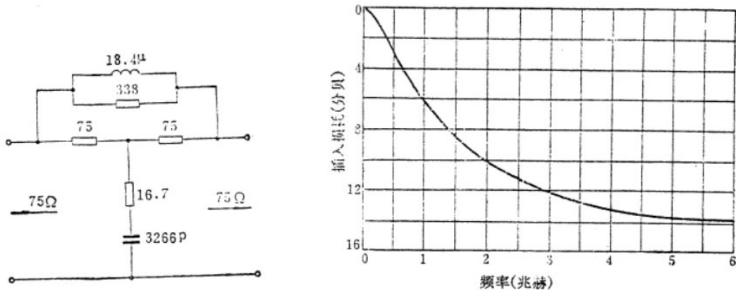
图 2.29 (a) 统一的加权网络 (b) 统一加权网络的幅频特性
