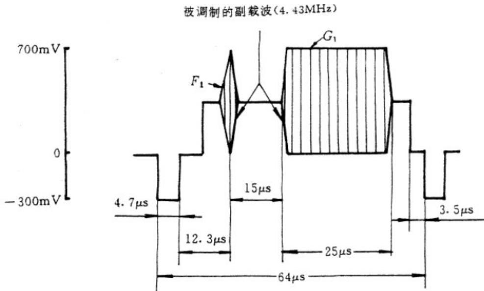
图 2.5(a) 10T 和条脉冲调制的负载波信号 F1、G1
