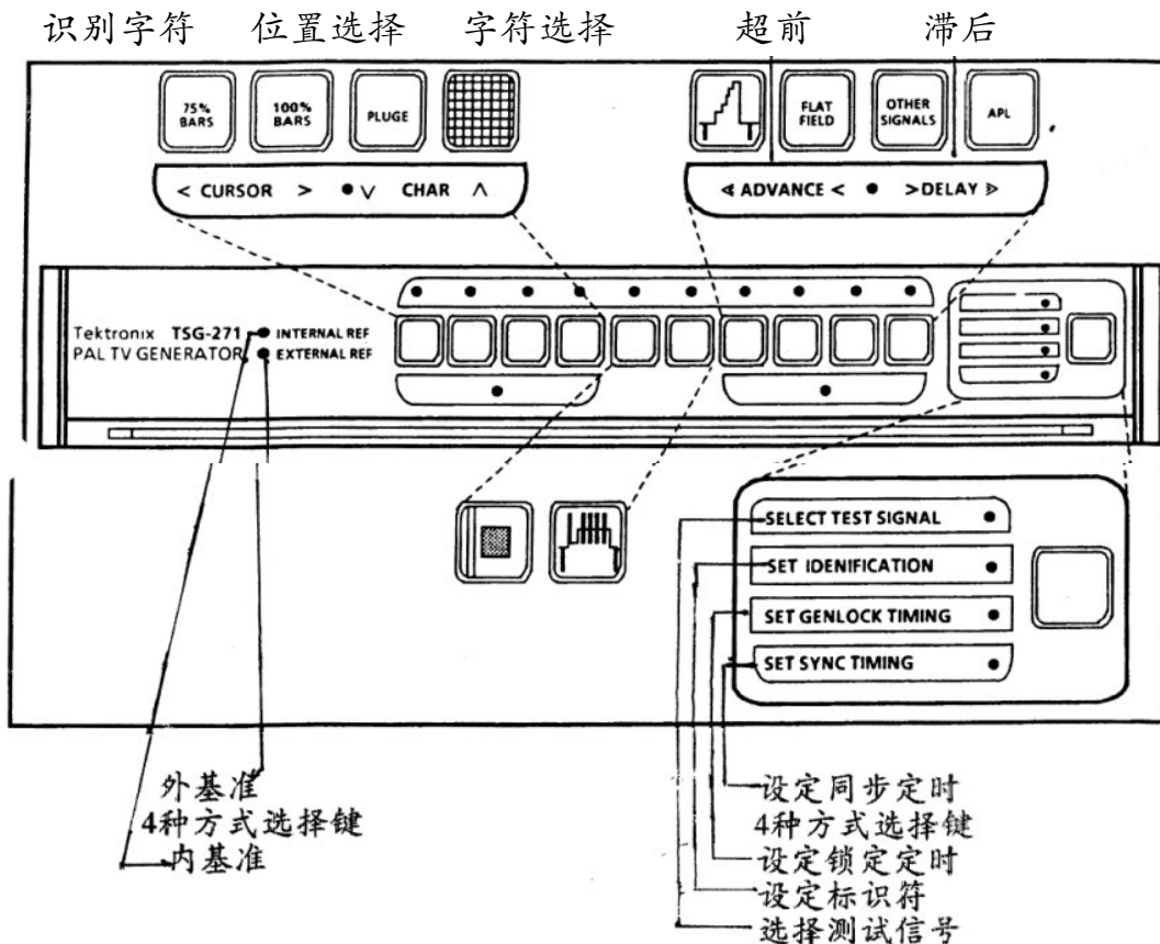
图 B.1 TSG-271 前面板
