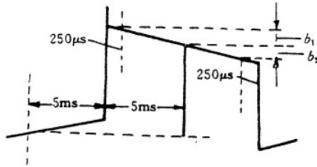
图 2.16 场时间波形失真
