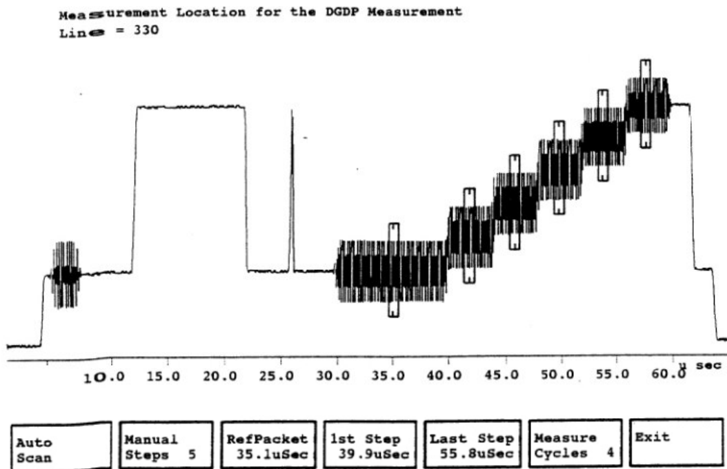
图 6.8 DG DP 测试信号及测试位置
