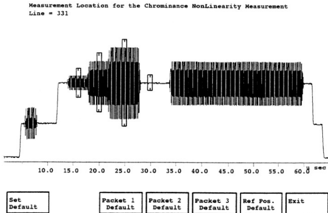
图 6.6 色度非线性测试信号及子菜单
