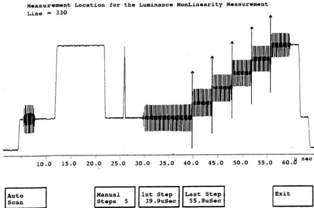
图 6.11 亮度非线性测试波形及测量位置
