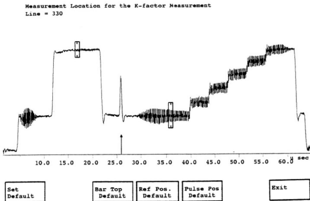
图 6.10 K 系数测试波形及测量位置
