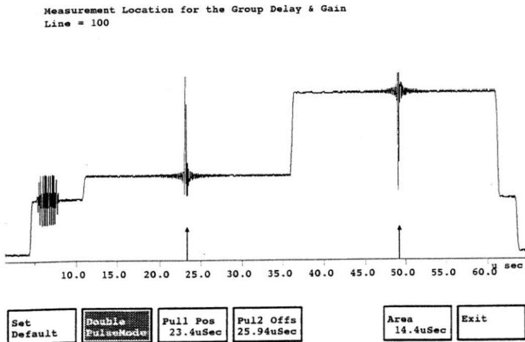
图 6.9 Group Delay~Sinx-x 测试信号及测试位置
