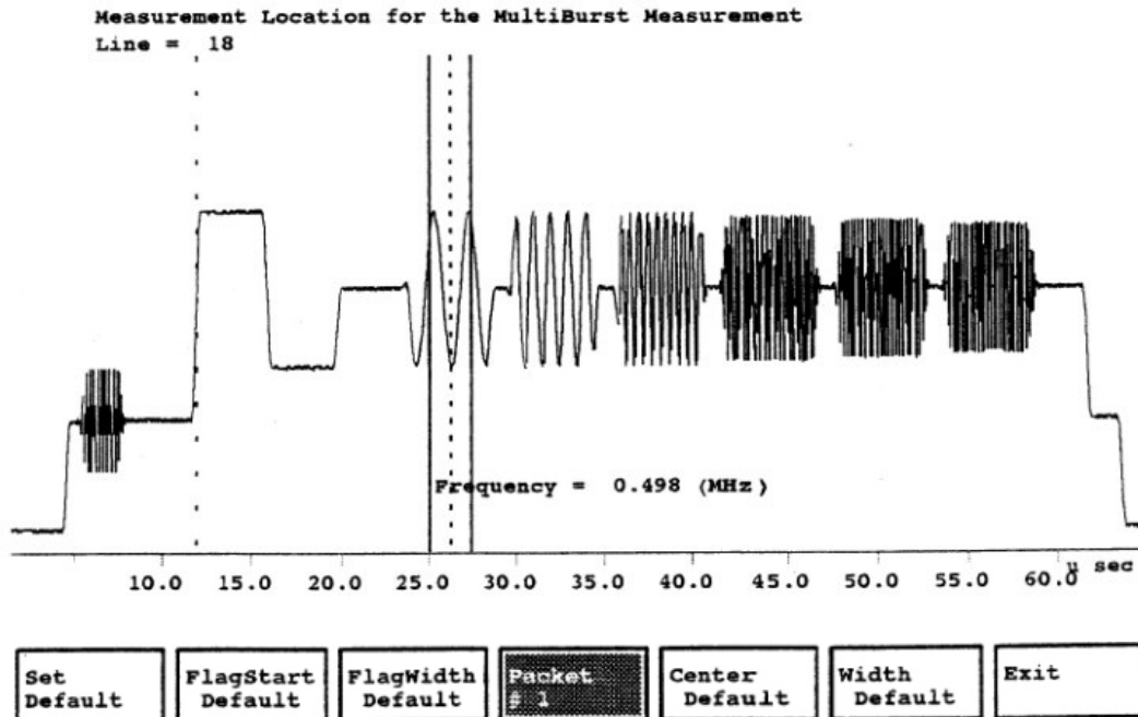
图 6.12 多波群测试信号及测量位置
