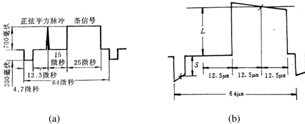
图 2.9 (a)同步信号非线性失真的测试信号 (b)同步信号的非线性失真
