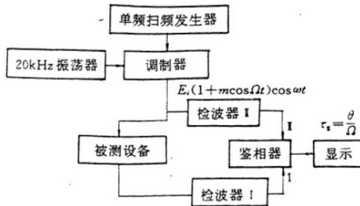
图 2.13 调幅法测群时延失真
