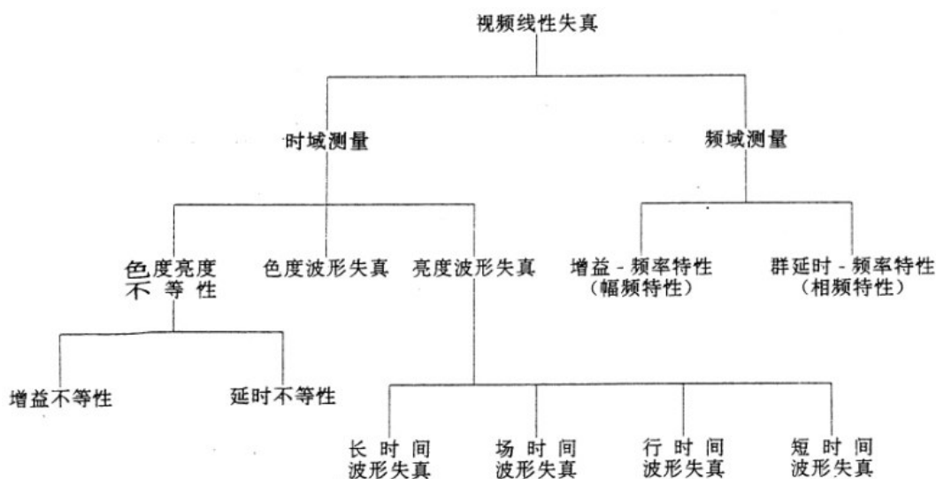
图 2.11 视频线性失真分类
