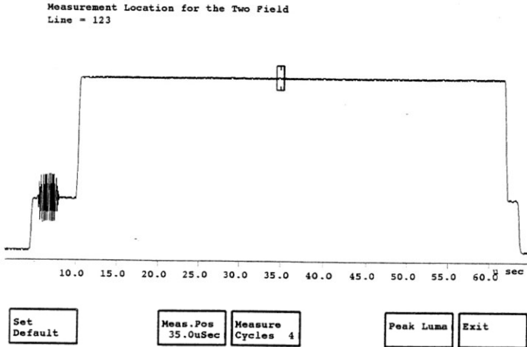
图 6.14 Two Field 测试信号及测量位置
