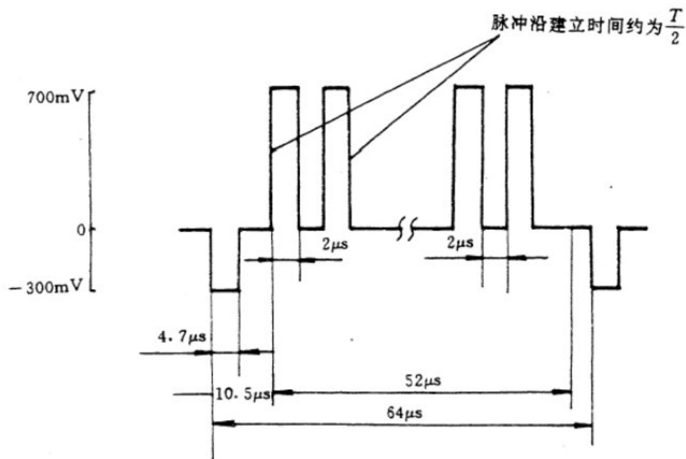
图 2.21 250KHz 方波信号
