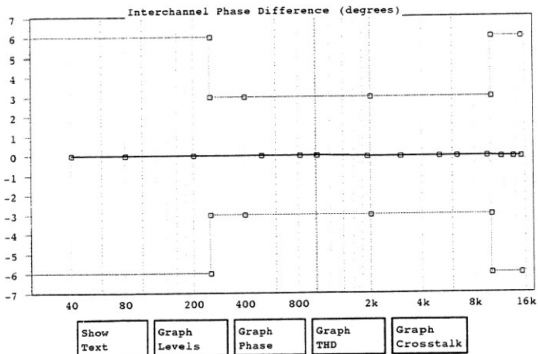
图 9.3 音频自动测试的图形显示
