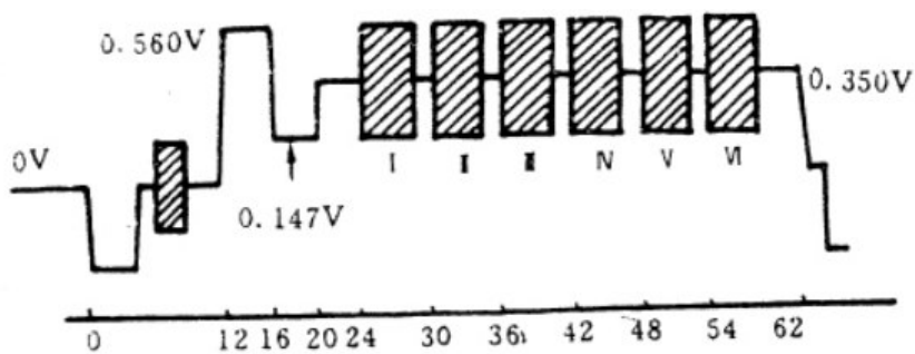
图 2.35 第 20 行插测信号
