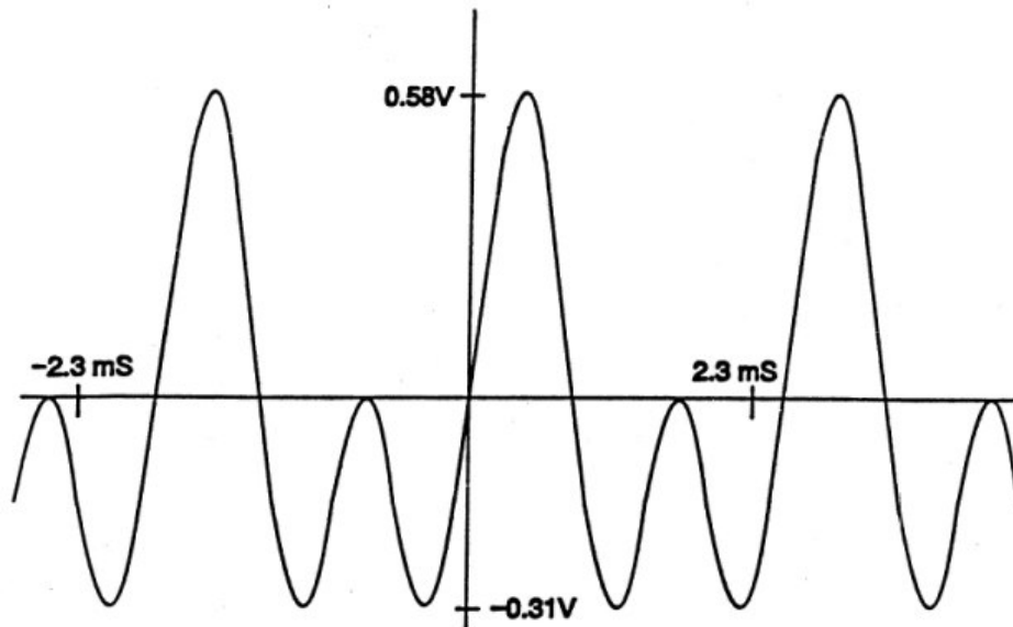
图 A.4 极性信号
