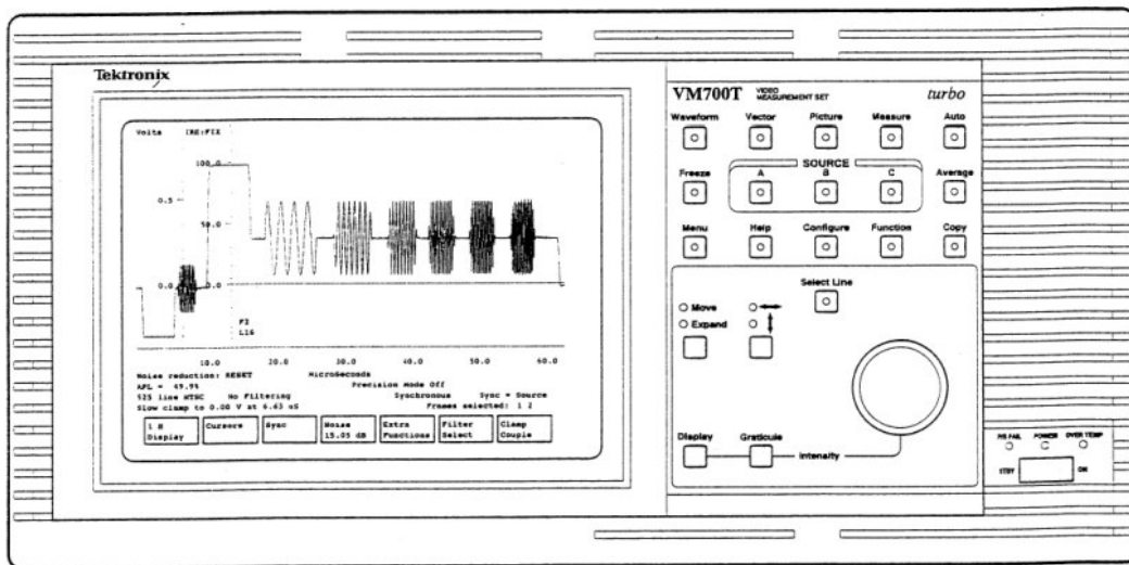
图 1.1 VM700 的前面板
