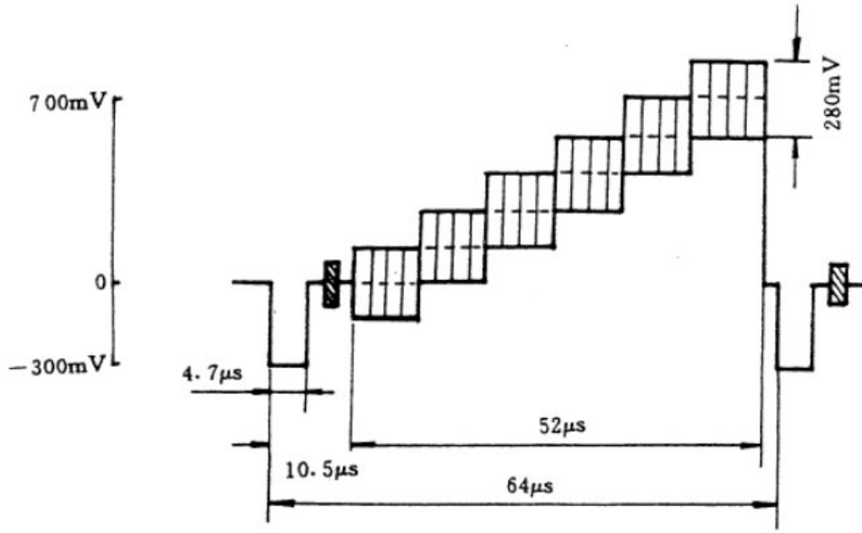
图 2.7 五阶梯叠加 4.43MHz 信号
