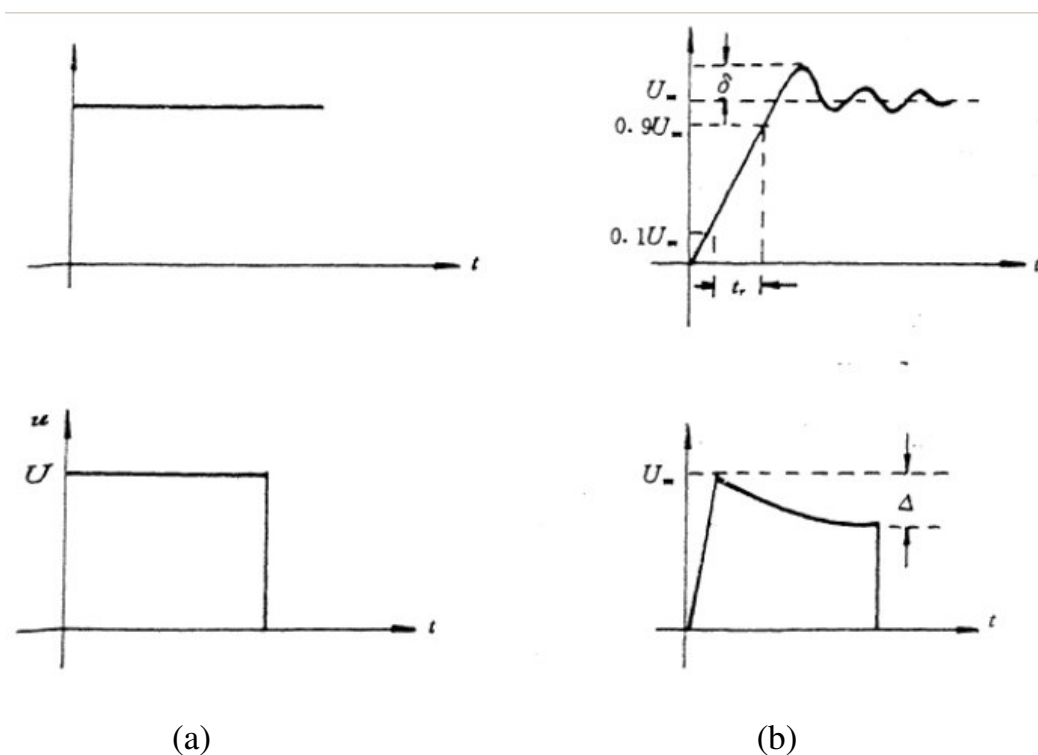
图 2.10 用方波瞬态响应
