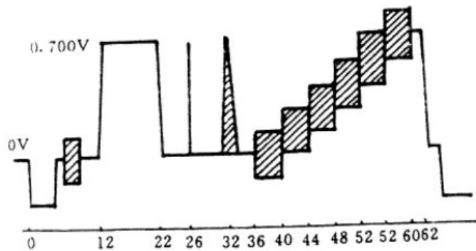
图 2.34 第 19 行插测信号
