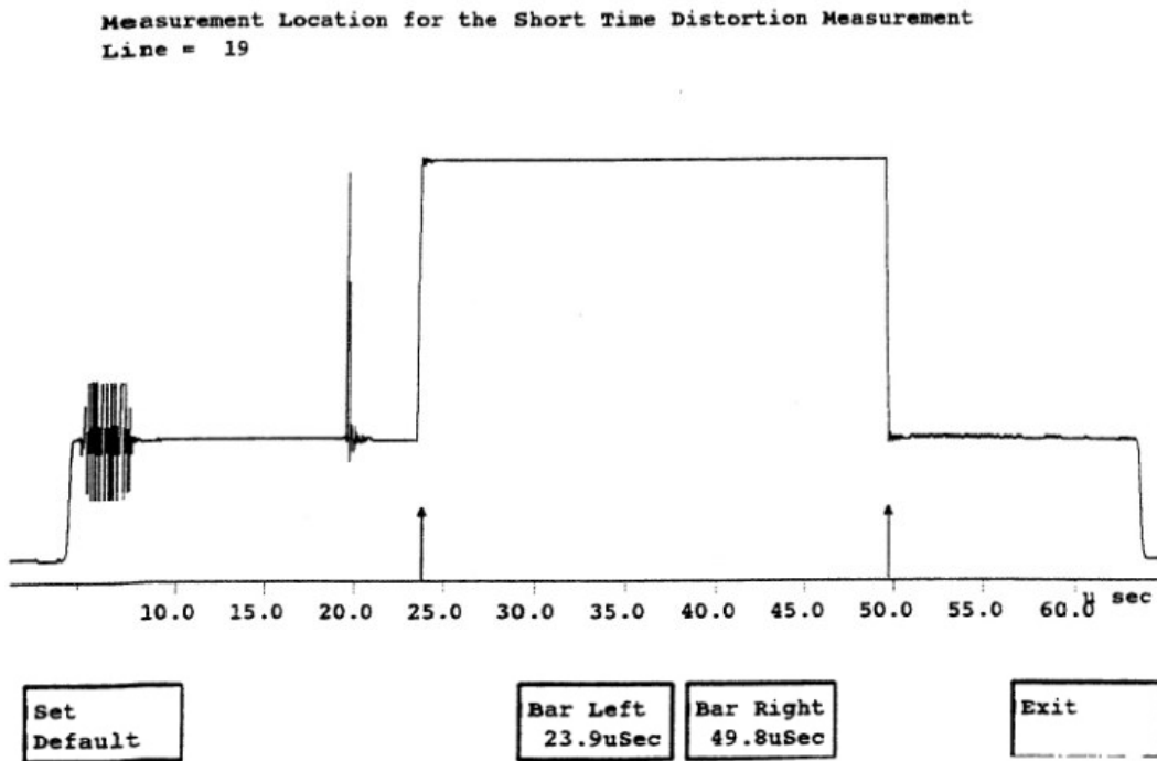
图 6.13 短实际失真测试波形及测量位置
