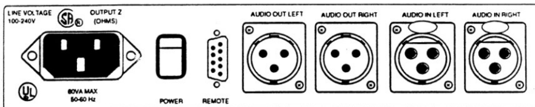
图 A.2 ASG100 的后面板
