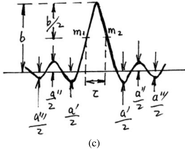
图 2.26 (a) 2T 脉冲信号 (b) K_p 容限图 (c) 2T 脉冲失真波形
