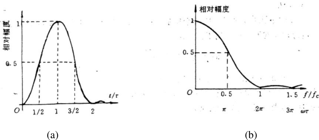
图 2.19 (a) 正弦平方脉冲波形 (b) 正弦平方脉冲的频谱
