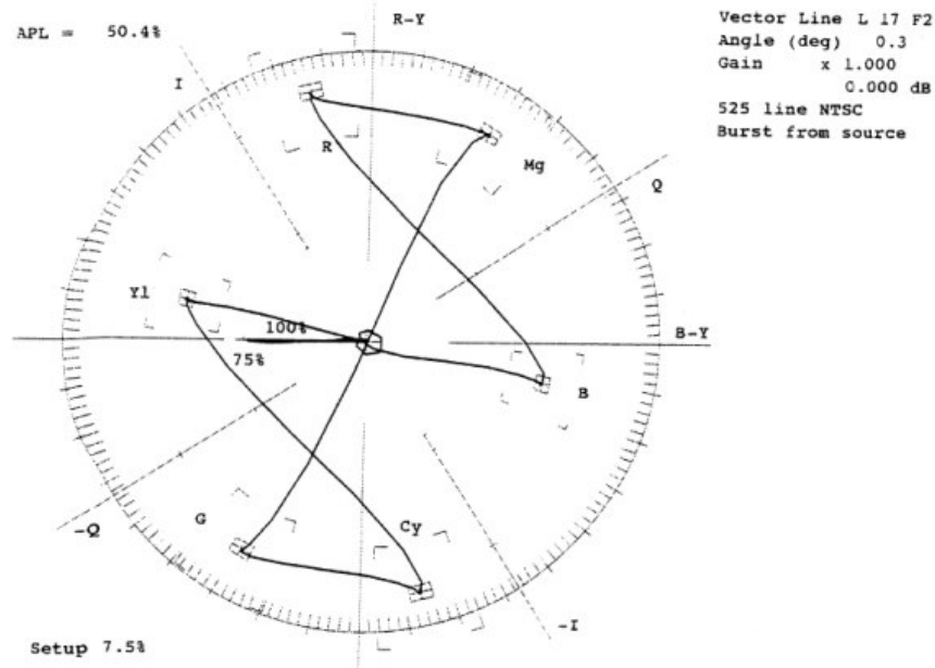
图 4.1 标准彩条信号的向量表示
