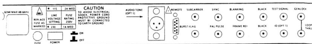
图 B.2 TSG-271 后面板
