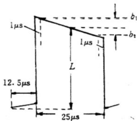
图 2.18 行时间波形失真
