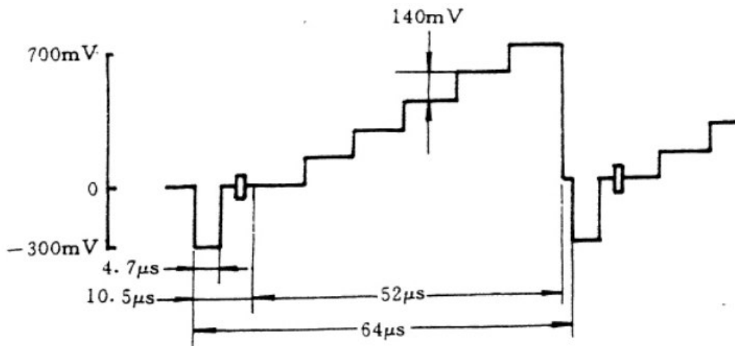
图 2.3 (a) 五阶梯波
