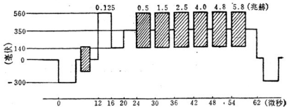
图 2.12 多波群信号
