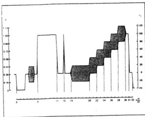
图 2.30 第 17 行插测信号
