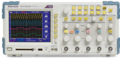
幅: 336mm 高さ: 161mm 奥行: 130mm 質量: 約3.2kg (バッテリー1個を含む)
