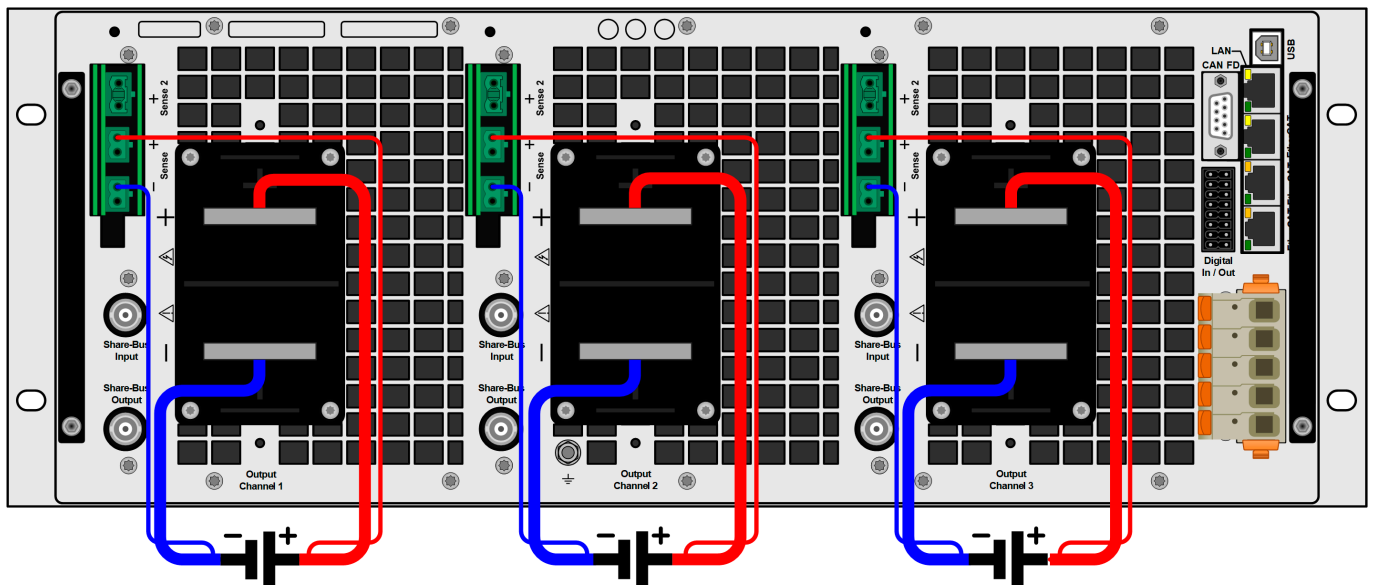
Figure 15 - Exemple de câblage Sense d'une batterie sur chaque canal (capuchons masqués à des fins d'illustration)
