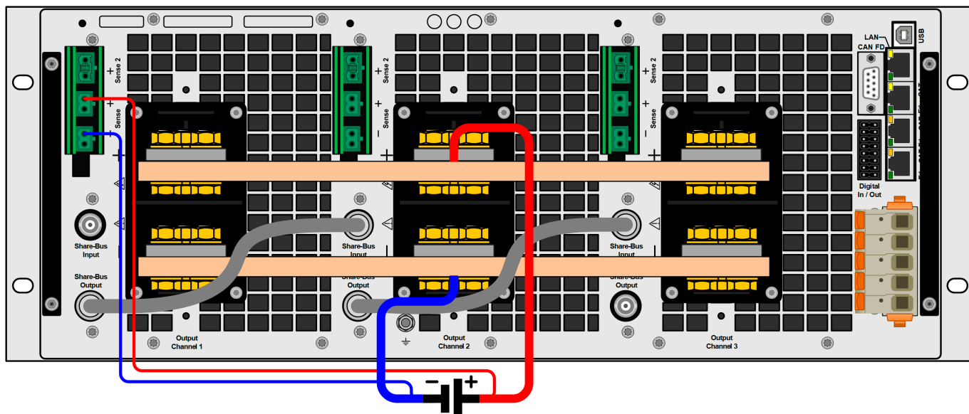
Figure 16 - Exemple de câblage Sense d'une charge en mode groupement de canaux (capuchons masqués à des fins d'illustration)
