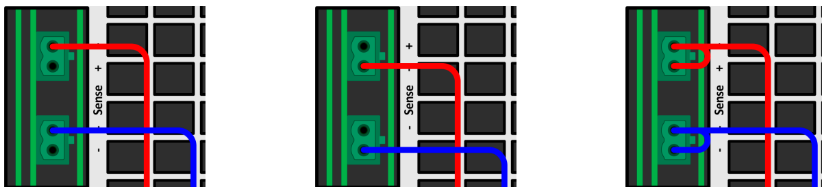
Figure 15 - Exemple de câblage Sense d'une batterie sur chaque canal (capuchons masqués à des fins d'illustration)
