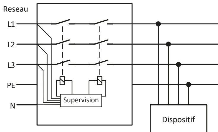
Figure 9 - Principe d'un réseau de protection RI
