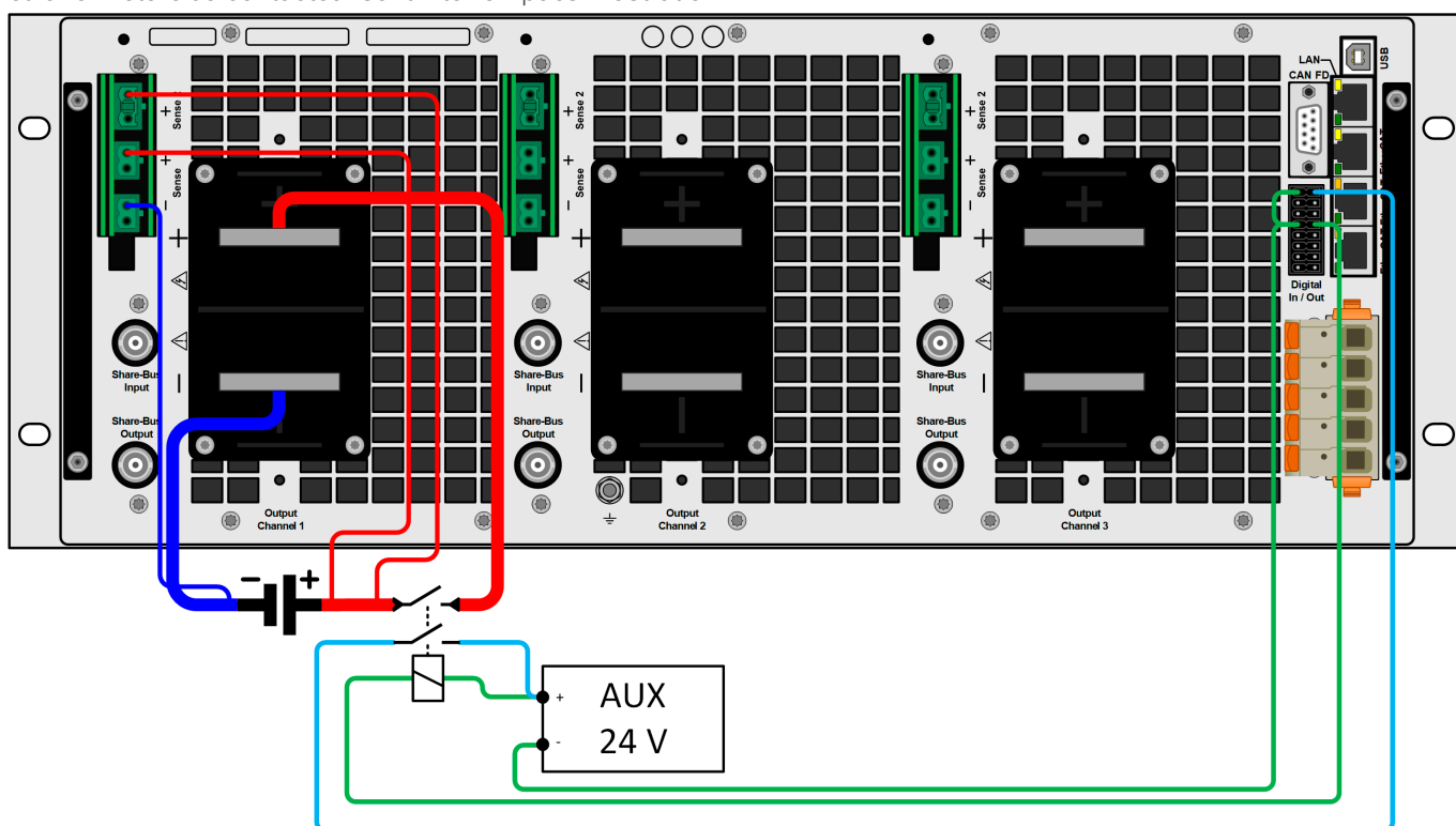
Figure 17 - Exemple de câblage d'une batterie sur le canal 1, avec détection de la polarité, précharge et commande des contacteurs (Digital In / Out-Port)
