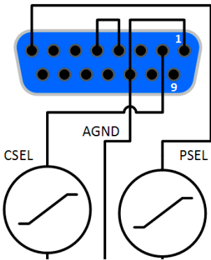
利用外部电压源的范例
