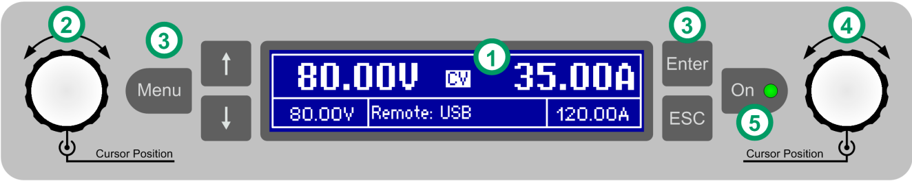
图 6 – 控制面板
