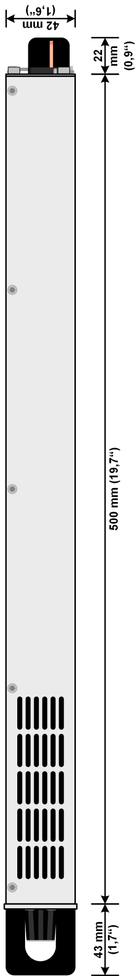
图 4 - 右侧视图 (带直流端子盖)
