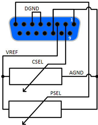
利用电位器的范例
