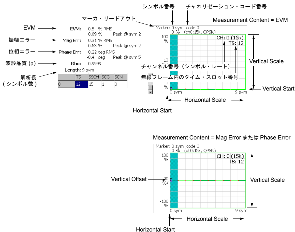
図 2-19 : シンボル EVM
