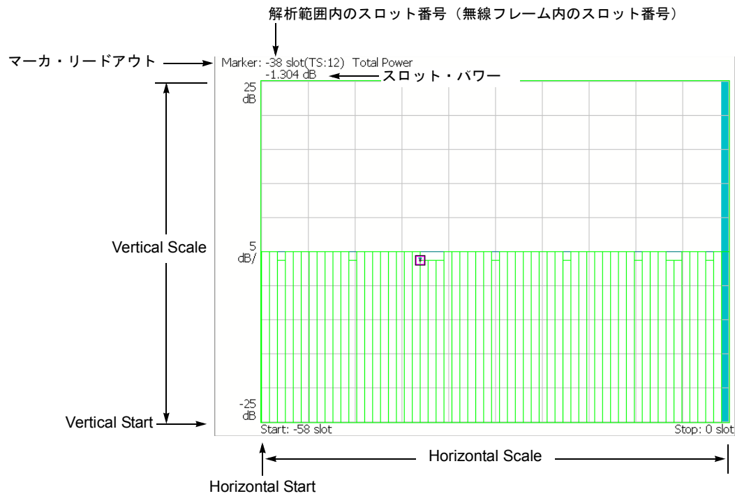
図 2-32 : コード・ドメイン・パワー vs タイム・スロット
