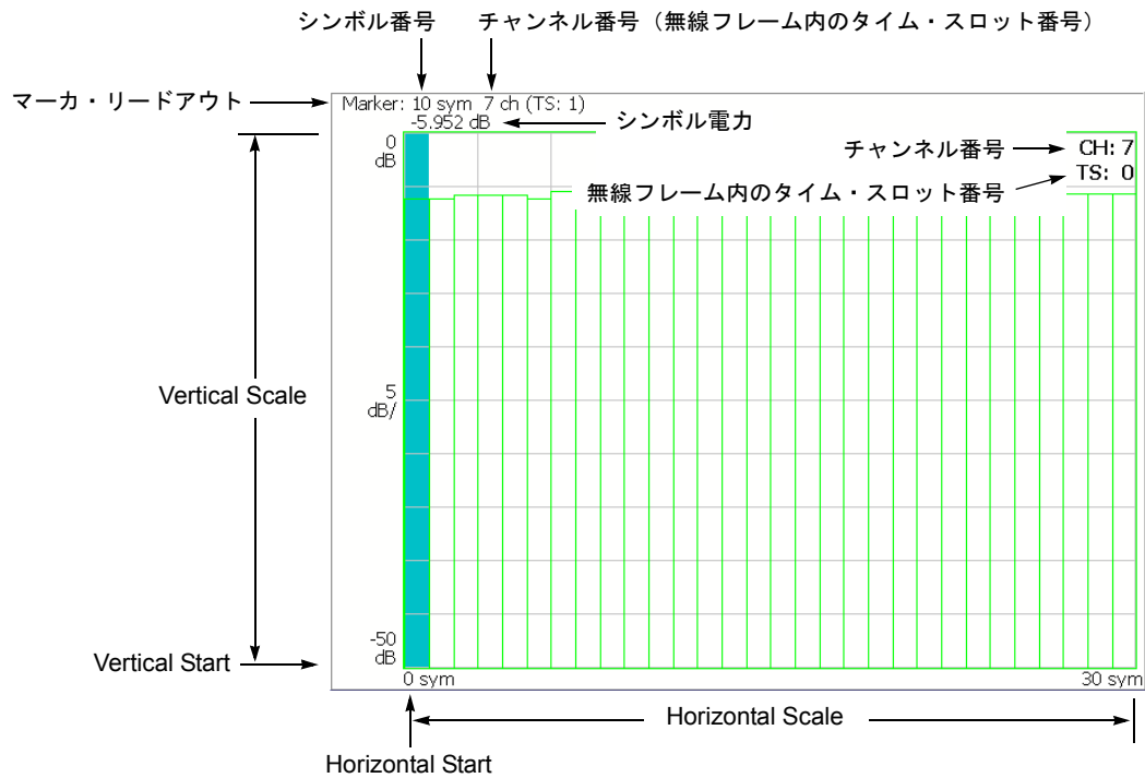
図 2-33 : コード・ドメイン・パワー vs シンボル
