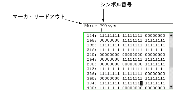
図 2-37 : シンボル・テーブル
