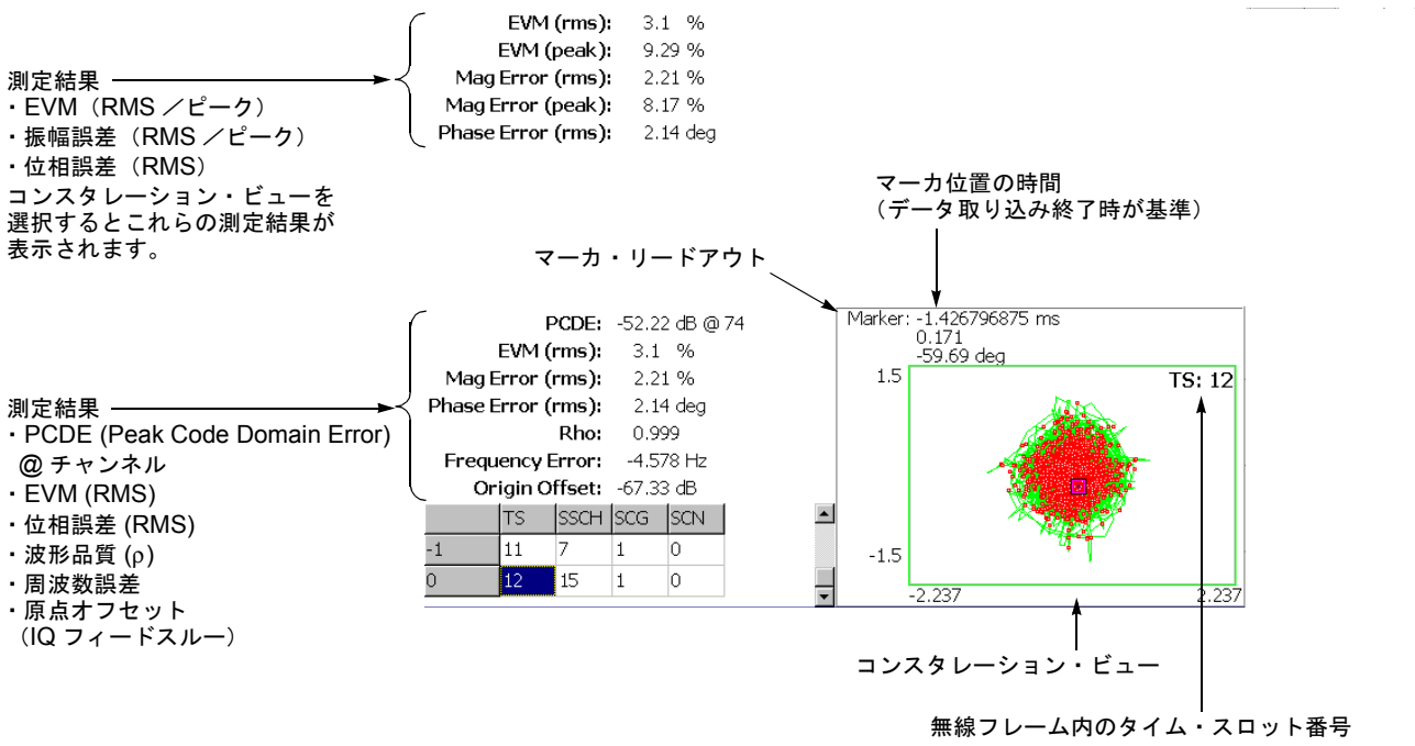
図 2-22 : 変調確度
