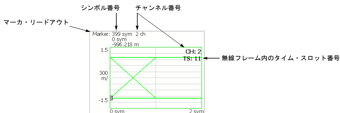
図 2-36 : シンボル・アイ・ダイアグラム
