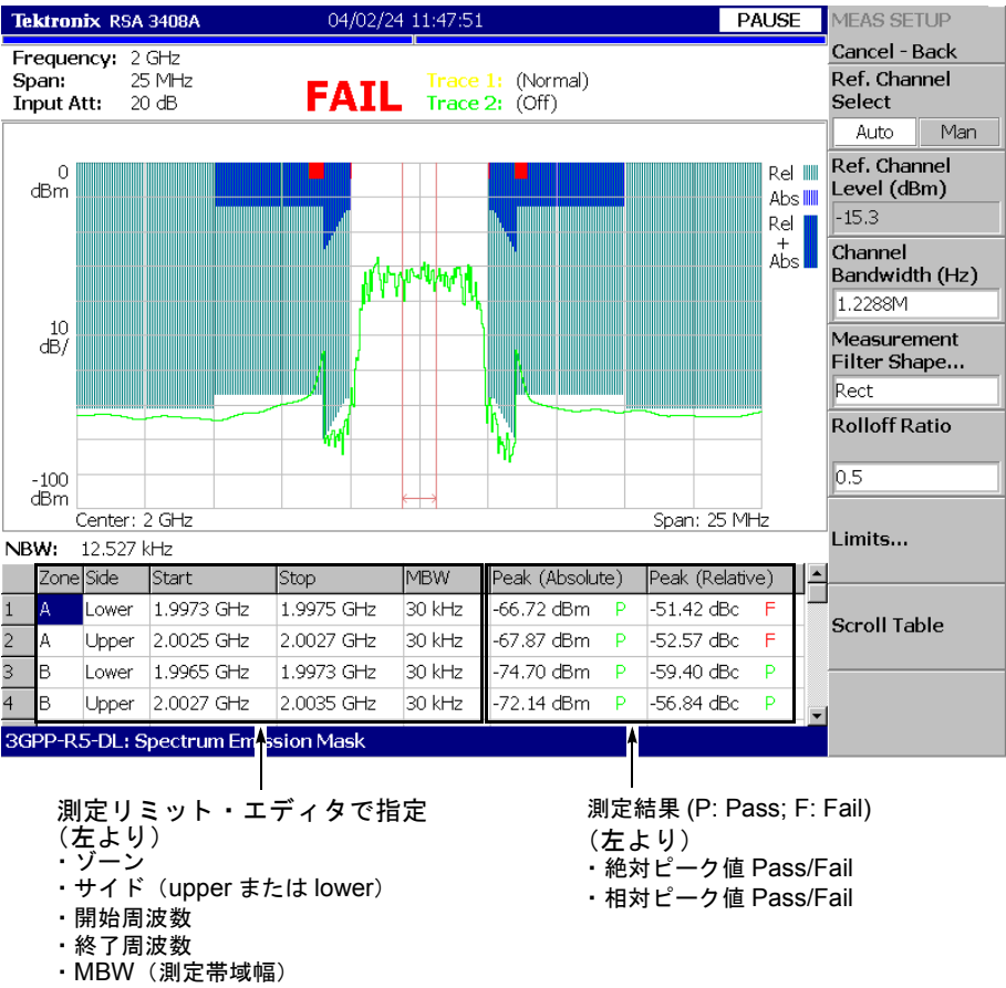
図 2-5 : スペクトラム放射マスク測定
