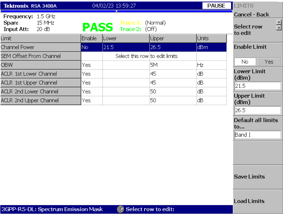
図 2-9 : 測定リミット・エディタ
