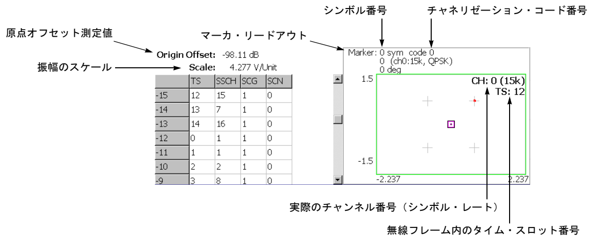
図 2-18 : シンボル・コンスタレーション
