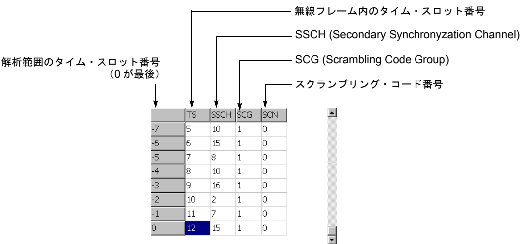
図 2-13 : タイム・スロット・テーブル
