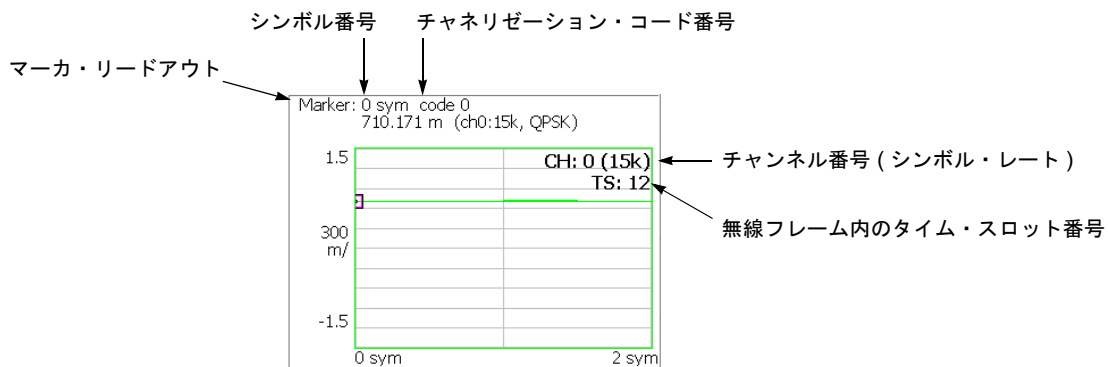
図 2-20 : シンボル・アイ・ダイアグラム
