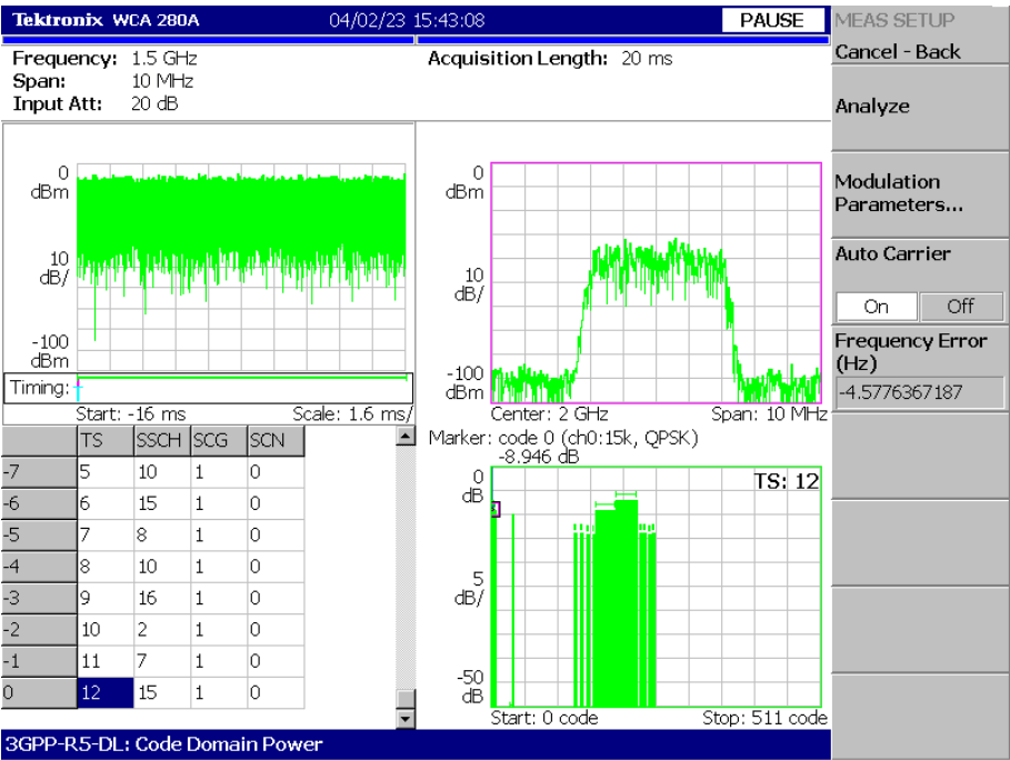
図 2-12 : コード・ドメイン・パワー測定例
