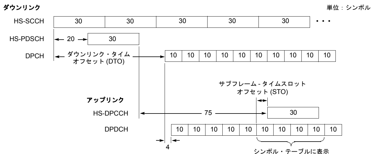
図 2-25 : サブフレーム・オフセット
