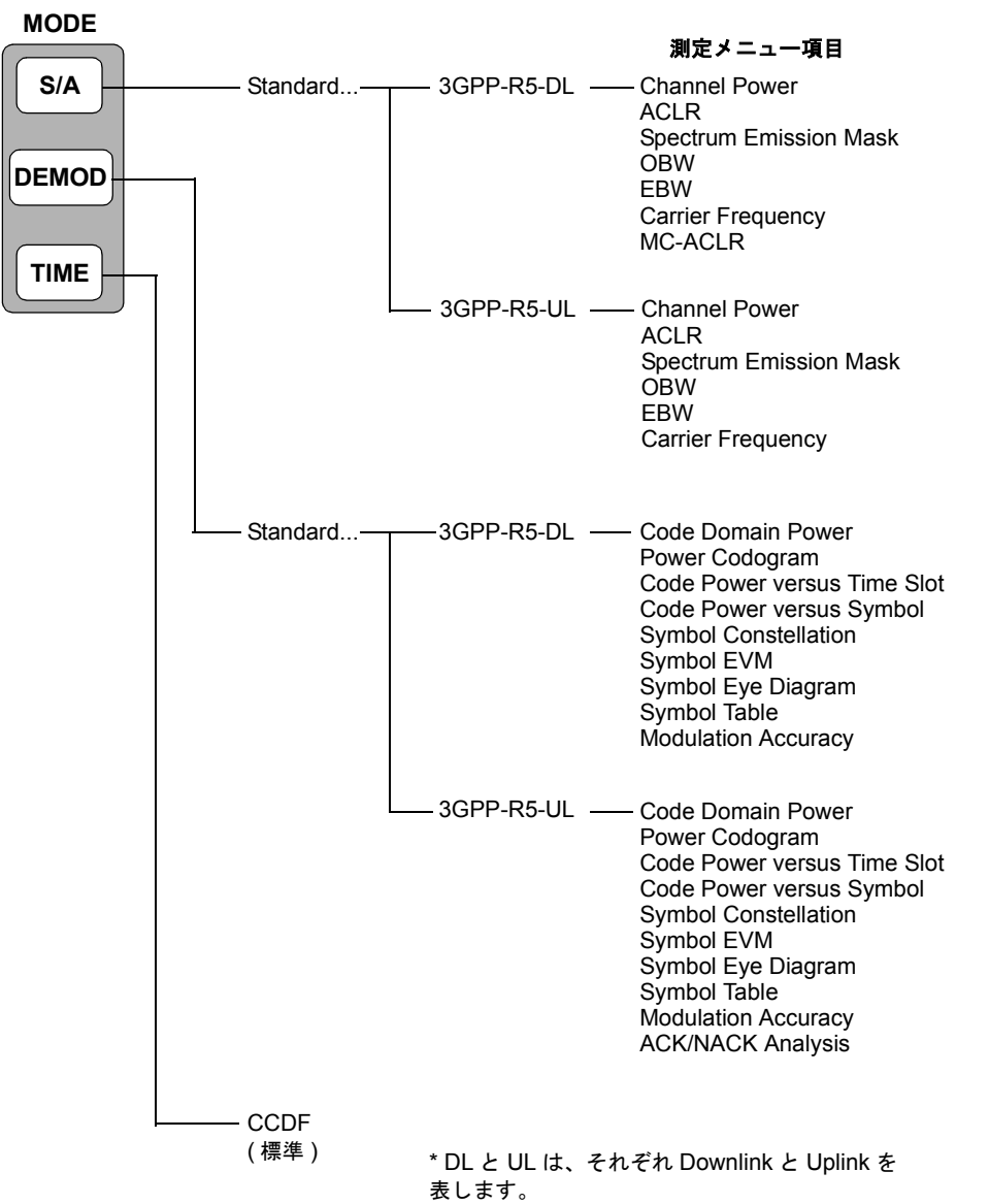
図 1-1 : 3GPP-R5 解析の測定メニュー
