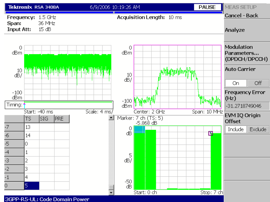
図 2-24 : コード・ドメイン・パワー測定例
