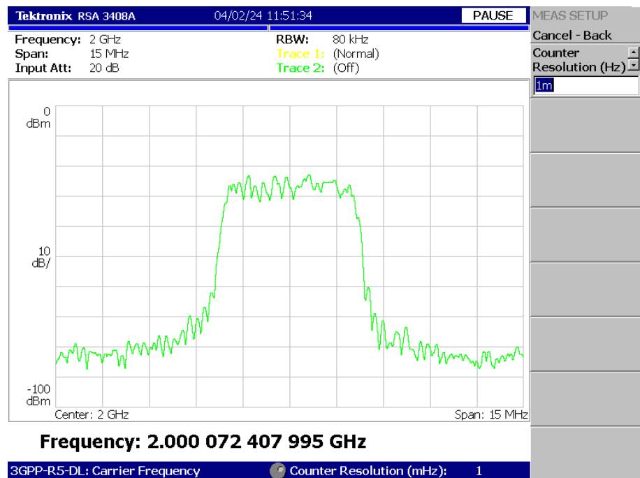
図 2-8：キャリア周波数測定
