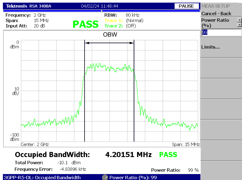
図 2-6 : OBW 測定
