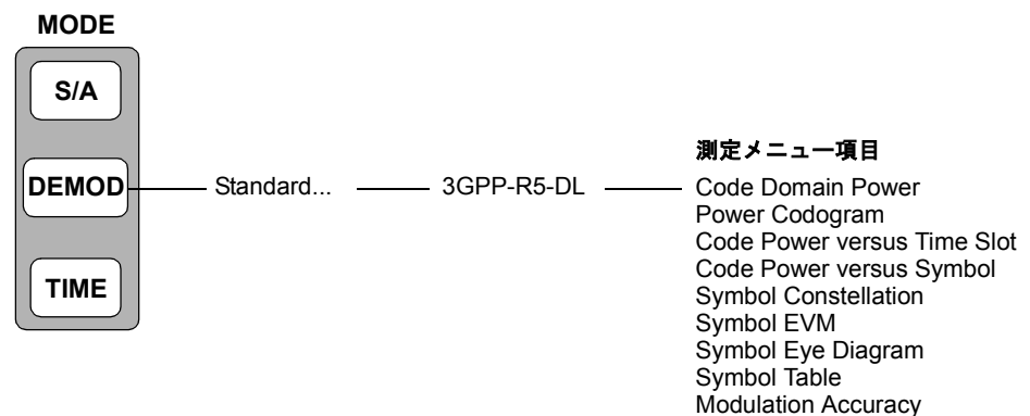
図 2-11 : ダウンリンク変調解析メニュー
