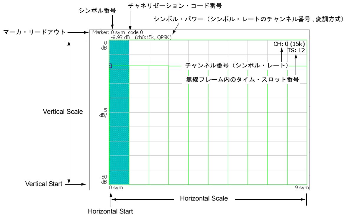
図 2-17 : コード・ドメイン・パワー vs シンボル
