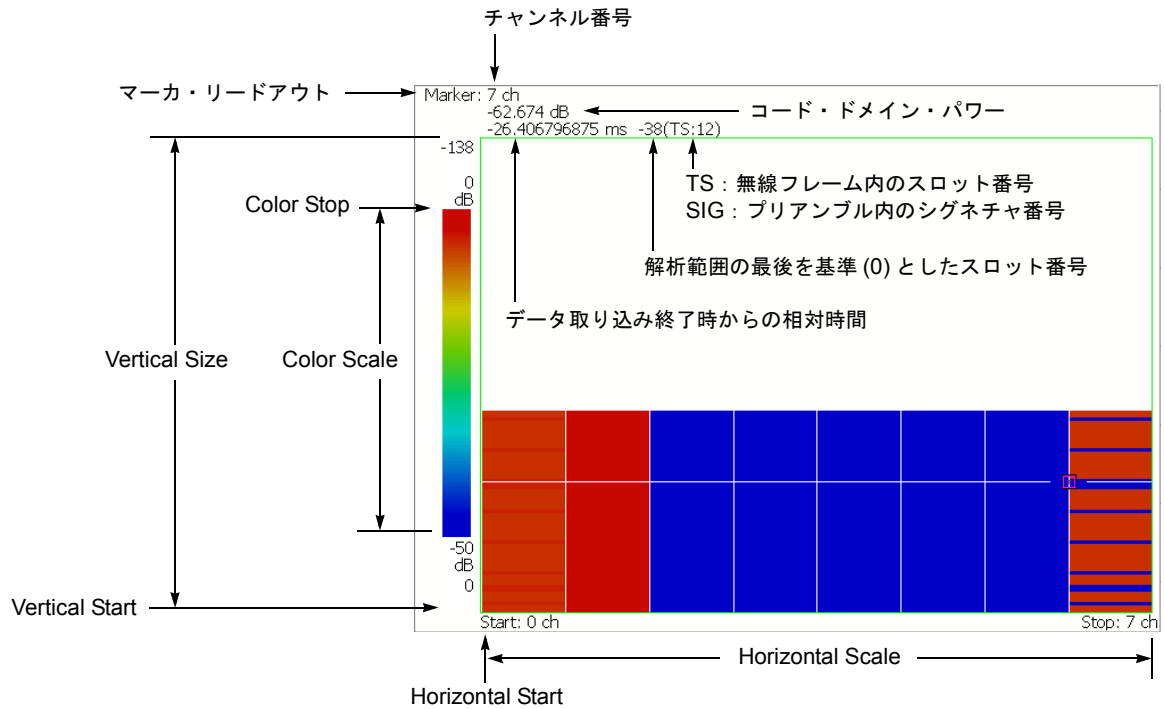
図 2-31 : パワー・コードグラム
