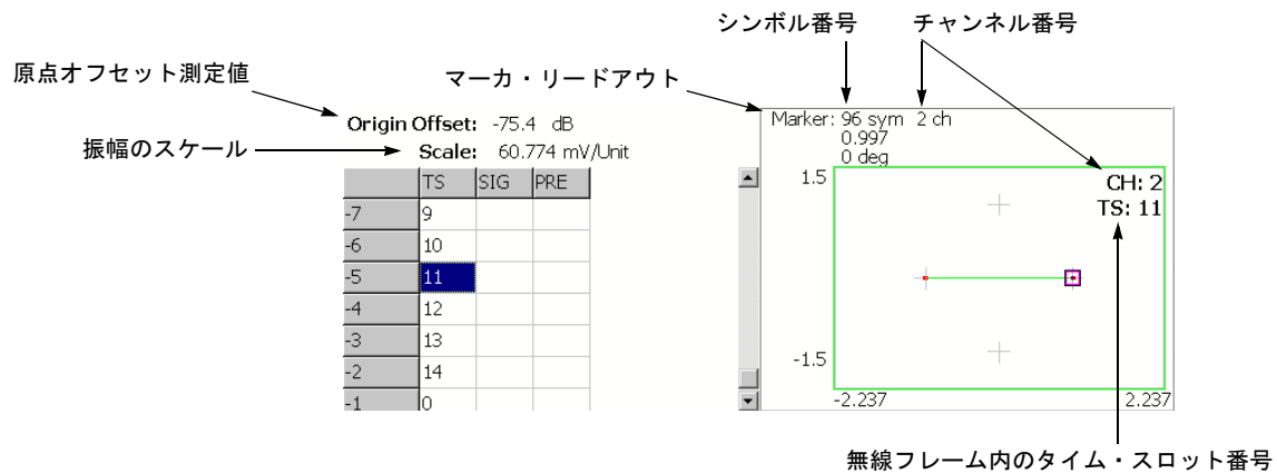
図 2-34 : シンボル・コンスタレーション
