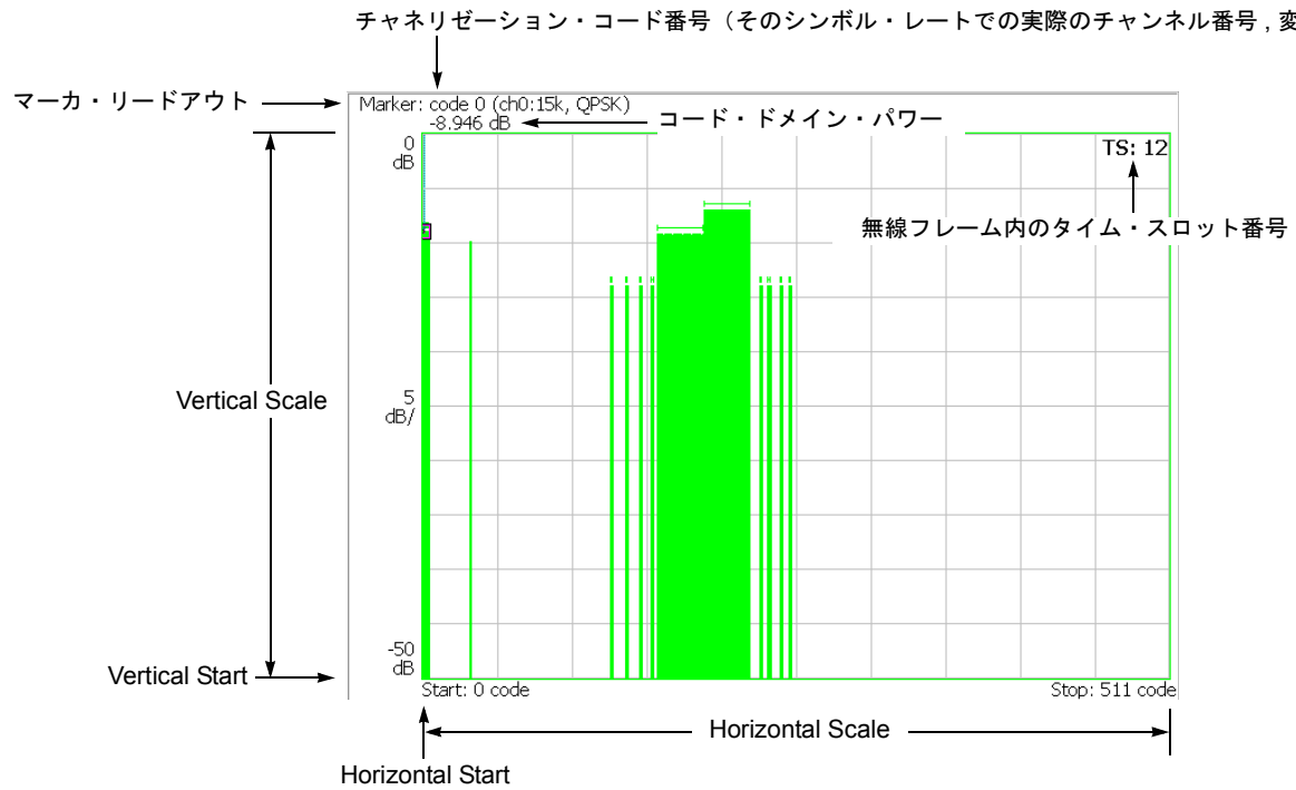
図 2-14 : コード・ドメイン・パワー
