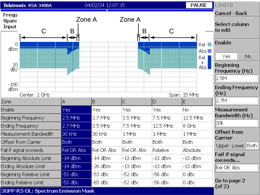
図 2-10 : スペクトラム放射マスク測定用リミット・エディタ
