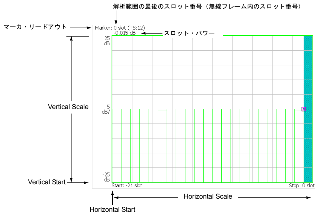
図 2-16 : コード・ドメイン・パワー vs タイム・スロット
