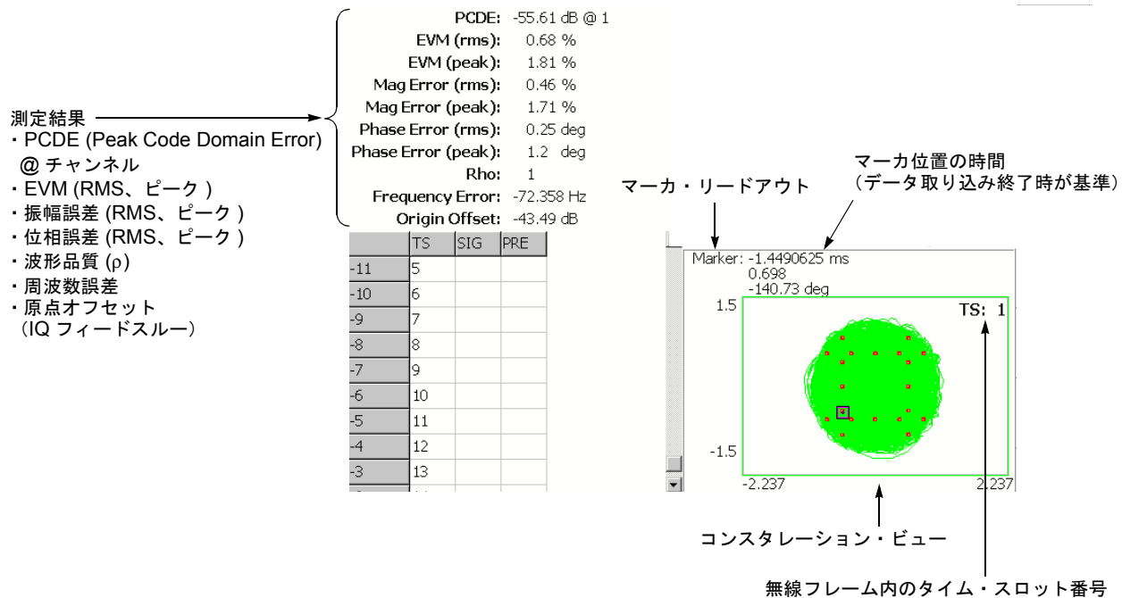
図 2-38 : 変調確度
