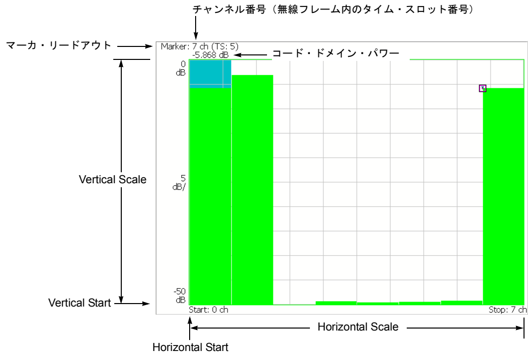
図 2-30 : コード・ドメイン・パワー
