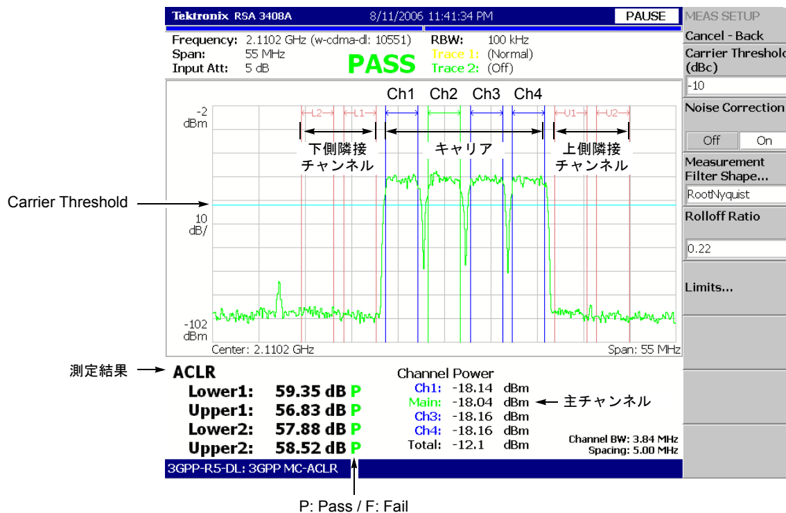
図 2-4 : 3GPP-R5 マルチキャリア ACLR 測定
