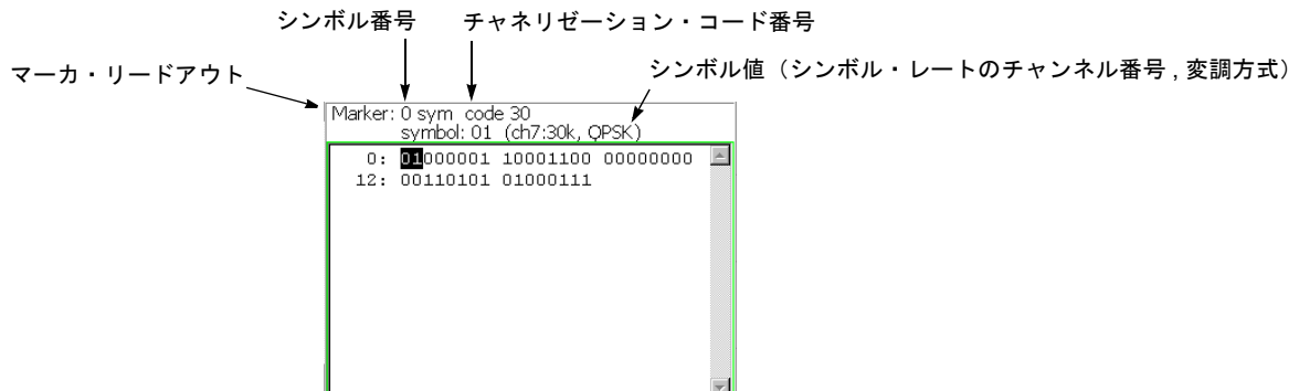
図 2-21 : シンボル・テーブル
