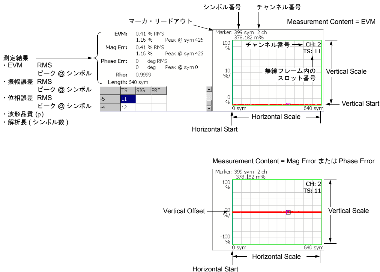
図 2-35 : シンボル EVM
