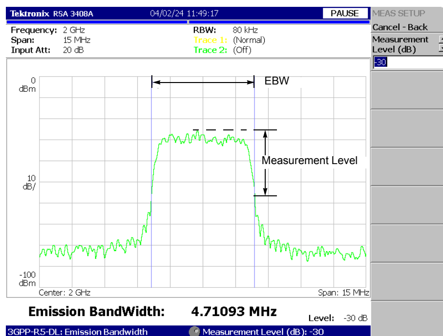
図 2-7 : EBW 測定
