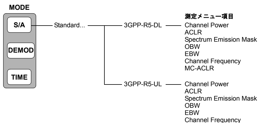
図 2-1 : S/A モードの解析測定メニュー
