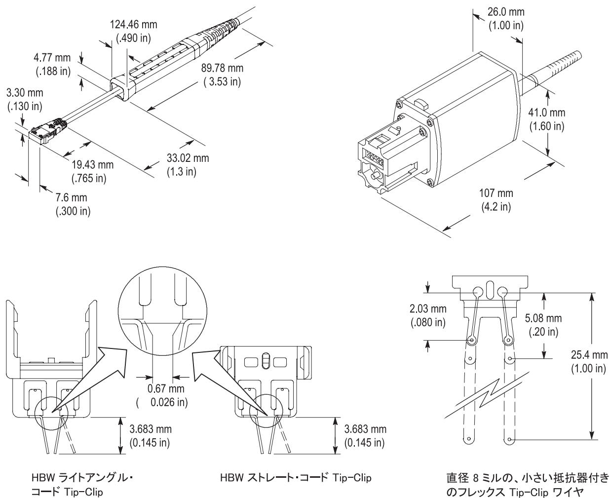
図 6 : プローブと Tip-Clip の寸法
