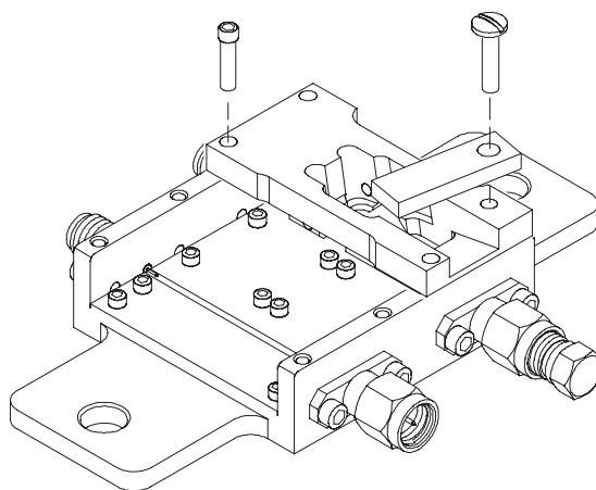
図 8 : プローブ校正アダプタ
