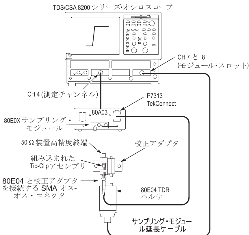
図 17: テスト・プローブの立上り時間の設定
