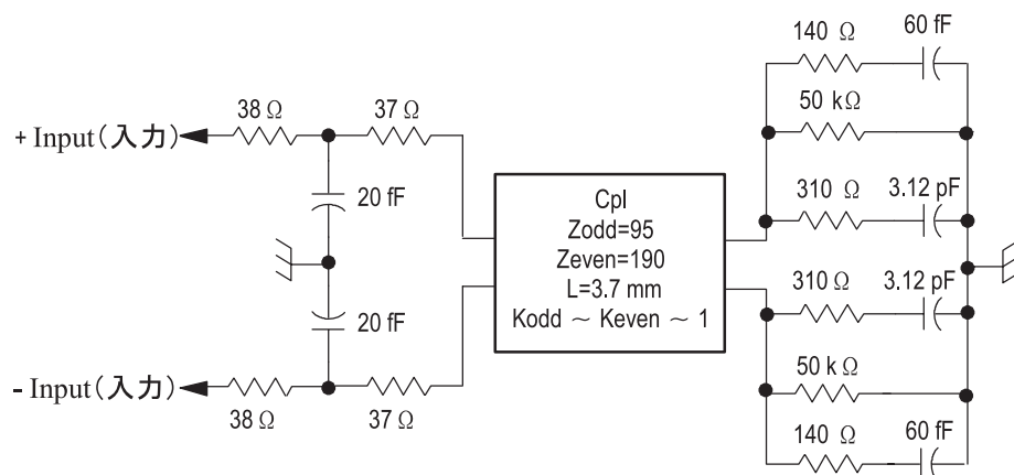
図 3 : 代表的なプローブ入力のモデル
