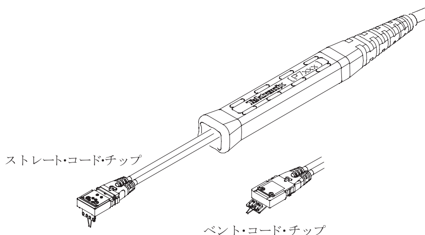
図 2： HBW ストレート・コード、8 ミルワイヤの Tip-Clip アセンブリ
