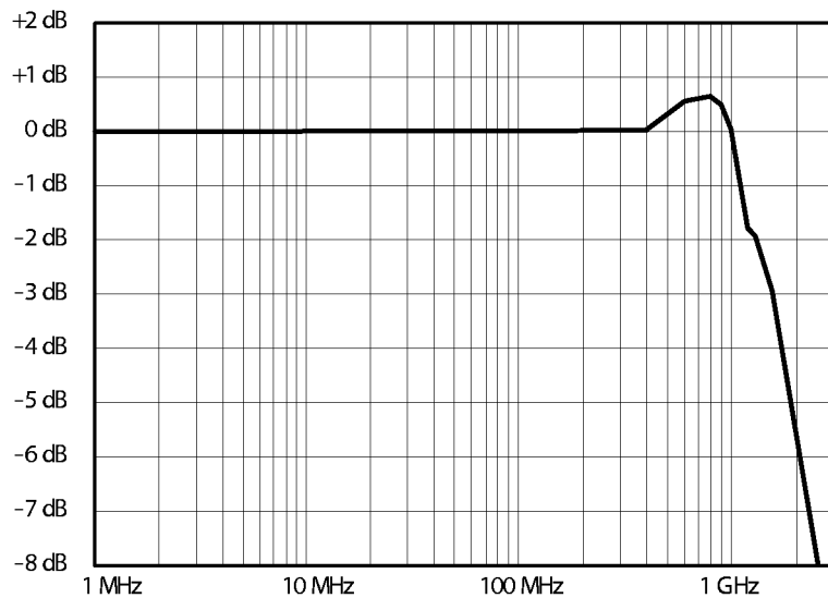
图 2: 典型带宽
