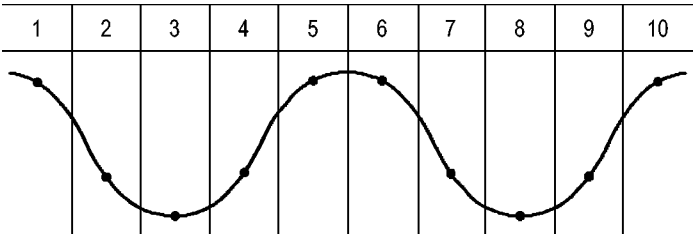
取樣擷取間隔 (2,500)
