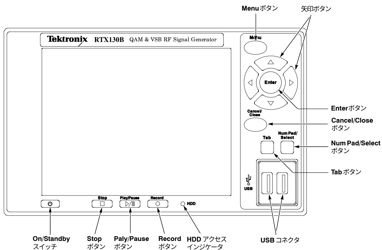
図 2-1：フロント・パネル
