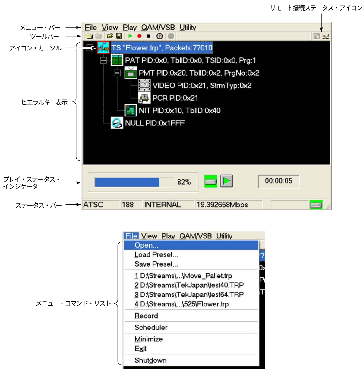
図 2-3 : Play スクリーンでの表示項目
