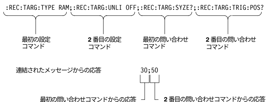
図 3-30：設定コマンドおよび問い合わせコマンドの連結
