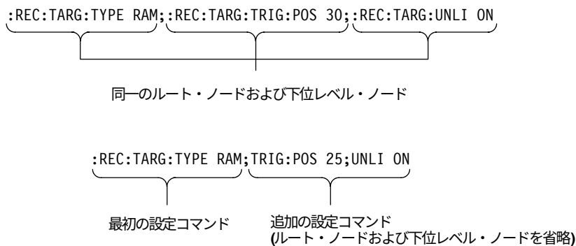
図 3-31：連結されたメッセージ内でのルート・ノードと下位レベル・ノードの省略
