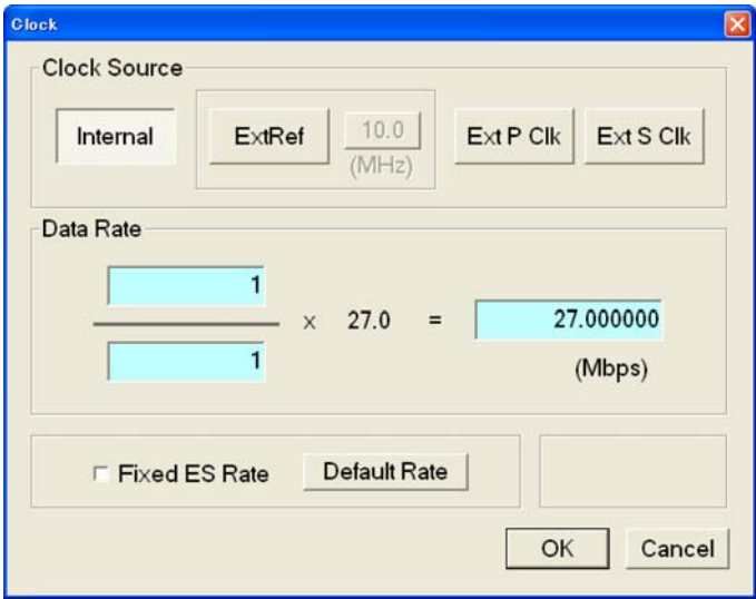
図 3-2 : Clock ダイアログ・ボックス
