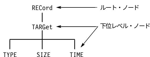
図 3-28 : SCPI サブシステムのツリー構造
