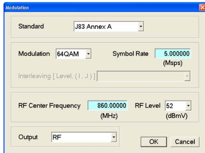
図 3-8 : Modulation ダイアログ・ボックス
