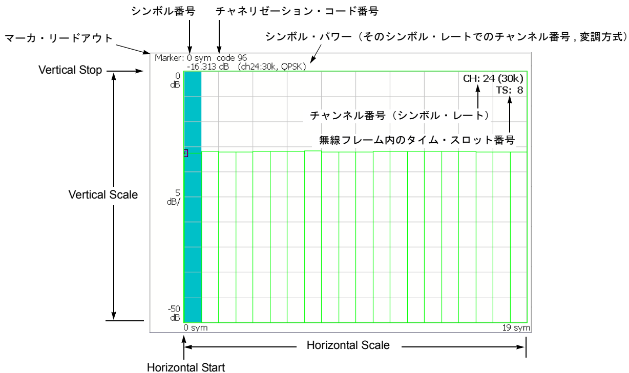
図 2-7 : コード・ドメイン・パワー vs. シンボル
