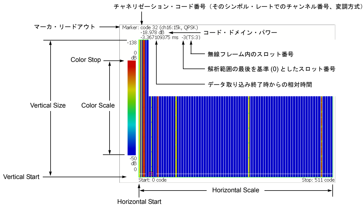
図 2-5 : パワー・コードグラム
