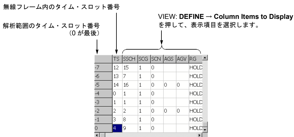
図 2-3 : タイム・スロット・テーブル (画面左下)
