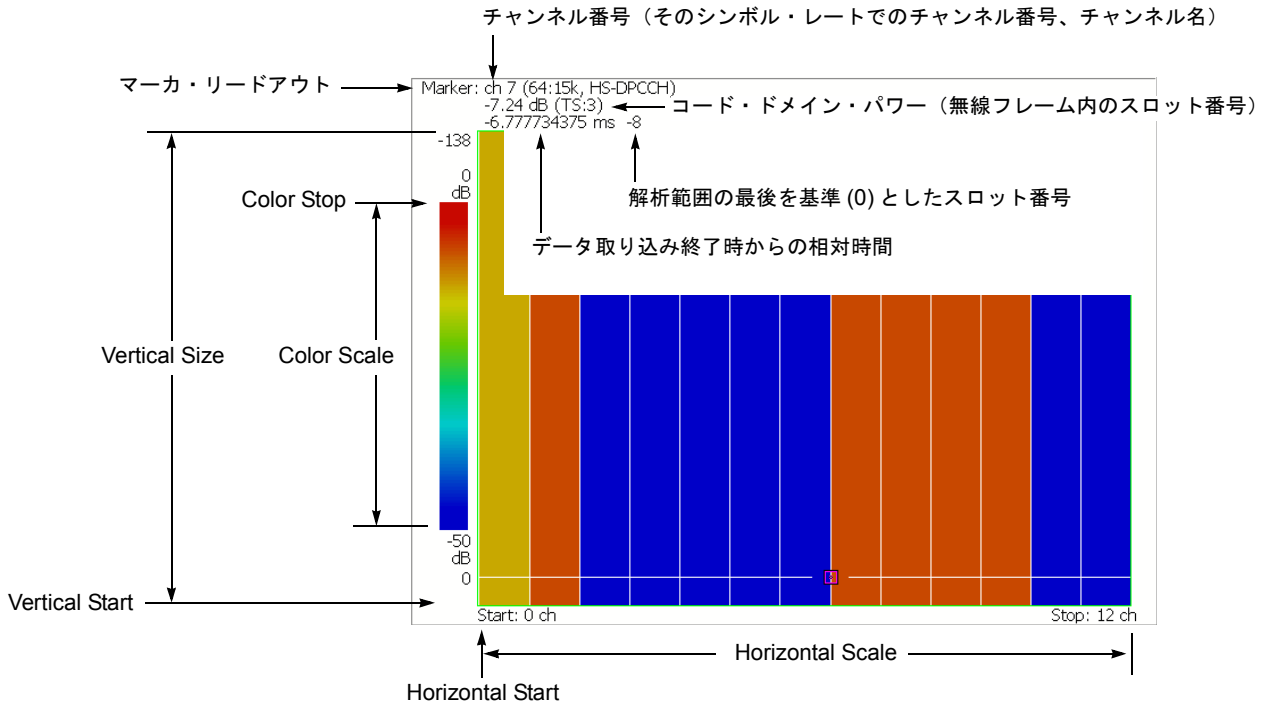
図 2-23 : パワー・コードグラム
