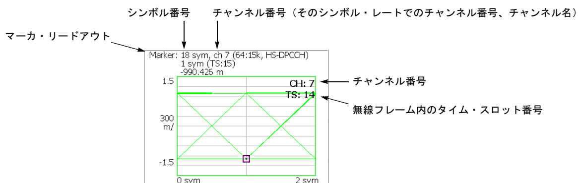
図 2-28 : シンボル・アイ・ダイアグラム
