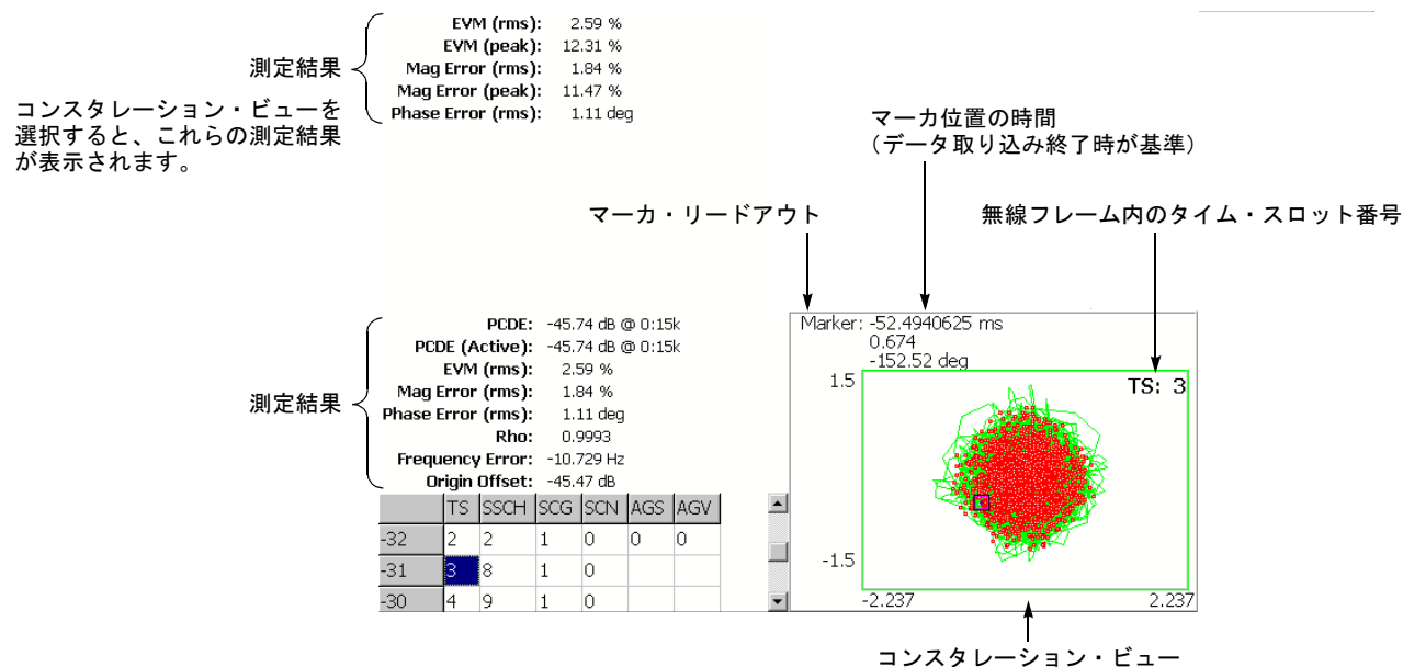
図 2-12 : 変調確度
