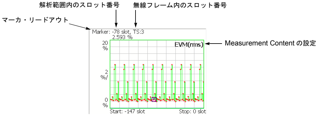
図 2-13 : 変調精度 vs タイム・スロット、EVM (rms)
