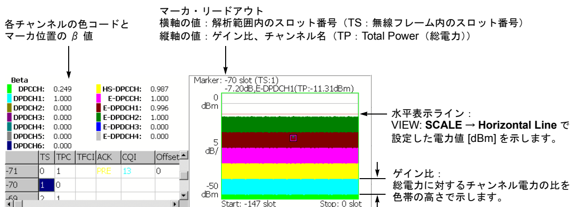
図 2-32 : ゲイン比
