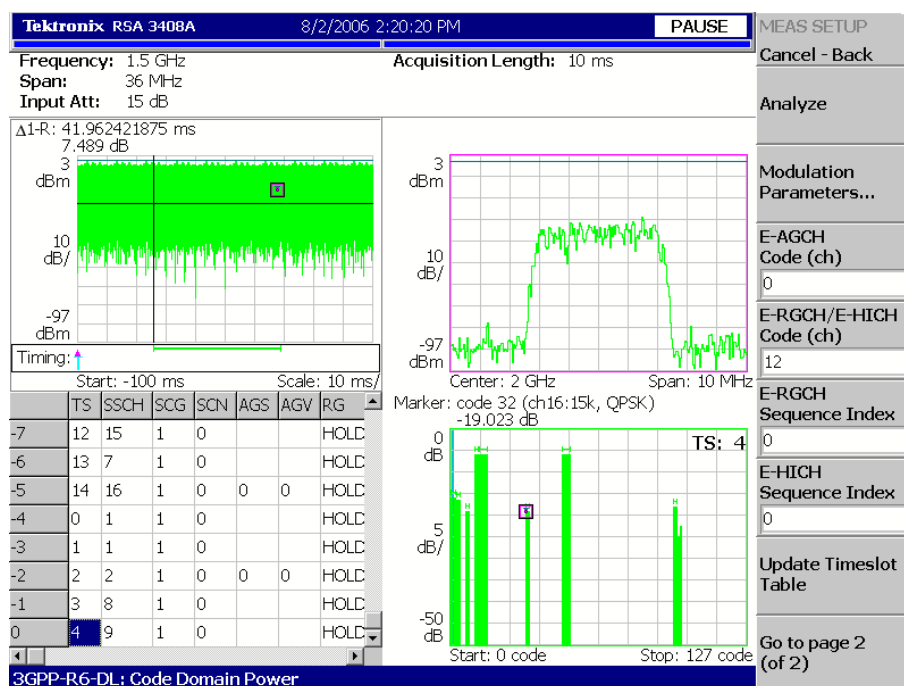
図 2-2 : コード・ドメイン・パワー測定例
