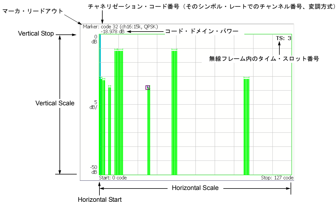
図 2-4 : コード・ドメイン・パワー
