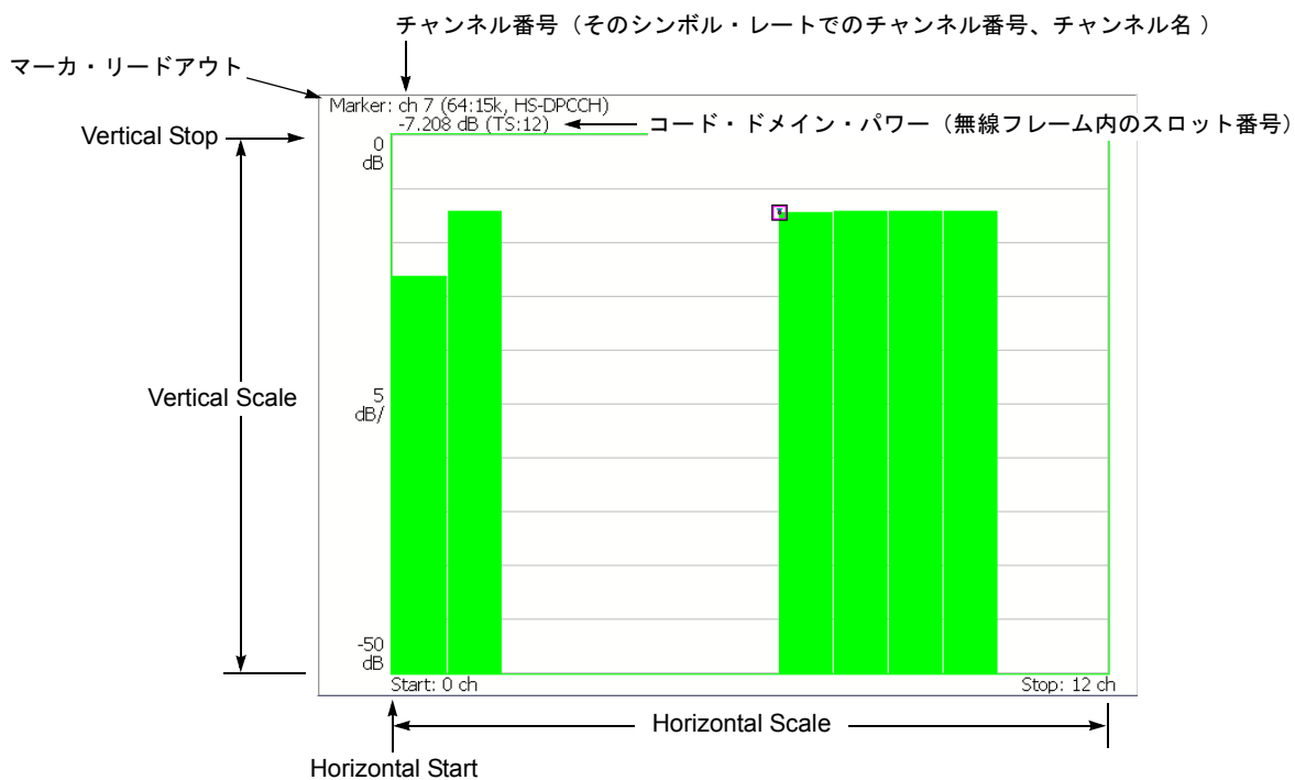
図 2-22 : コード・ドメイン・パワー
