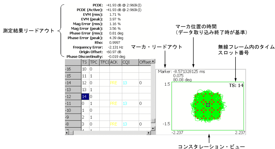
図 2-30 : 変調確度
