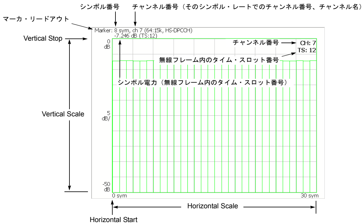
図 2-25 : コード・ドメイン・パワー vs. シンボル
