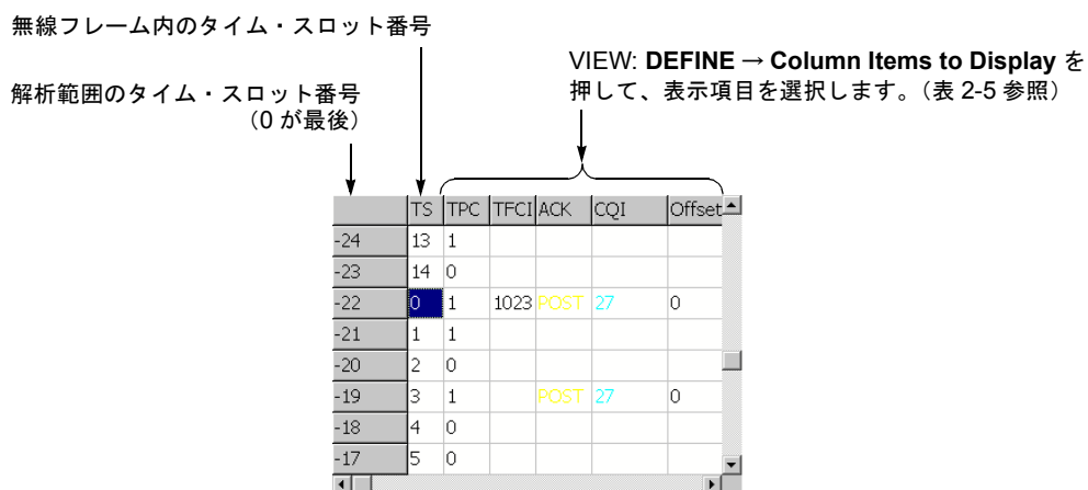
図 2-21 : タイム・スロット・テーブル
