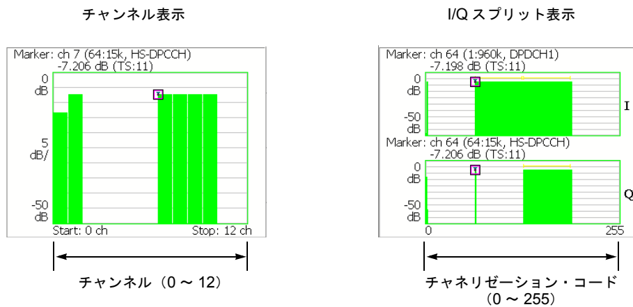
図 2-20 : View Format 設定 (コード・ドメイン・パワー測定)
