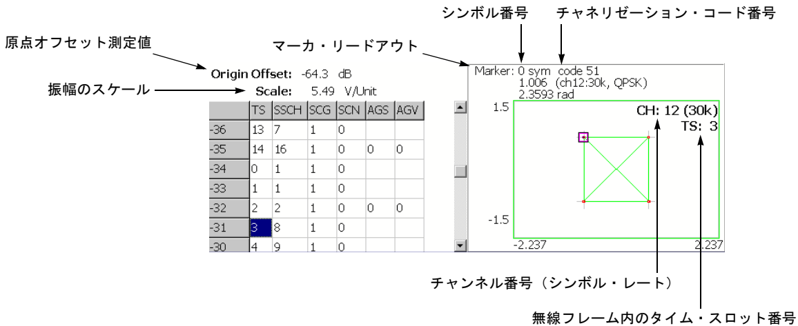
図 2-8 : シンボル・コンスタレーション
