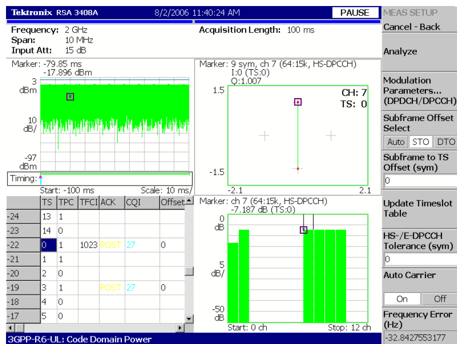
図 2-15 : コード・ドメイン・パワー測定例
