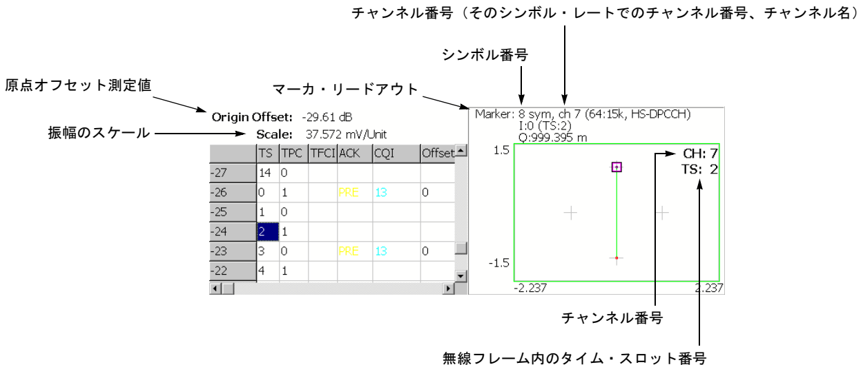
図 2-26 : シンボル・コンスタレーション
