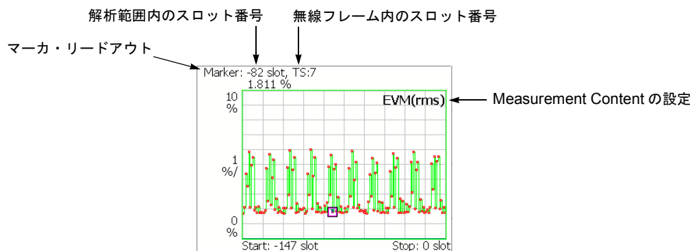
図 2-31 : 変調確度 vs タイム・スロット、EVM (rms)
