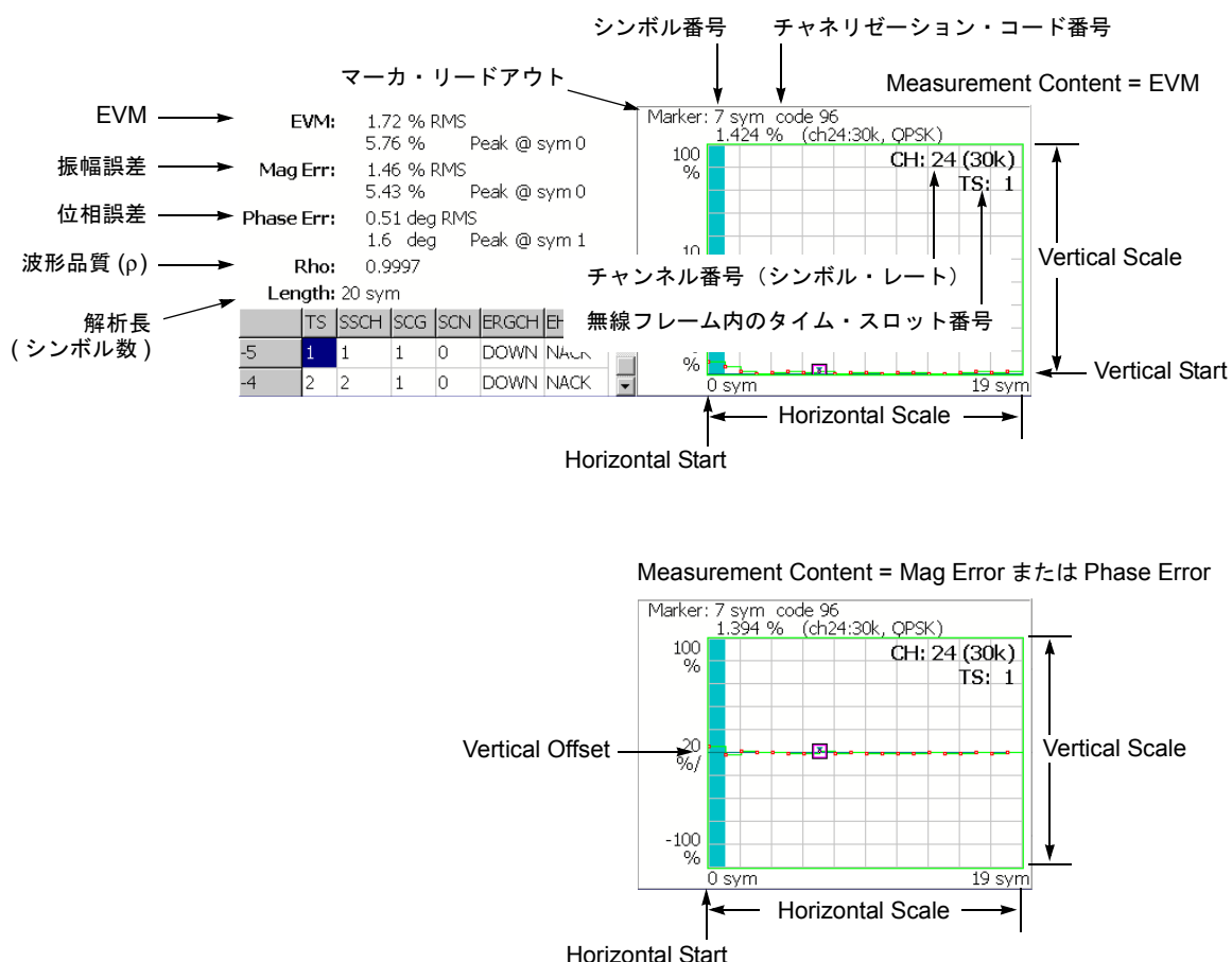
図 2-9 : シンボル EVM
