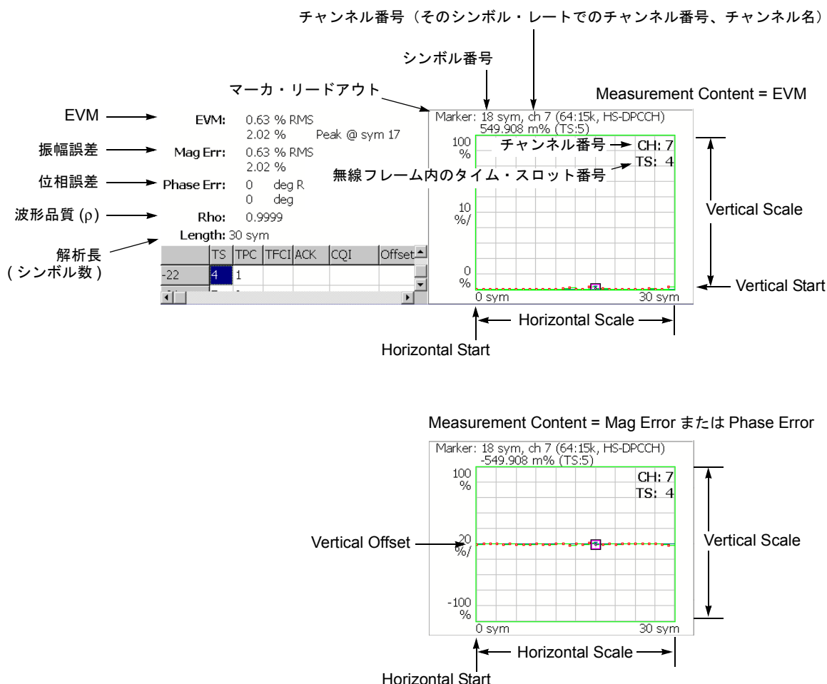
図 2-27 : シンボル EVM
