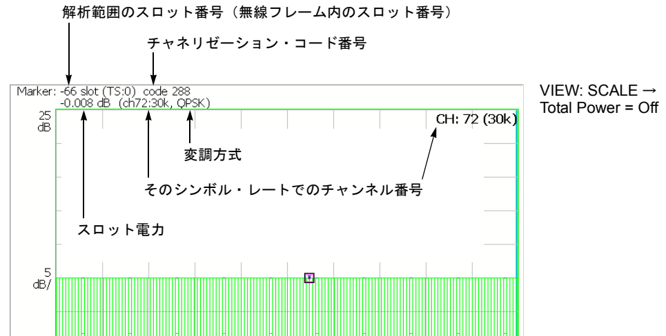
図 2-6 : コード・ドメイン・パワー vs. タイム・スロット
