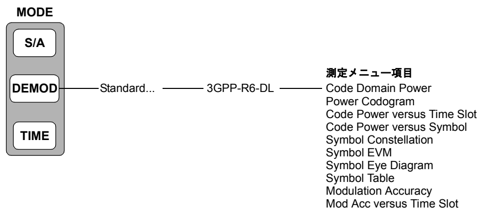
図 2-1 : ダウンリンク解析測定メニュー
