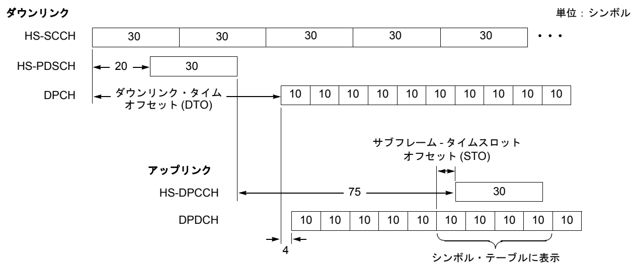
図 2-16 : サブフレーム・オフセット
