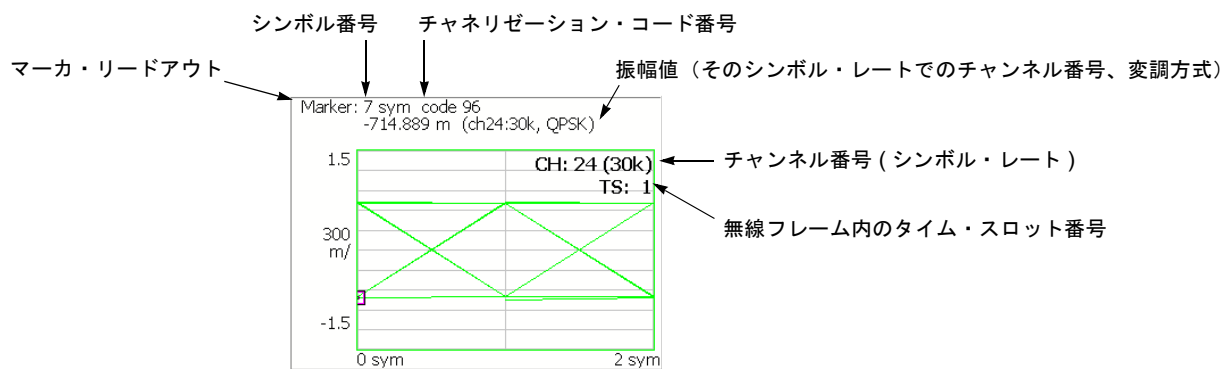
図 2-10 : シンボル・アイ・ダイアグラム
