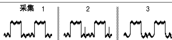
包络在每个单采集采用峰值探测模式。
